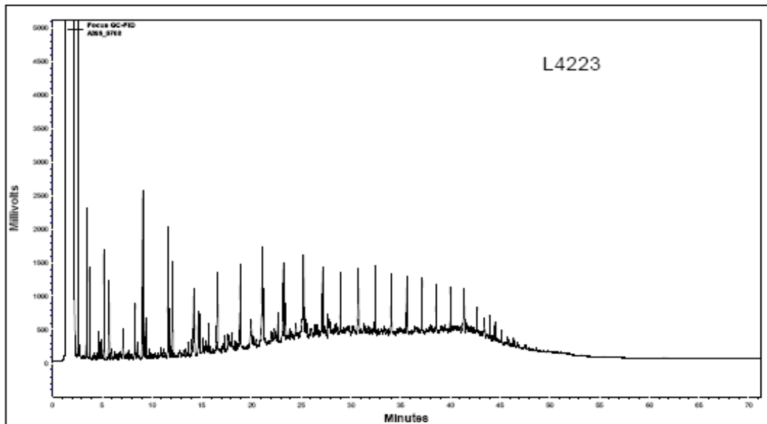
FIGURA 1: Cromatograma da análise de TPH da amostra de água produzida PNA 1 FLOTADOR B
