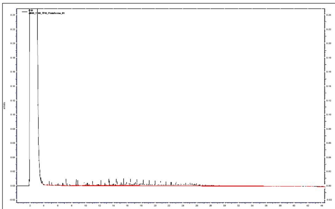
FIGURA 2: Cromatograma da análise de TPH da amostra de água produzida PNA 1 FLOTADOR B
