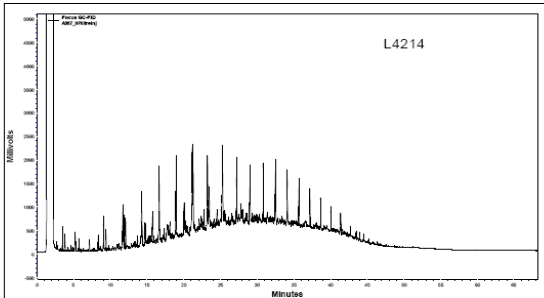
FIGURA 1: Cromatograma da análise de TPH da amostra de água produzida PGP 1 SA1201 B
