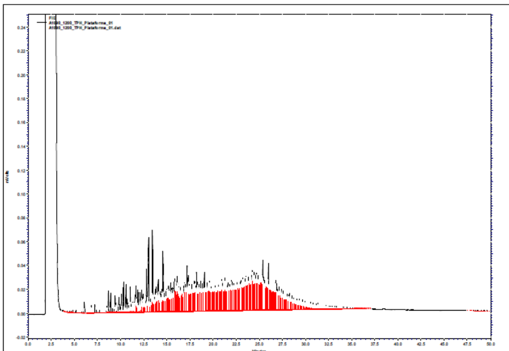
FIGURA 2: Cromatograma da análise de TPH da amostra de água produzida P 33
