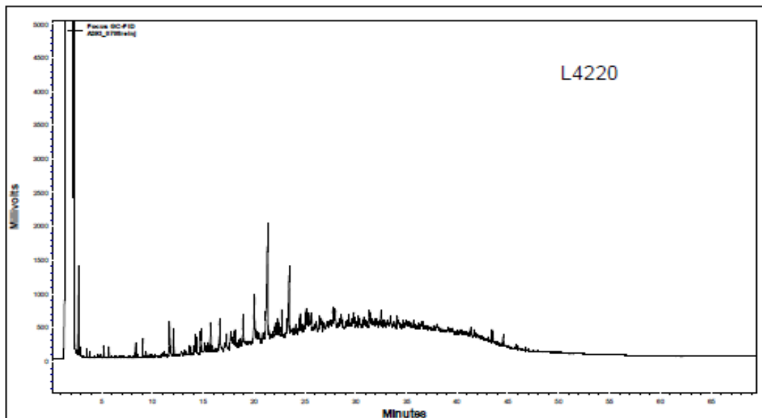
FIGURA 1: Cromatograma da análise de TPH da amostra de água produzida P 33
