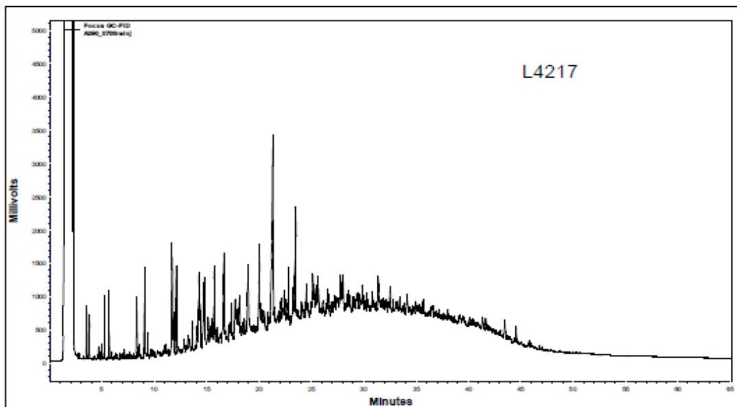
FIGURA 1: Cromatograma da análise de TPH da amostra de água produzida P 26
