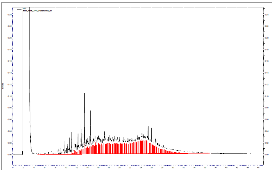
FIGURA 2: Cromatograma da análise de TPH da amostra de água produzida P 26
