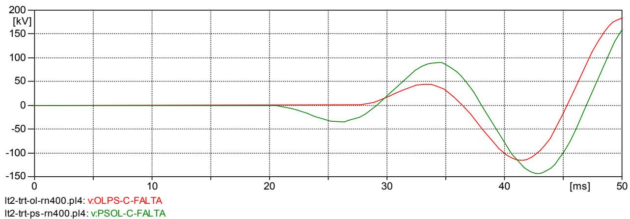
Figura 6.8 – Análise da TRT Associada à Extinção da Corrente de Arco Secundário, Com reator de neutro de 400 Ω
