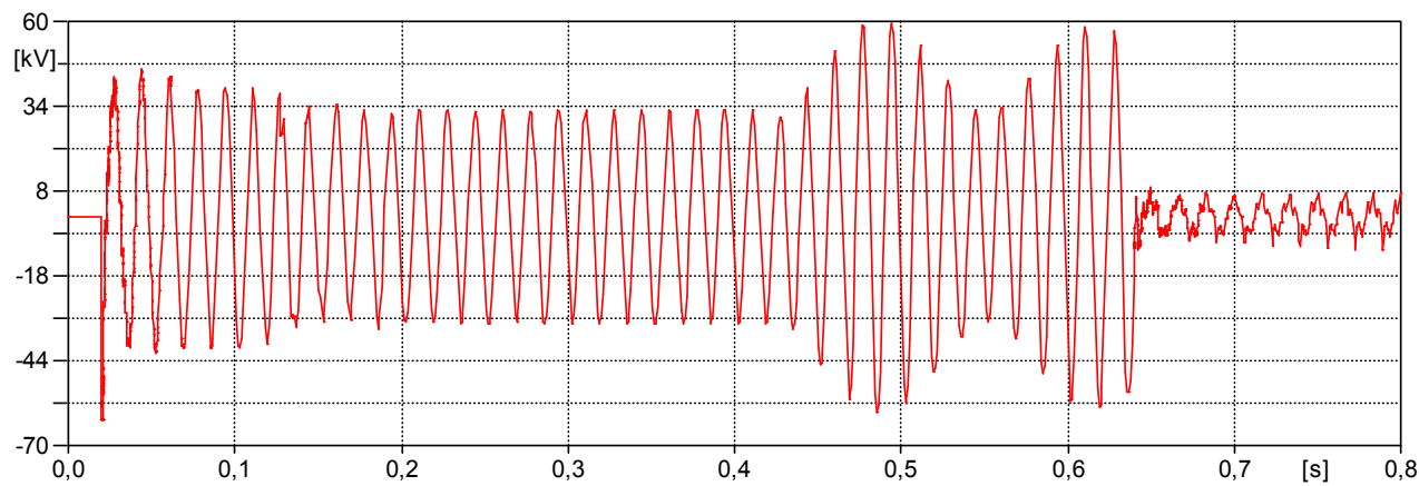
Figura 6.15 – Análise Transitória - Caso com pior Tensão no Neutro – Sem RPI – Religamento Monopolar através do terminal de P. Sergipe, com falta no terminal de P. Sergipe
