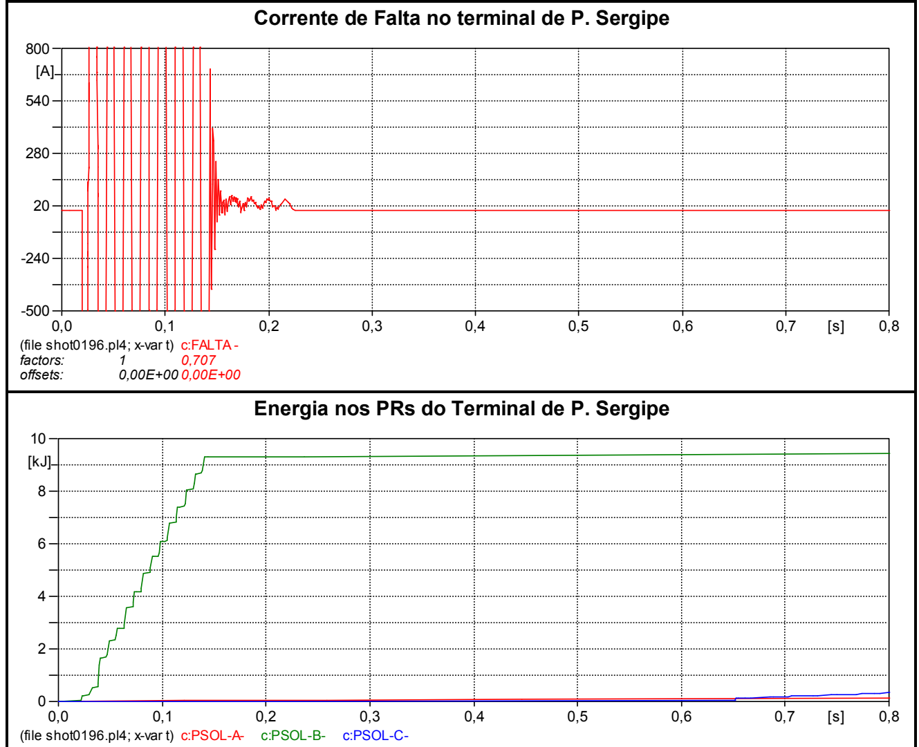
Figura 6.16 – Análise Transitória - Caso com pior sobretensão na LT – Com RPI – Religamento Monopolar através do terminal de Olindina, com falta no terminal de P. Sergipe
