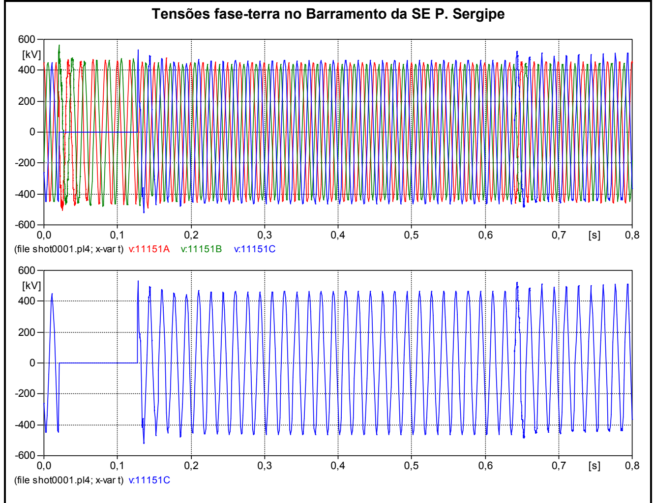
Figura 6.15 – Análise Transitória - Caso com pior Tensão no Neutro – Sem RPI – Religamento Monopolar através do terminal de P. Sergipe, com falta no terminal de P. Sergipe
