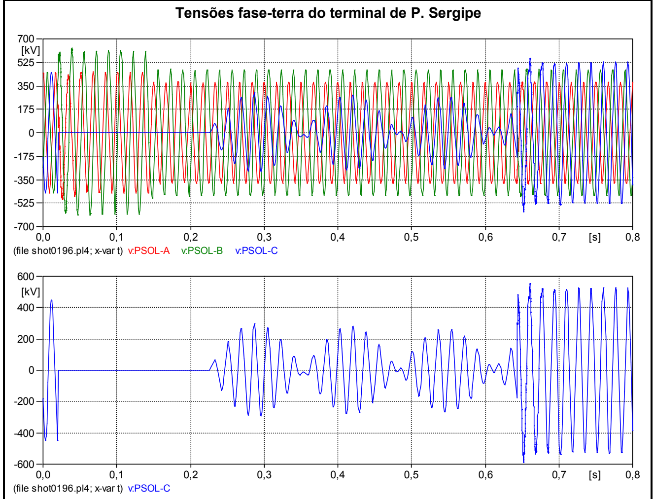
Figura 6.16 – Análise Transitória - Caso com pior sobretensão na LT – Com RPI – Religamento Monopolar através do terminal de Olindina, com falta no terminal de P. Sergipe
