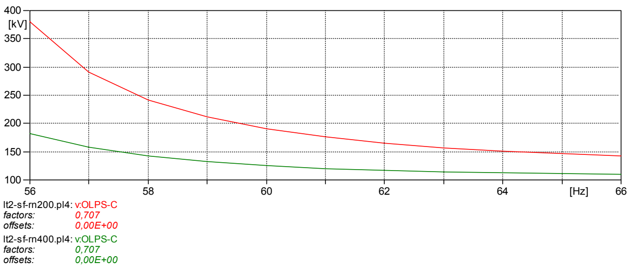
Figura 6.4 – Análise em Regime Permanente no Domínio da Frequência, Sem falta – Com reatores de neutro de 200 \Omega e 400 \Omega - Tensão induzida na fase aberta ( V_{rms} ) no Terminal de Olindina
