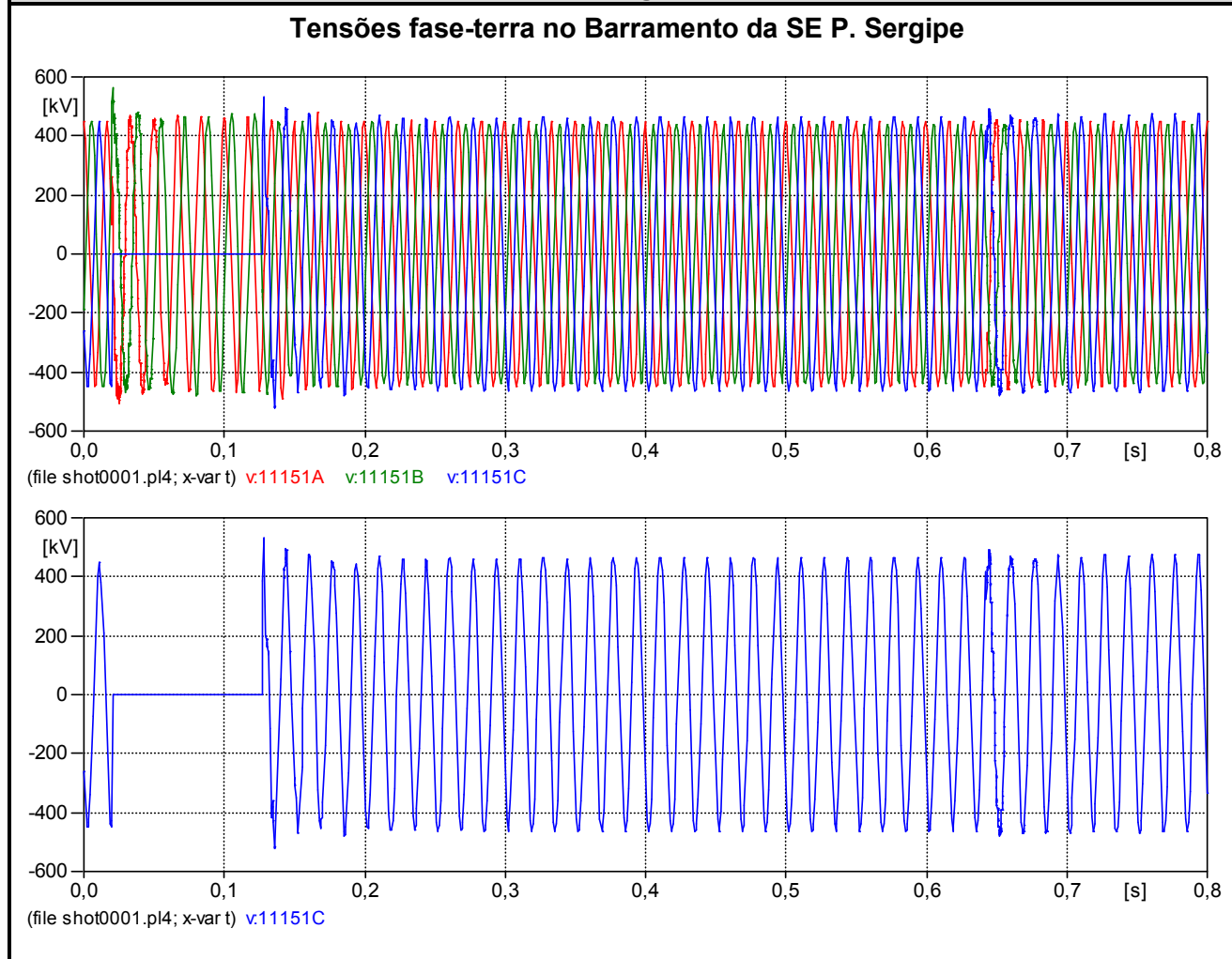
Figura 6.17 – Análise Transitória - Caso com pior Tensão no Neutro – Sem RPI – Religamento Monopolar através do terminal de P. Sergipe, com falta no terminal de P. Sergipe
