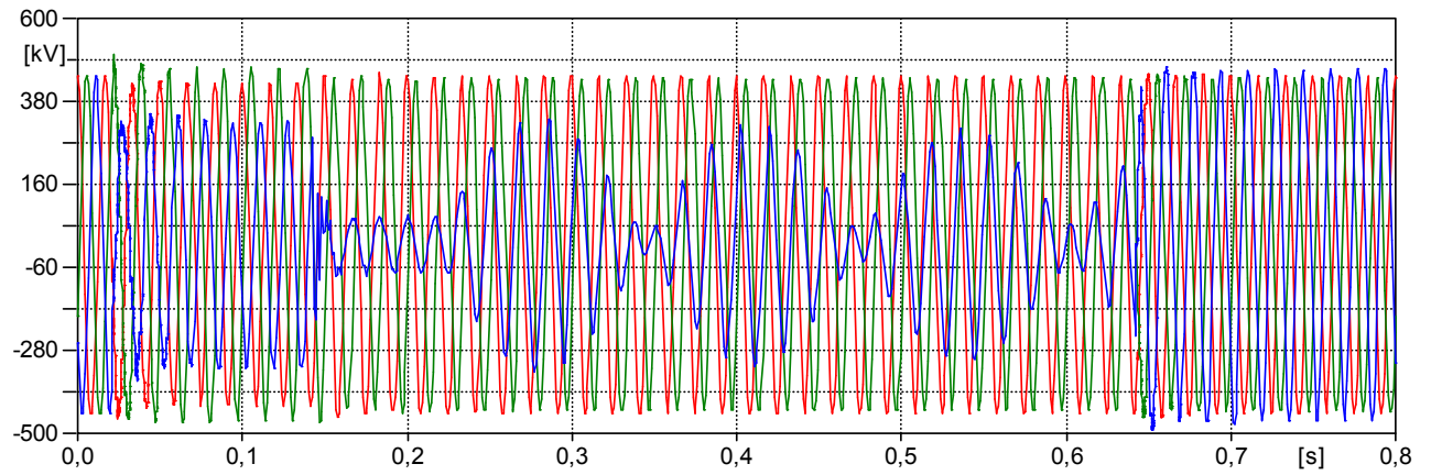
Figura 6.16 – Análise Transitória - Caso com pior sobretensão na LT – Com RPI – Religamento Monopolar através do terminal de Olindina, com falta no terminal de P. Sergipe
