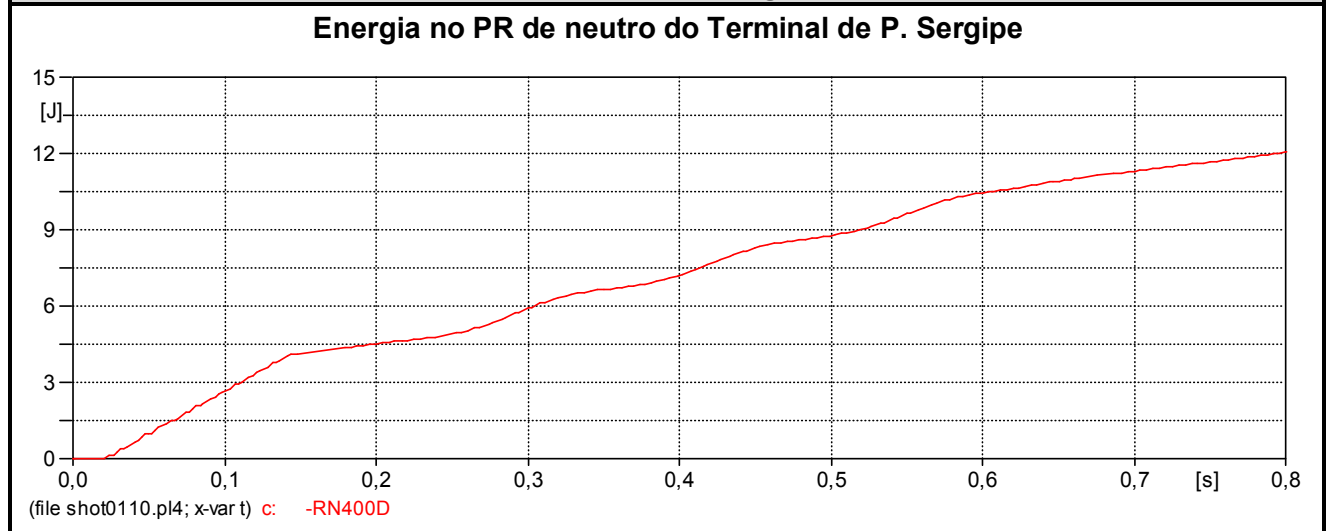
Figura 6.14 – Análise Transitória - Caso com pior sobretensão na LT e Pior Energia nos PRs de Linha – Sem RPI – Religamento Monopolar através do terminal de Olindina, com falta no terminal de P. Sergipe
