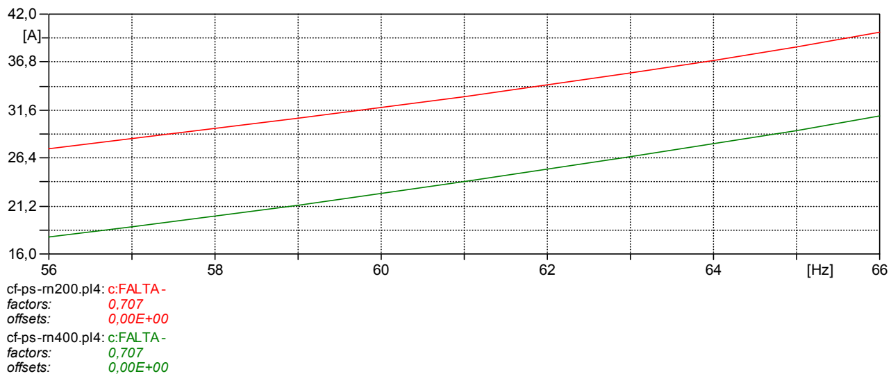
Figura 6.7 – Análise em Regime Permanente no Domínio da Frequência, Com falta – Com reatores de neutro de 200 Ω e 400 Ω - Corrente de arco secundário ( A_{rms} ) no Terminal de P. Sergipe
