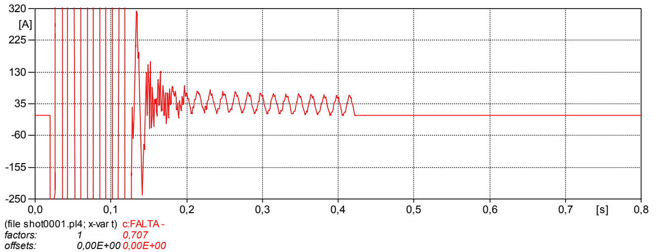
Figura 6.15 – Análise Transitória - Caso com pior Tensão no Neutro – Sem RPI – Religamento Monopolar através do terminal de P. Sergipe, com falta no terminal de P. Sergipe
