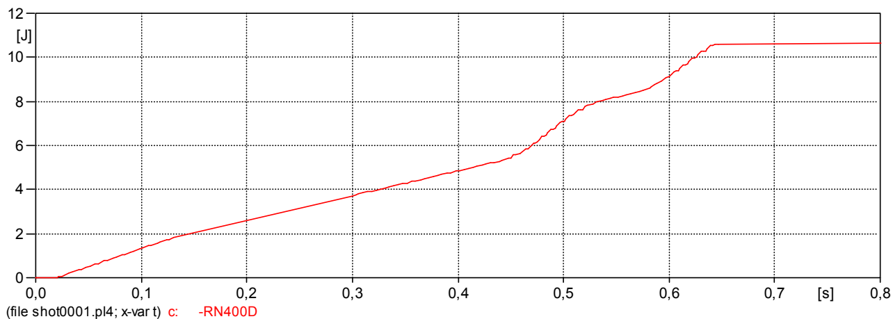
Figura 6.17 – Análise Transitória - Caso com pior Tensão no Neutro – Sem RPI – Religamento Monopolar através do terminal de P. Sergipe, com falta no terminal de P. Sergipe
