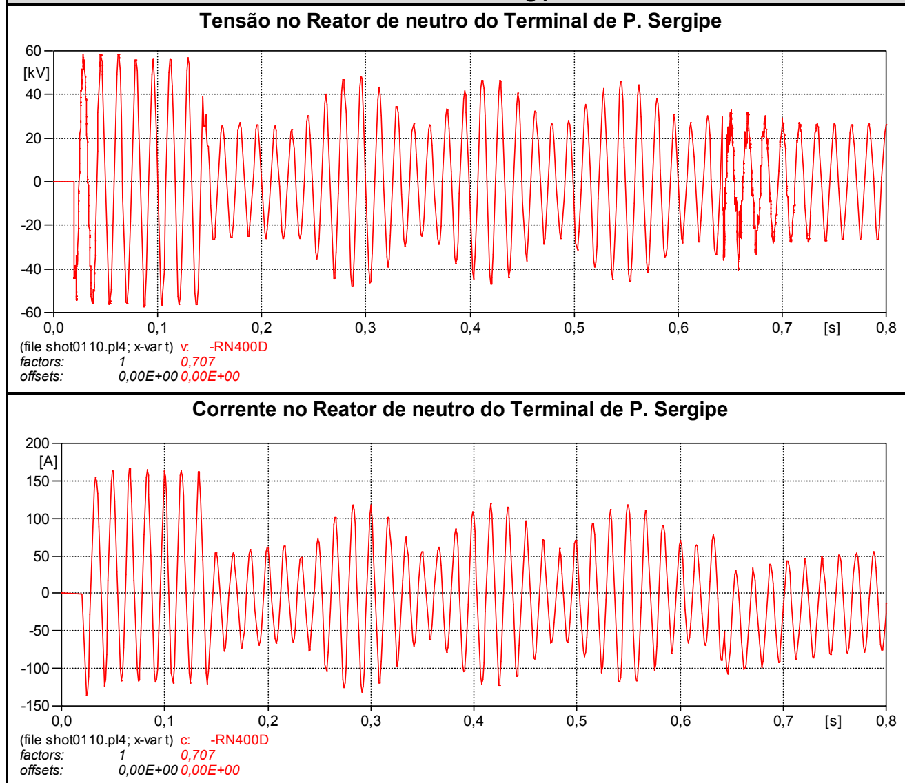
Figura 6.14 – Análise Transitória - Caso com pior sobretensão na LT e Pior Energia nos PRs de Linha – Sem RPI – Religamento Monopolar através do terminal de Olindina, com falta no terminal de P. Sergipe
