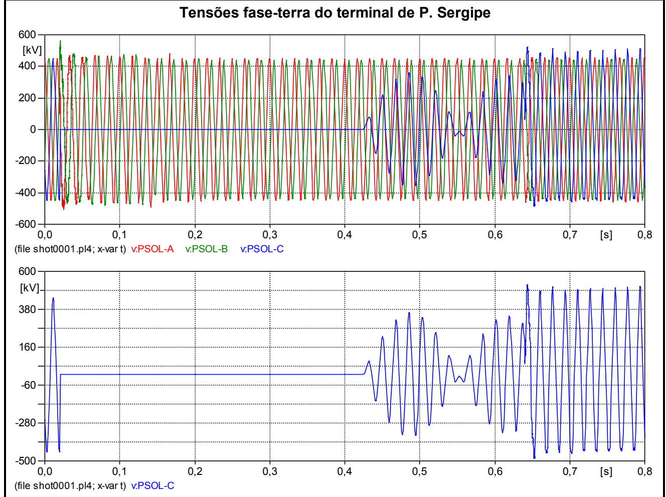
Figura 6.15 – Análise Transitória - Caso com pior Tensão no Neutro – Sem RPI – Religamento Monopolar através do terminal de P. Sergipe, com falta no terminal de P. Sergipe
