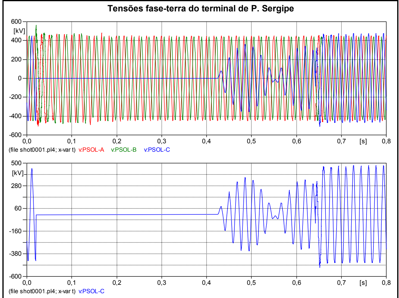
Figura 6.17 – Análise Transitória - Caso com pior Tensão no Neutro – Sem RPI – Religamento Monopolar através do terminal de P. Sergipe, com falta no terminal de P. Sergipe
