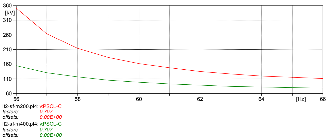
Figura 6.5 – Análise em Regime Permanente no Domínio da Frequência, Sem falta – Com reatores de neutro de 200 Ω e 400 Ω - Tensão induzida na fase aberta ( V_{rms} ) no Terminal de P. Sergipe
