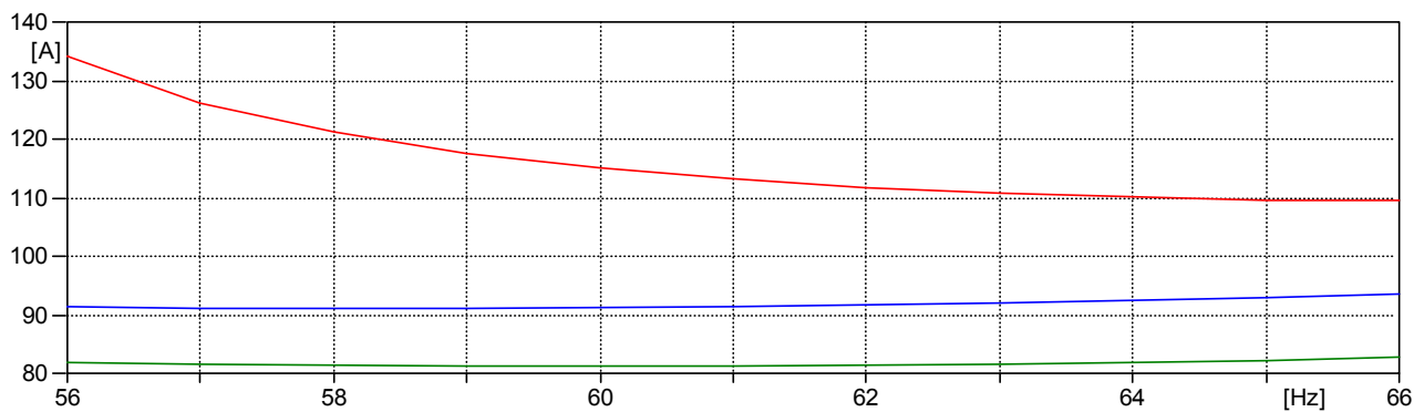
Figura 6.12 – Análise em Regime Permanente no Domínio da Frequência – Com reator de neutro de 400 Ω - Corrente no reator de neutro ( A_{rms} ) no Terminal de Olindina
