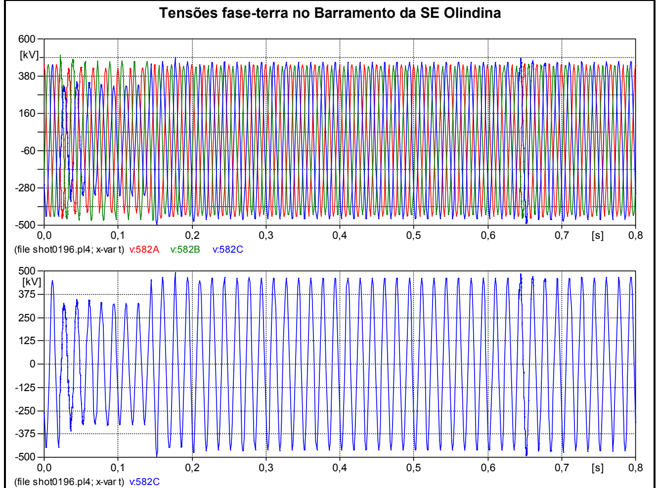
Figura 6.16 – Análise Transitória - Caso com pior sobretensão na LT – Com RPI – Religamento Monopolar através do terminal de Olindina, com falta no terminal de P. Sergipe
