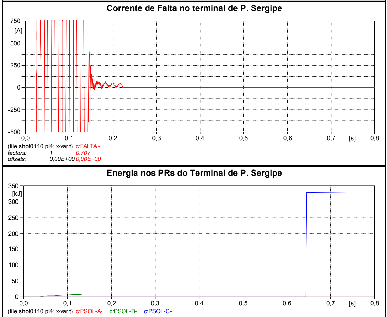
Figura 6.14 – Análise Transitória - Caso com pior sobretensão na LT e Pior Energia nos PRs de Linha – Sem RPI – Religamento Monopolar através do terminal de Olindina, com falta no terminal de P. Sergipe
