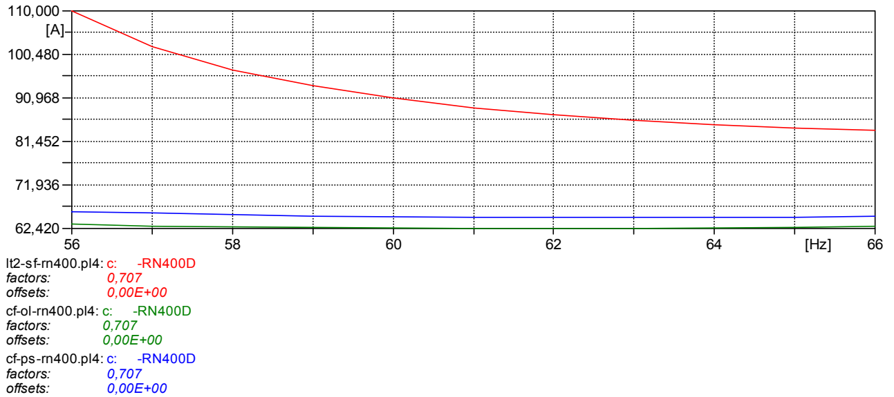
Figura 6.13 – Análise em Regime Permanente no Domínio da Frequência – Com reator de neutro de 400 Ω - Corrente no reator de neutro ( A_{rms} ) no Terminal de Porto Sergipe
