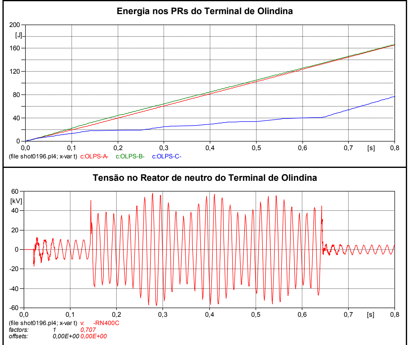
Figura 6.16 – Análise Transitória - Caso com pior sobretensão na LT – Com RPI – Religamento Monopolar através do terminal de Olindina, com falta no terminal de P. Sergipe
