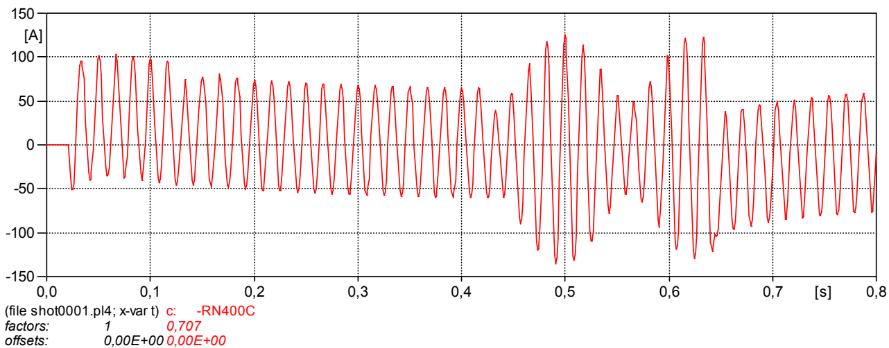
Figura 6.17 – Análise Transitória - Caso com pior Tensão no Neutro – Sem RPI – Religamento Monopolar através do terminal de P. Sergipe, com falta no terminal de P. Sergipe
