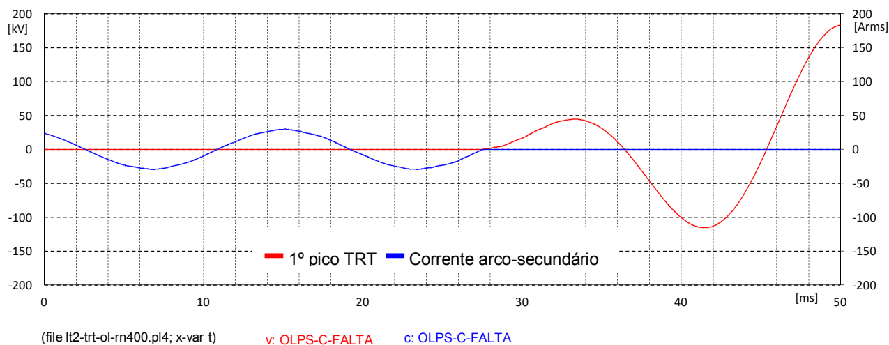
Figura 6.9 – Corrente de arco secundário x Primeiro pico da TRT – Com reator de neutro de 400 Ω
