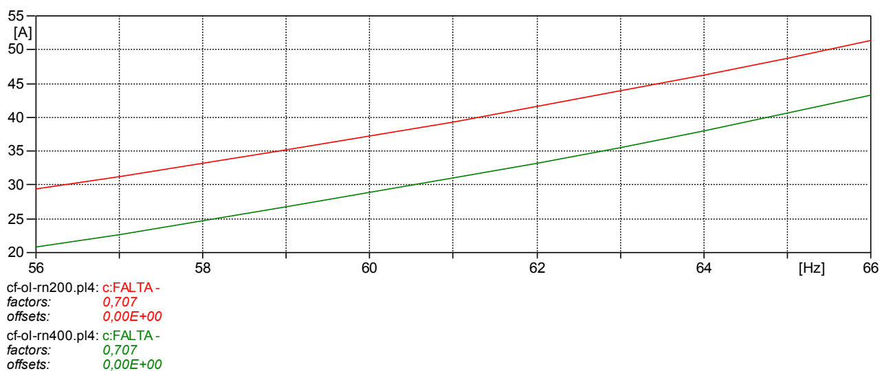
Figura 6.6 – Análise em Regime Permanente no Domínio da Frequência, Com falta – Com reatores de neutro de 200 Ω e 400 Ω - Corrente de arco secundário ( A_{rms} ) Terminal de Olindina
