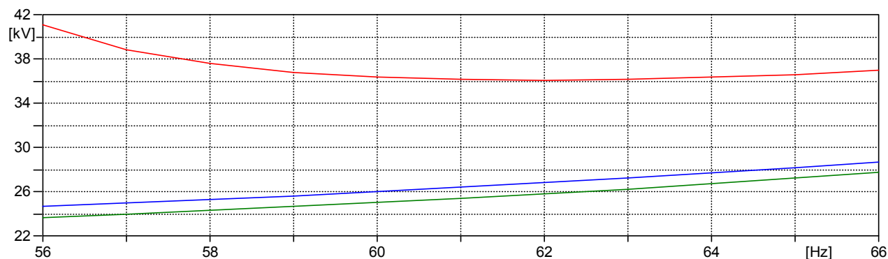
Figura 6.11 – Análise em Regime Permanente no Domínio da Frequência – Com reator de neutro de 400 Ω - Tensão no reator de neutro ( kV_{rms} ) no Terminal de Porto Sergipe
