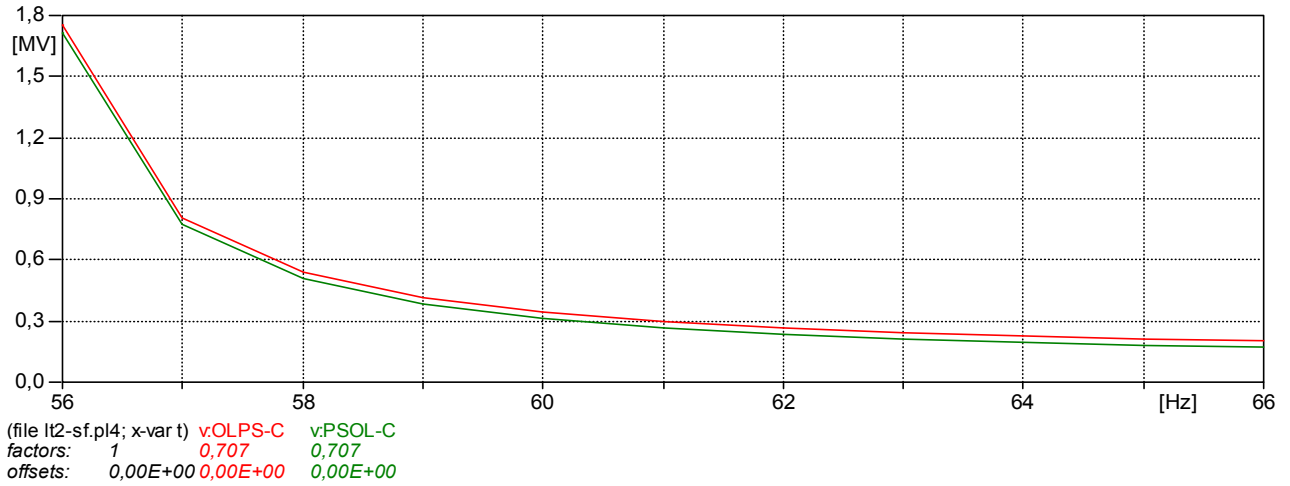
Figura 6.1 – Análise em Regime Permanente no Domínio da Frequência, Sem falta, Sem reator de neutro - Tensão induzida na fase aberta ( V_{rms} )
