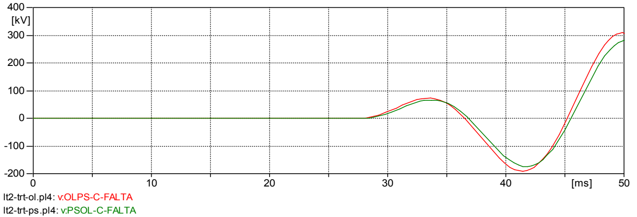
Figura 6.3 – Análise da TRT Associada à Extinção da Corrente de Arco Secundário, Sem reator de neutro - TRT após a extinção do arco secundário
