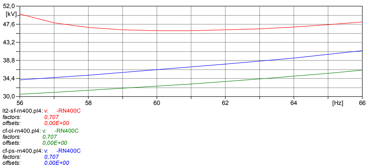
Figura 6.10 – Análise em Regime Permanente no Domínio da Frequência – Com reator de neutro de 400 Ω - Tensão no reator de neutro ( kV_{rms} ) no Terminal de Olindina
