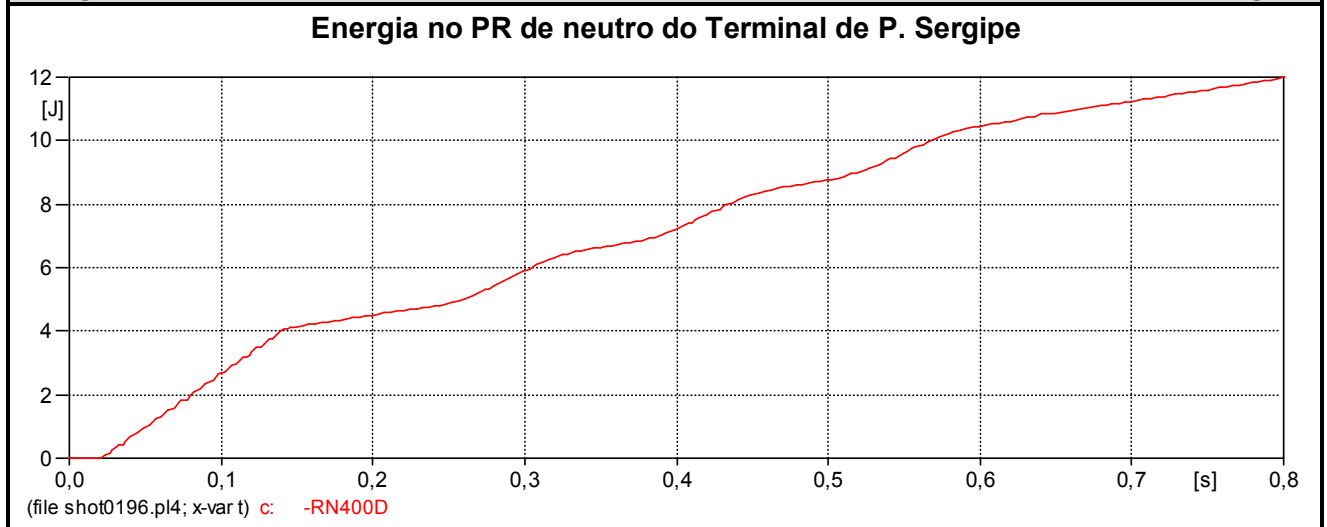
Figura 6.16 – Análise Transitória - Caso com pior sobretensão na LT – Com RPI – Religamento Monopolar através do terminal de Olindina, com falta no terminal de P. Sergipe
