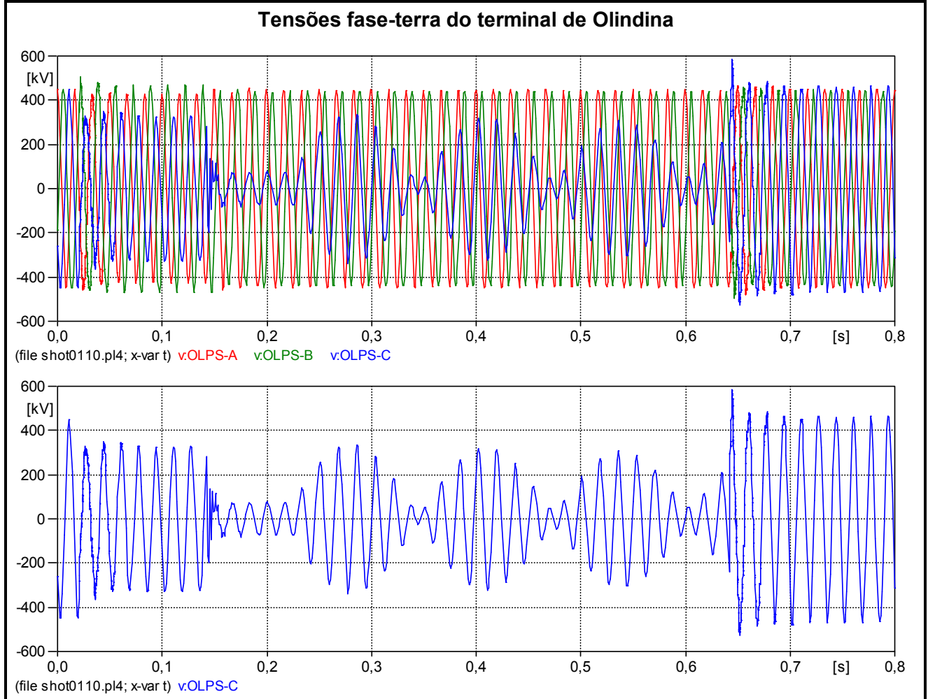
Figura 6.14 – Análise Transitória - Caso com pior sobretensão na LT e Pior Energia nos PRs de Linha – Sem RPI – Religamento Monopolar através do terminal de Olindina, com falta no terminal de P. Sergipe
