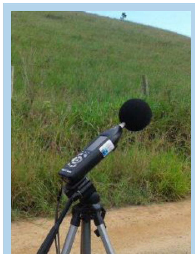
Equipamento de medição de ruídos
