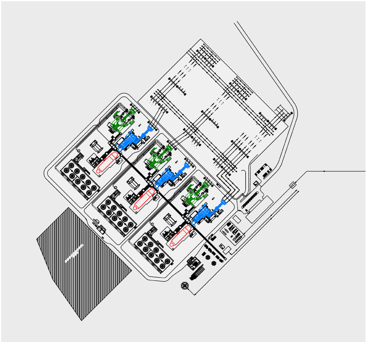
Figura 2 - Arranjo da UTE Nossa Senhora de Fátima
