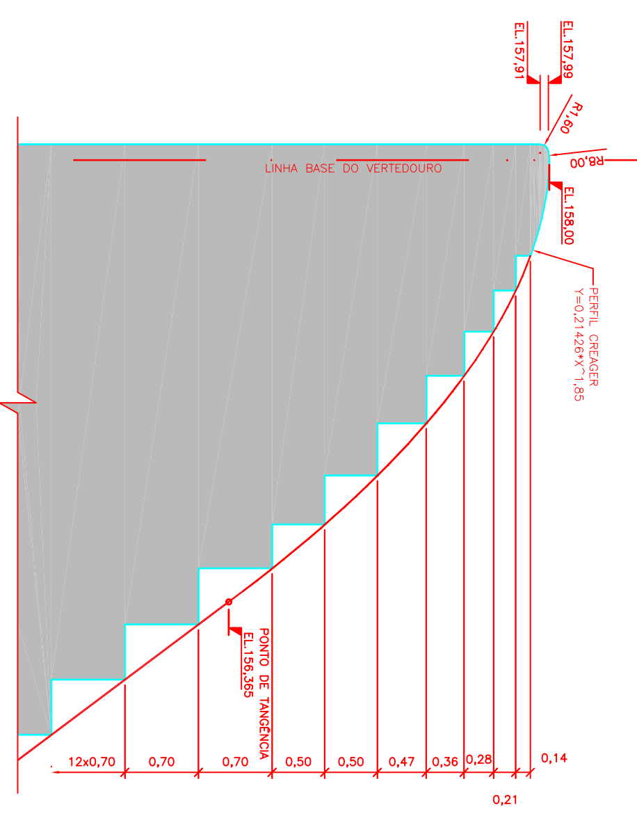
DETALHE 01 ESC: 1:50
