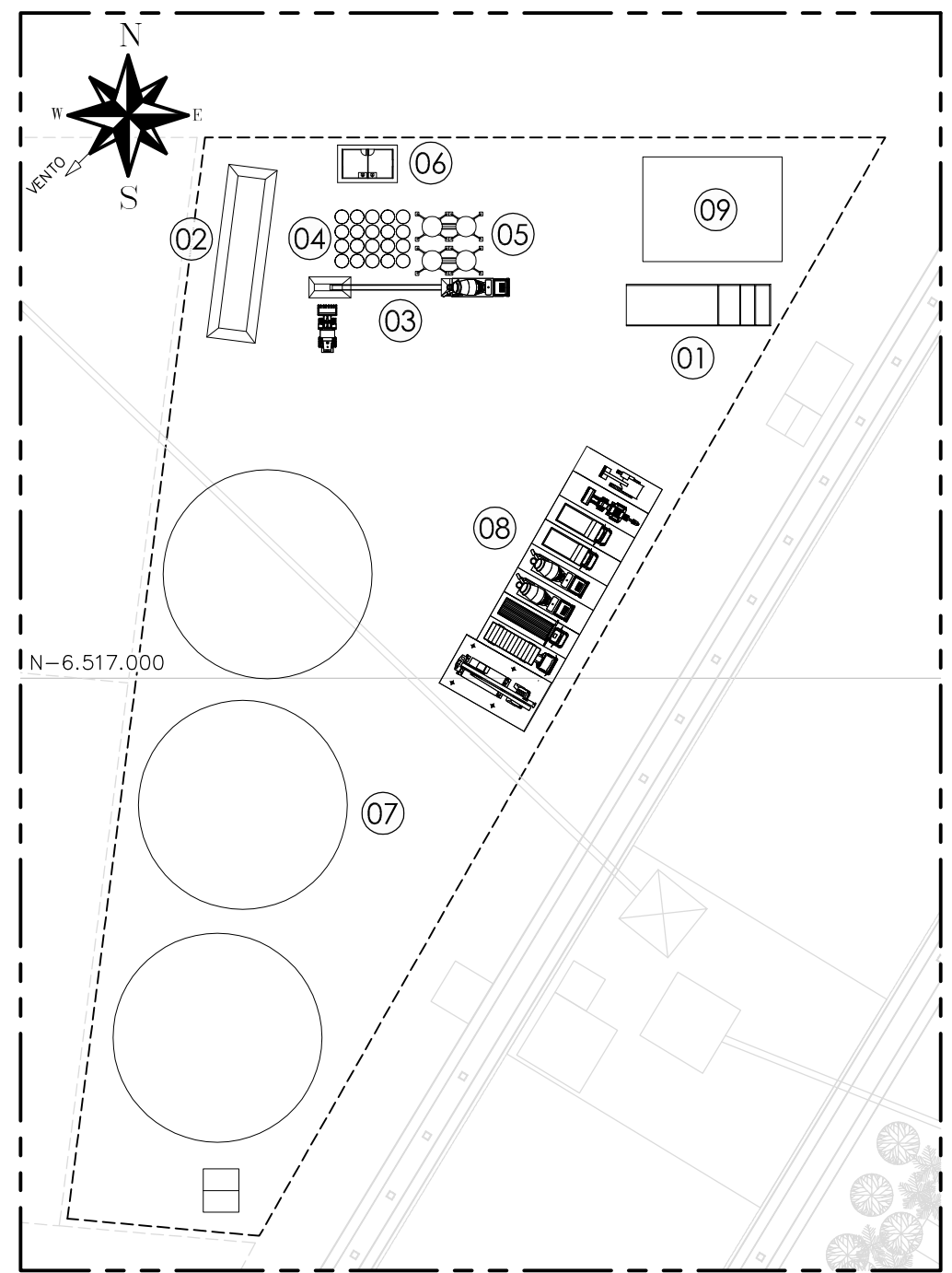
CANTEIRO INDUSTRIAL UTE PAMPA SUL ESC. 1:1.000
