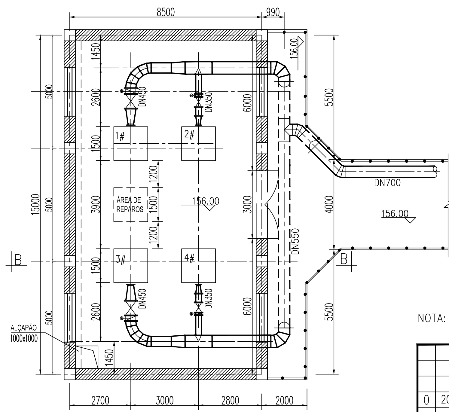
PLANTA DA CASA DE BOMBAS DA TOMADA DE ÁGUA
