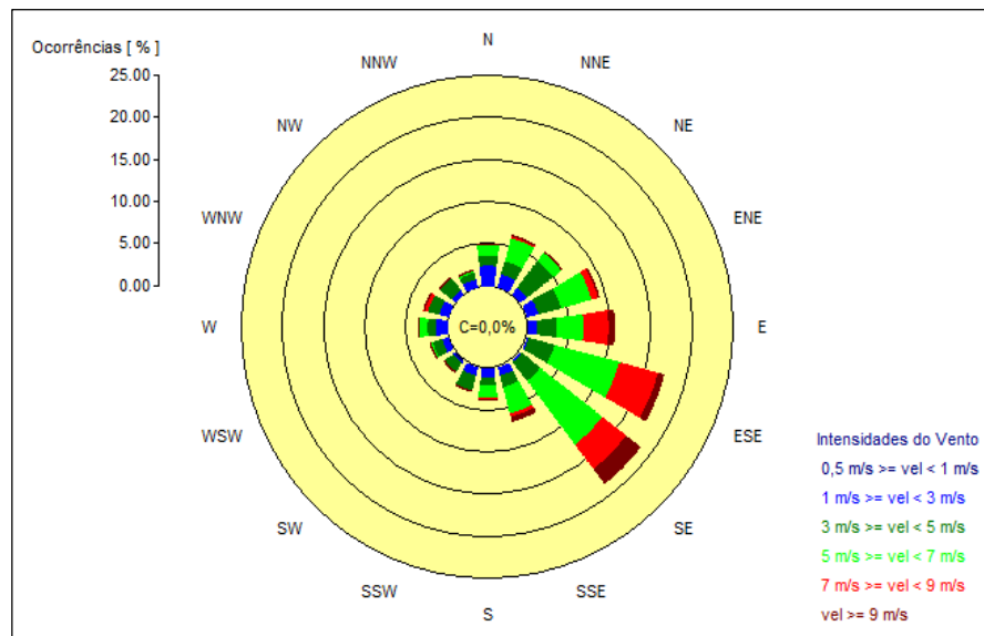
Figura 19 – Rosa dos Ventos – Estação Pedras Altas.
