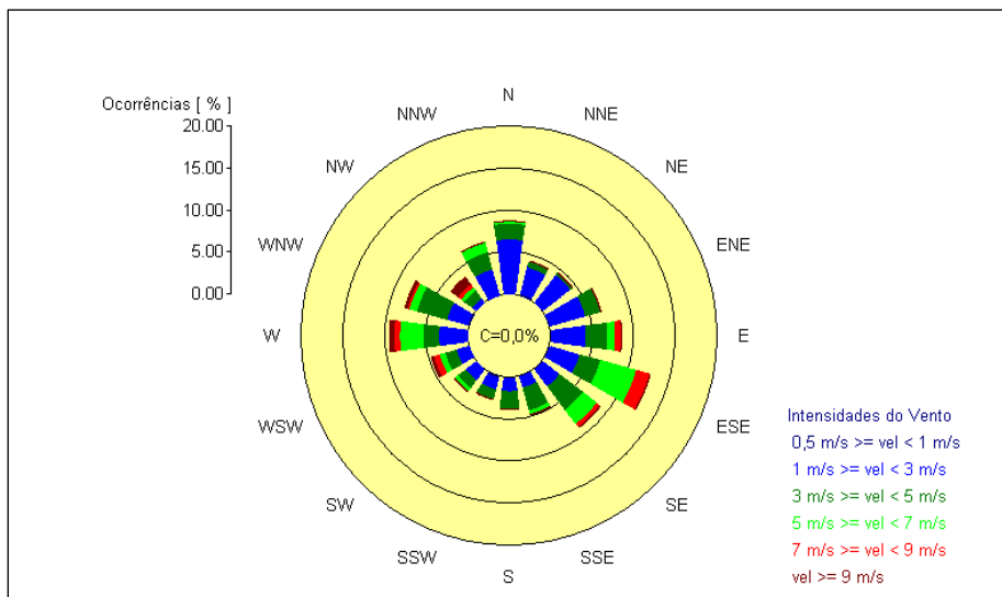
Figura 20 – Rosa dos Ventos – Estação Aceguá.
