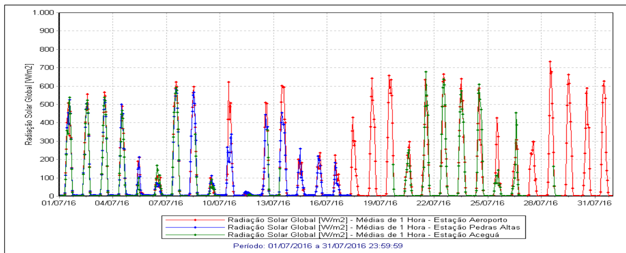
Figura 24 – Evolução das Medições de Radiação Solar.
