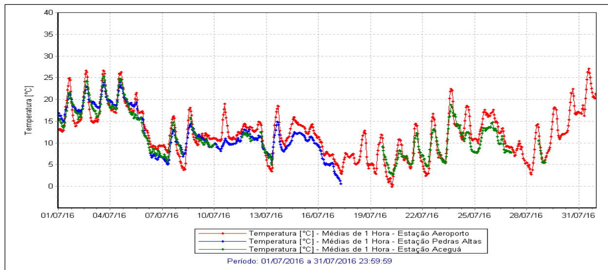
Figura 21 – Evolução das Medições de Temperatura.
