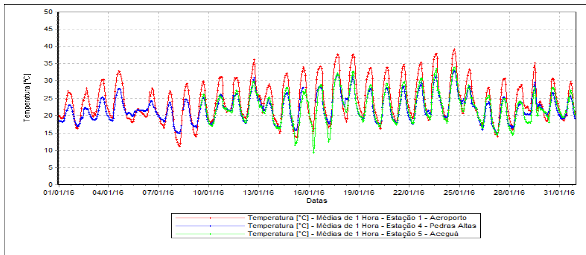
Figura 21 – Evolução das Medições de Temperatura.
