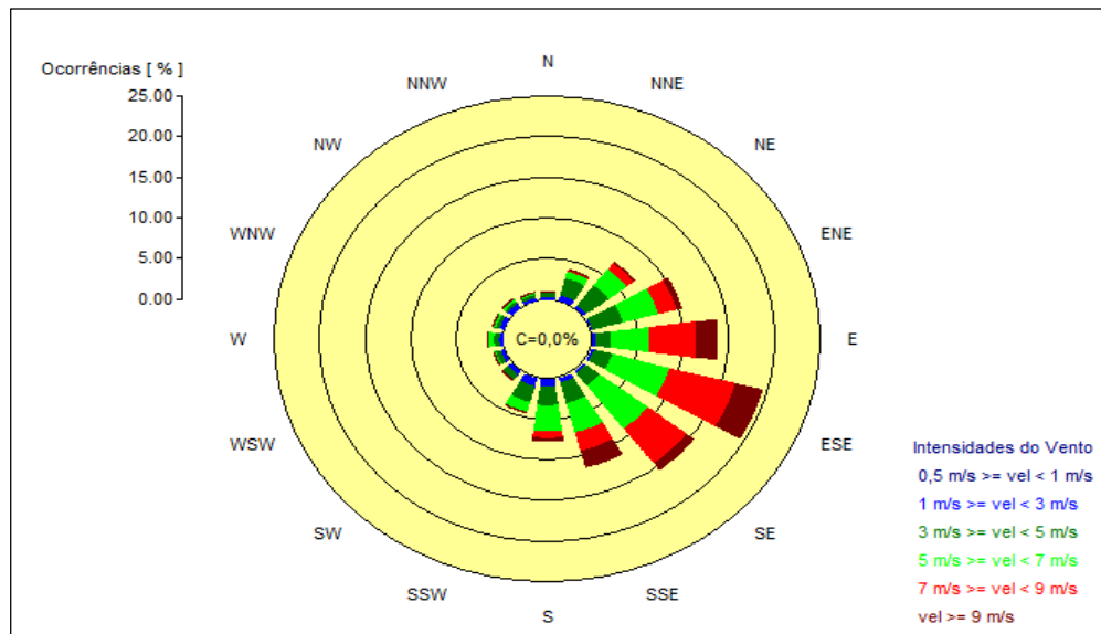
Figura 19 – Rosa dos Ventos – Estação Pedras Altas.
