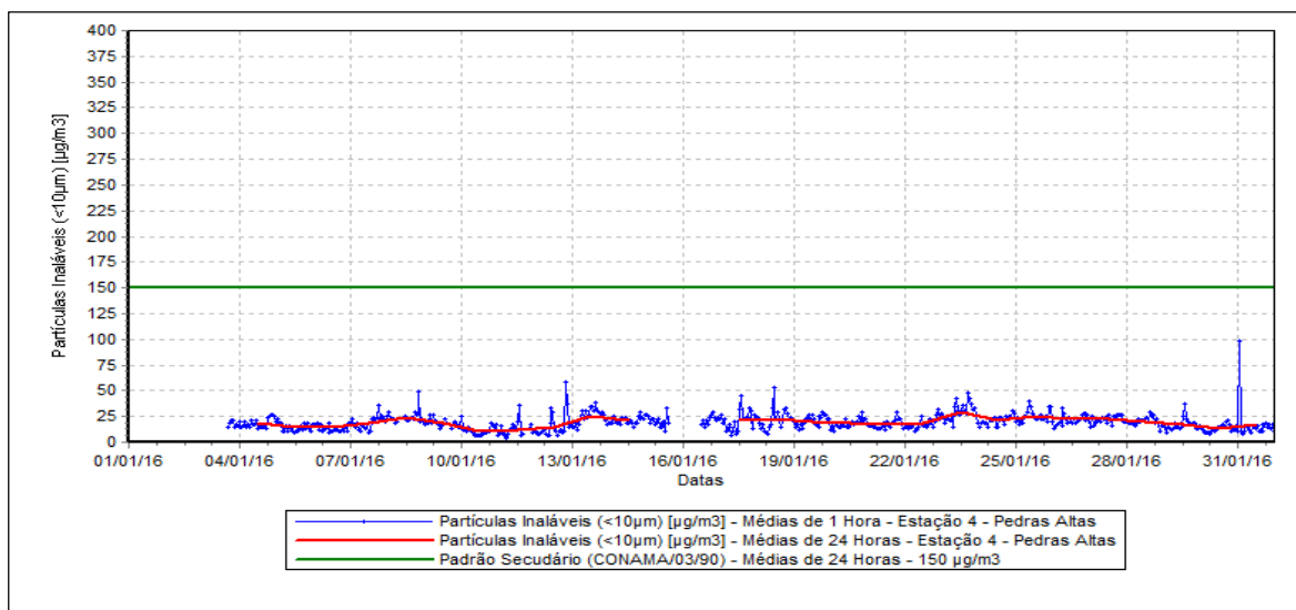
Figura 5 – Evolução da Concentração de Partículas Inaláveis - Estação Pedras Altas.
