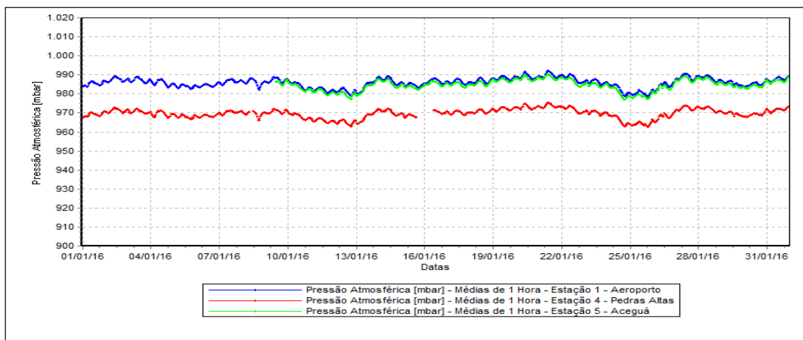
Figura 23 – Evolução das Medições de Pressão Atmosféricas.
