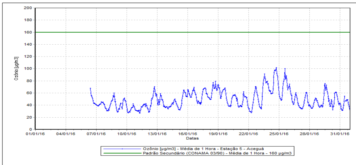
Figura 17 – Evolução das Concentrações de Ozônio – Estação Aceguá.
