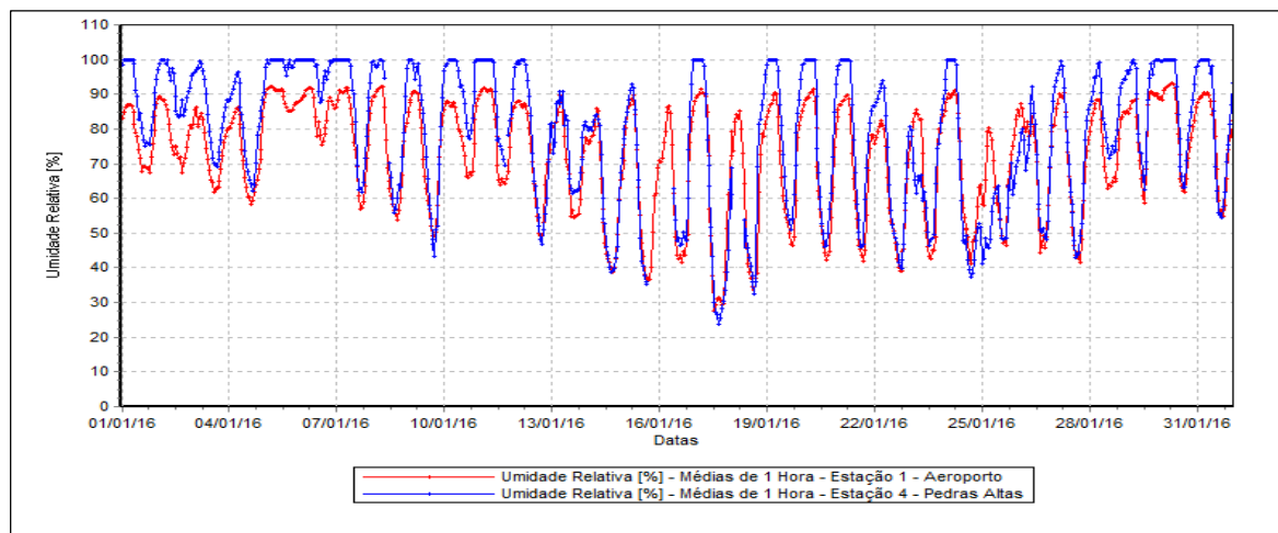
Figura 22 – Evolução das Medições de Umidade Relativa.
