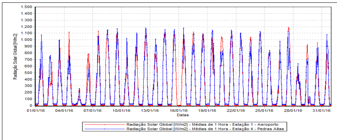
Figura 24 – Evolução das Medições de Radiação Solar.
