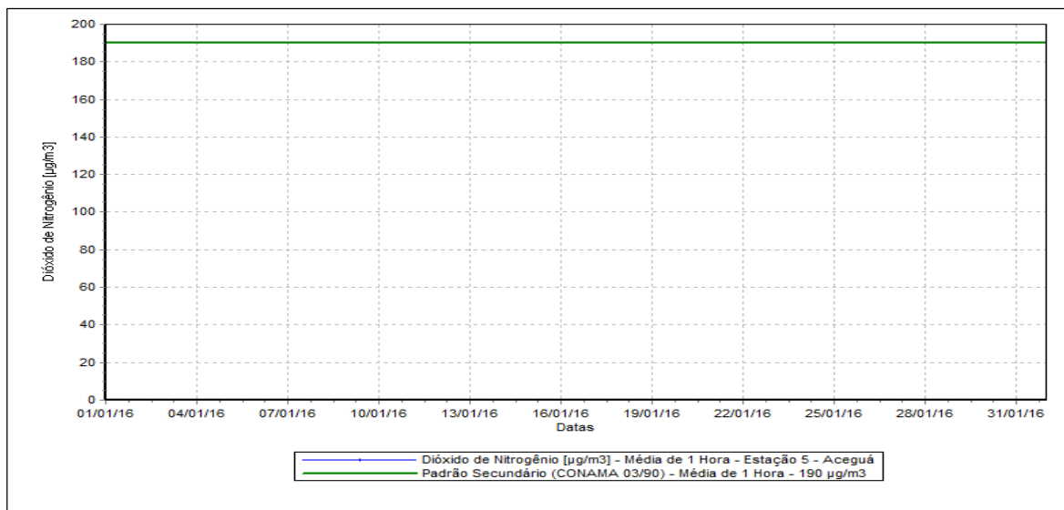
Figura 16 – Evolução das Concentrações de Dióxido de Nitrogênio – Estação Aceguá.
