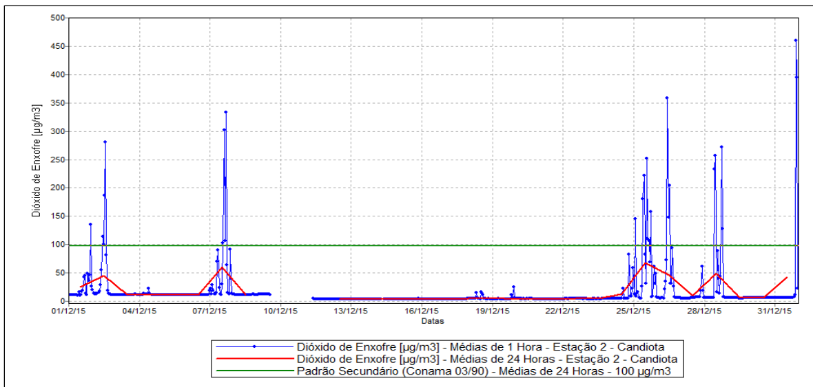
Figura 8 – Evolução das Concentrações de Dióxido de Enxofre – Estação Candiota.
