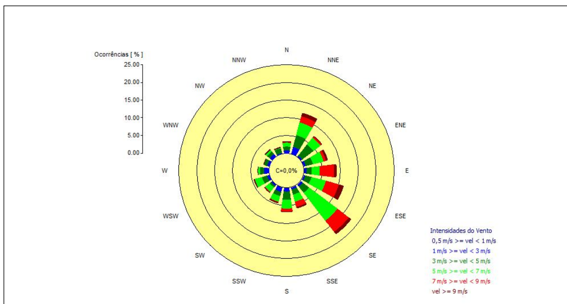
Figura 19 – Rosa dos Ventos – Estação Pedras Altas.
