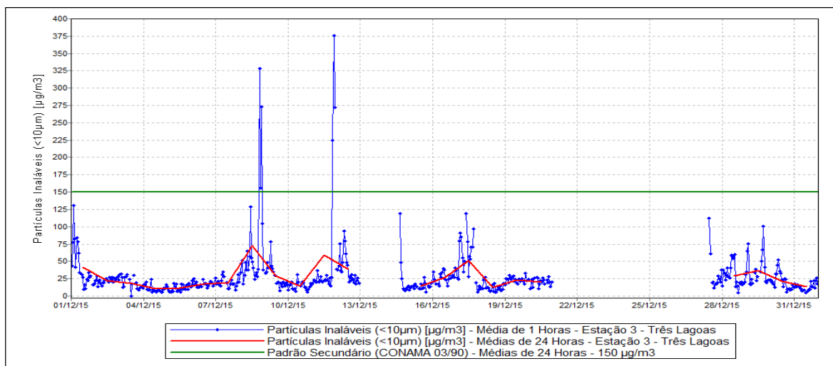
Figura 4 – Evolução da Concentração de Partículas Inaláveis - Estação Três Lagoas.
