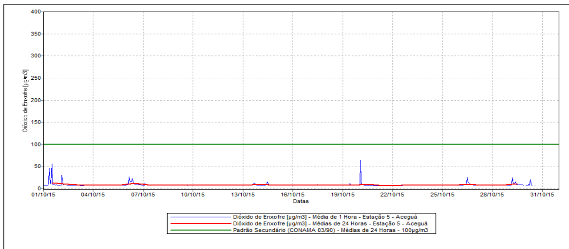
Figura 11 – Evolução das Concentrações de Dióxido de Enxofre – Estação Aceguá.
