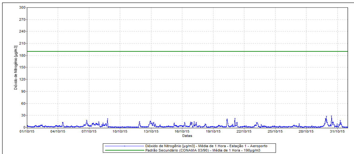
Figura 12 – Evolução das Concentrações de Dióxido de Nitrogênio – Estação Aeroporto.
