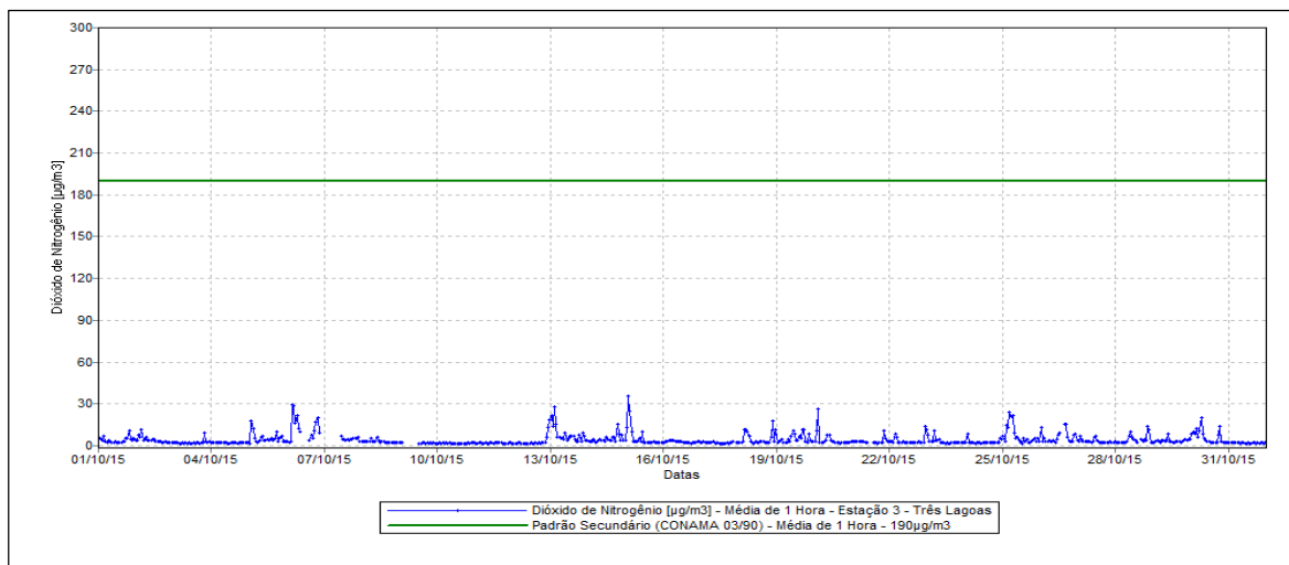
Figura 14 – Evolução das Concentrações de Dióxido de Nitrogênio – Estação Três Lagoas.
