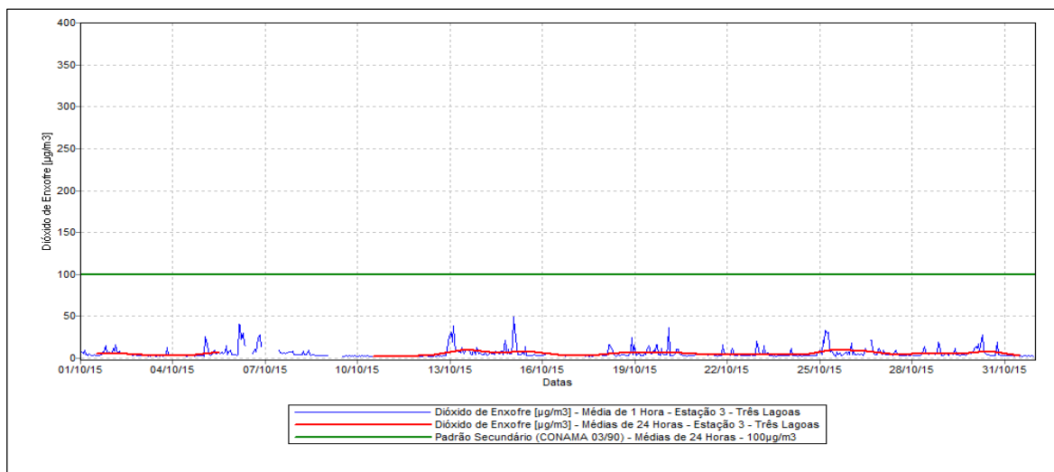
Figura 9 – Evolução das Concentrações de Dióxido de Enxofre – Estação Três Lagoas.
