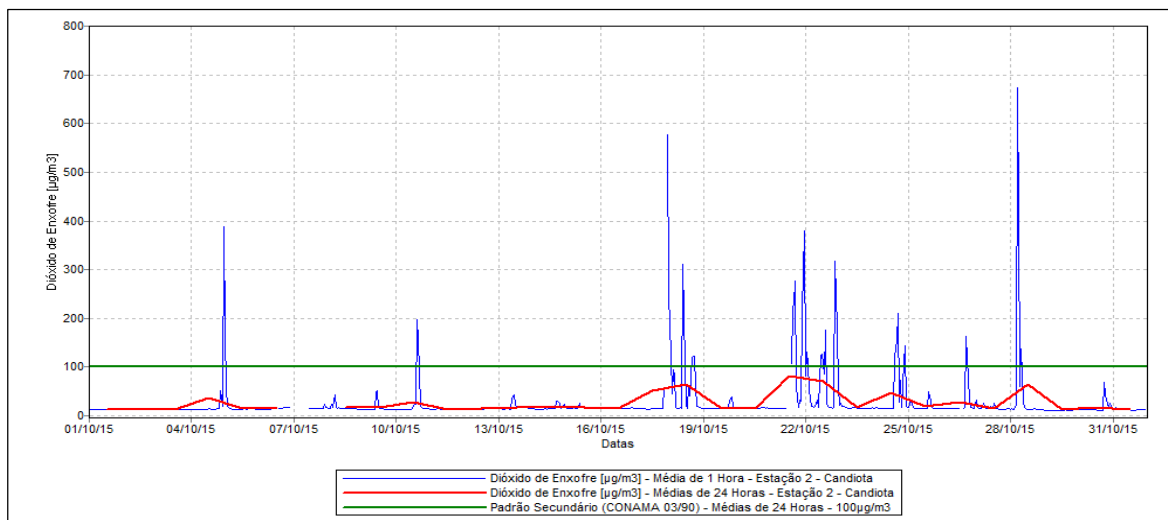
Figura 8 – Evolução das Concentrações de Dióxido de Enxofre – Estação Candiota.
