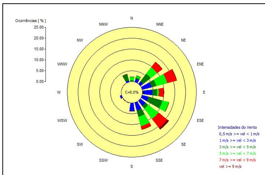
Figura 18 – Rosa dos Ventos – Estação Aeroporto.
