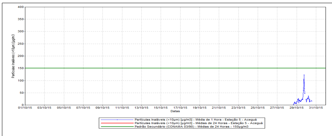
Figura 6 – Evolução da Concentração de Partículas Inaláveis - Estação Aceguá.
