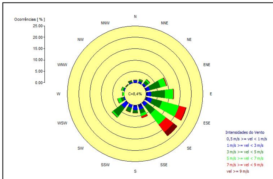
Figura 20 – Rosa dos Ventos – Estação Aceguá.
