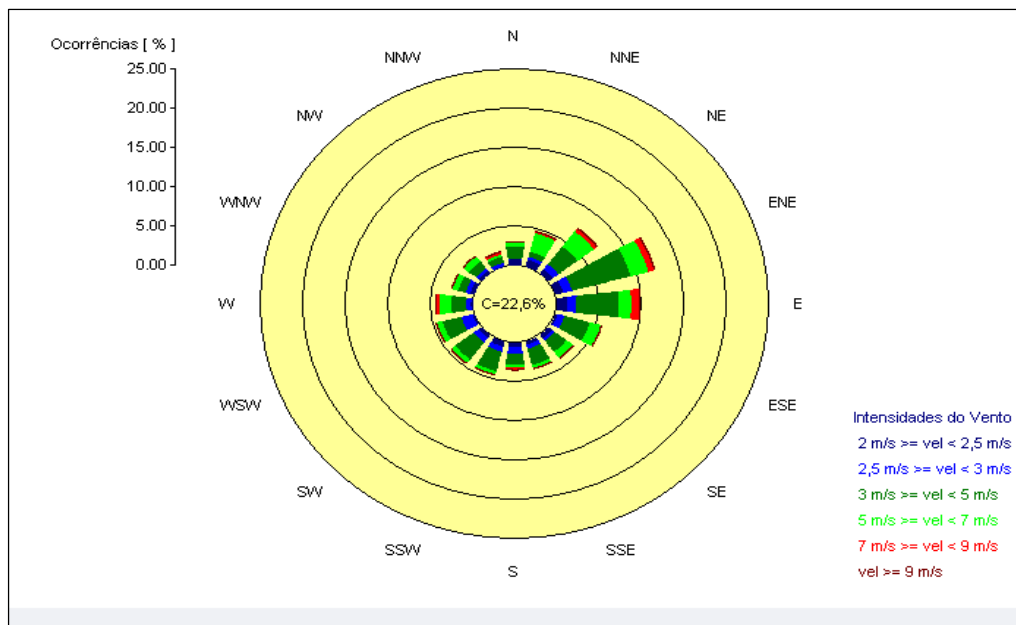
Figura 18 – Rosa dos Ventos – Estação Aeroporto.
