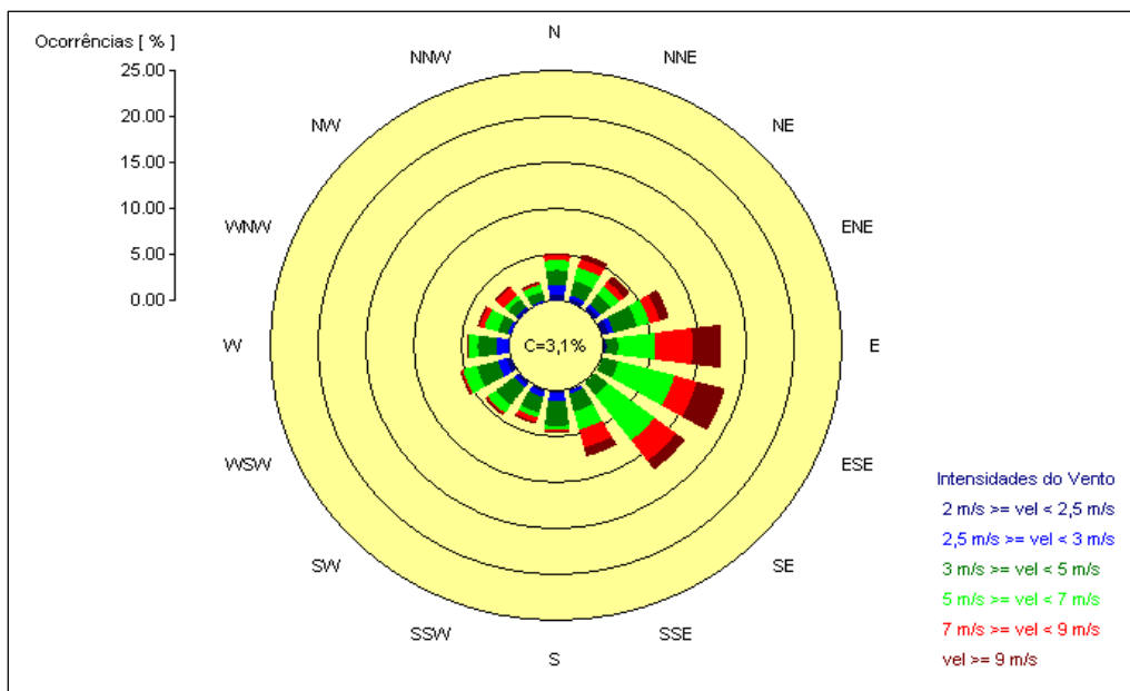
Figura 19 – Rosa dos Ventos – Estação Pedras Altas.
