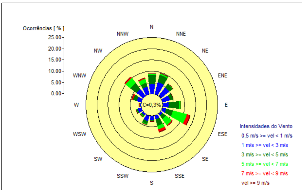
Figura 20 – Rosa dos Ventos – Estação Aceguá.
