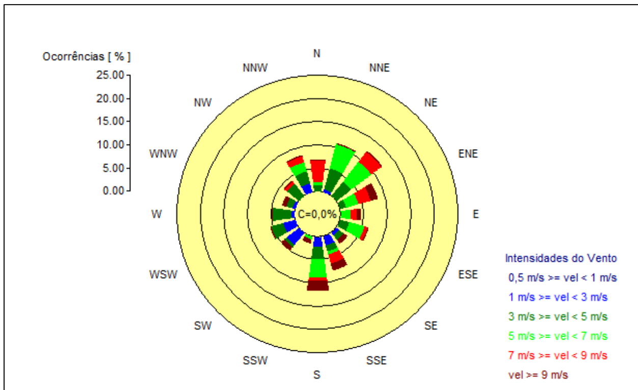
Figura 19 – Rosa dos Ventos – Estação Pedras Altas.
