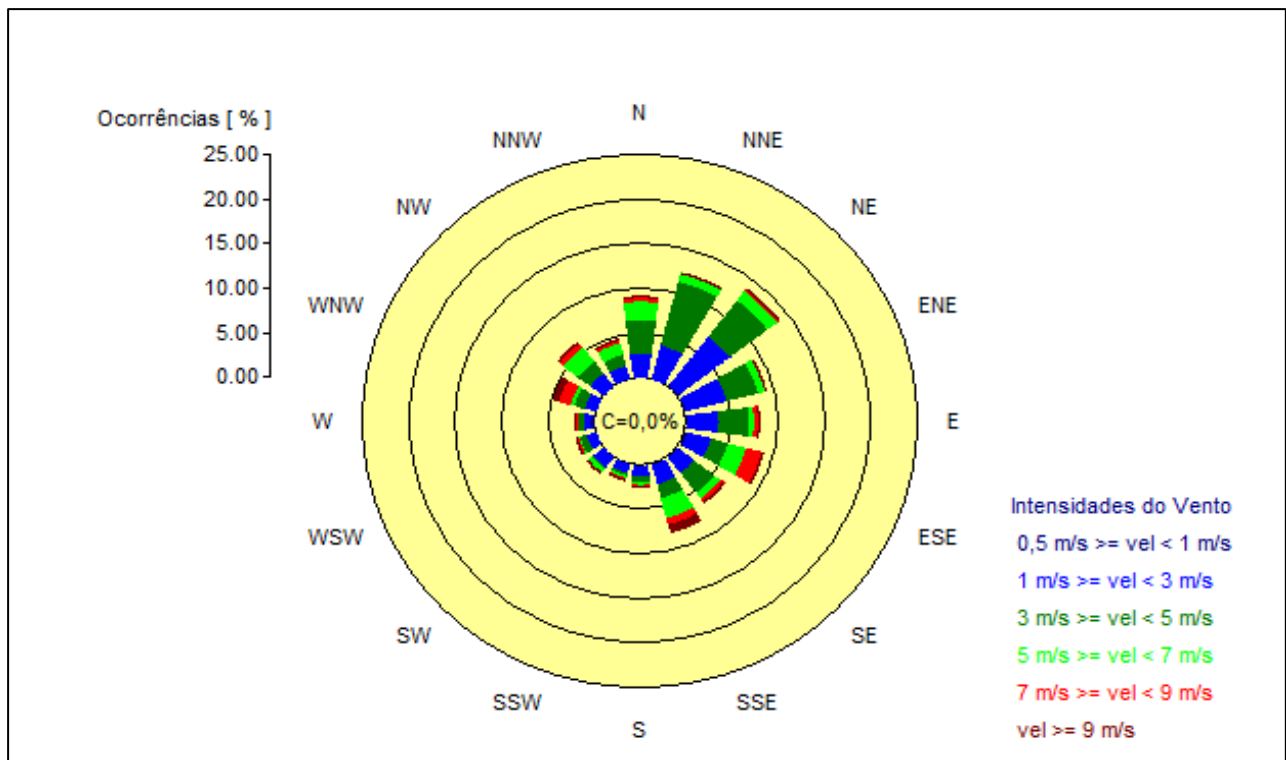
Figura 18 – Rosa dos Ventos – Estação Aeroporto.
