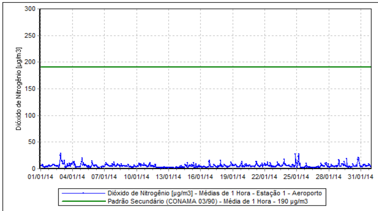
Figura 12 – Evolução das Concentrações de Dióxido de Nitrogênio – Estação Aeroporto.
