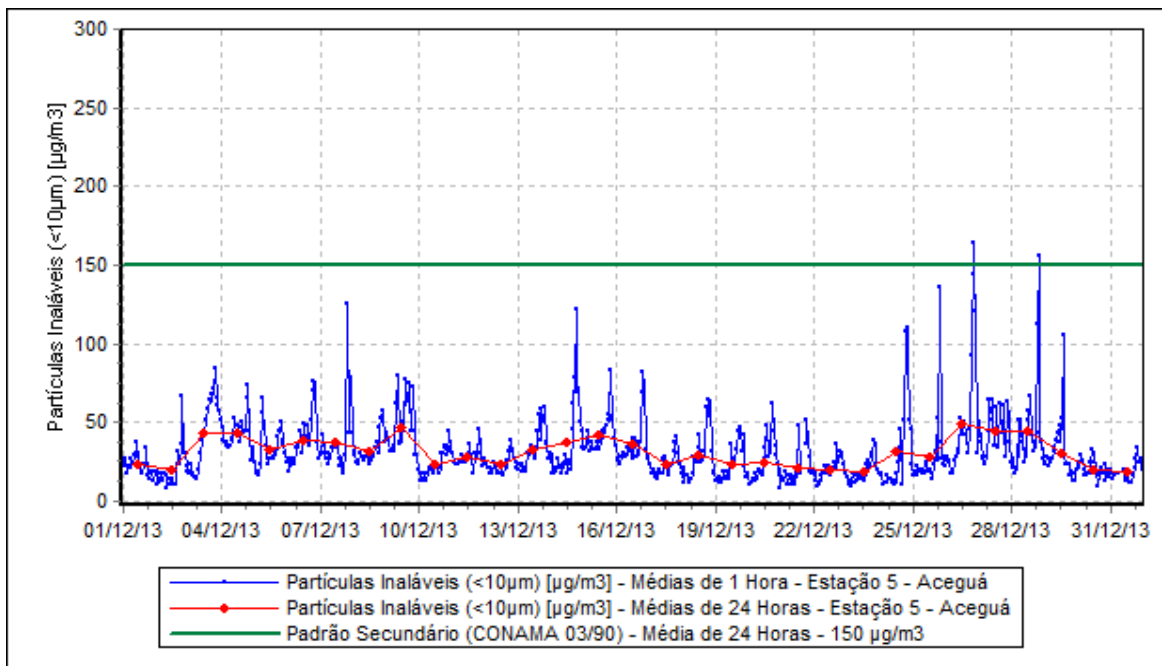
Figura 6 – Evolução da Concentração de Partículas Inaláveis - Estação Aceguá.
