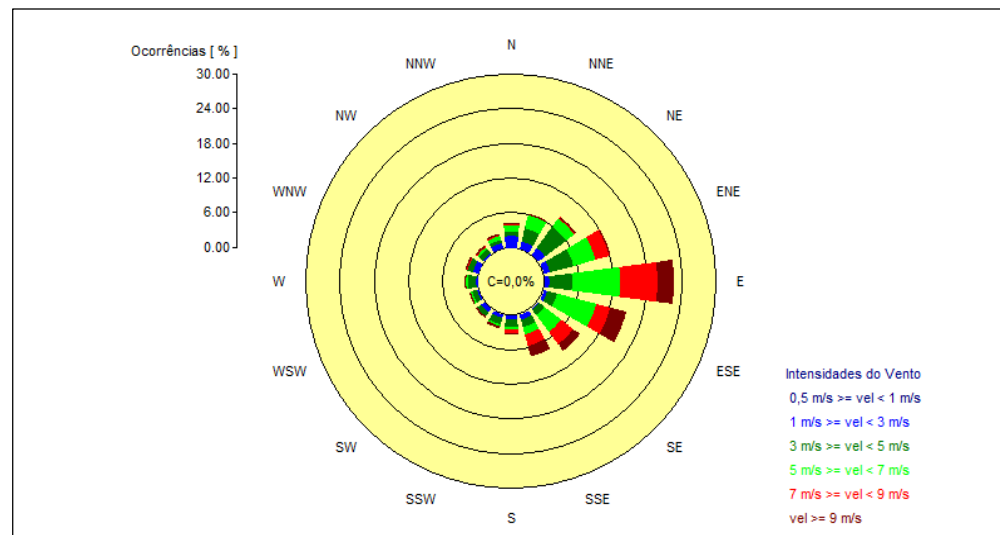
Figura 19 – Rosa dos Ventos – Estação Pedras Altas.
