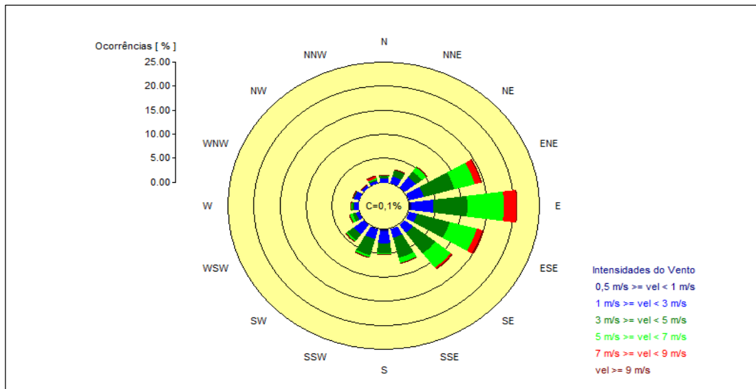
Figura 20 – Rosa dos Ventos – Estação Aceguá.
