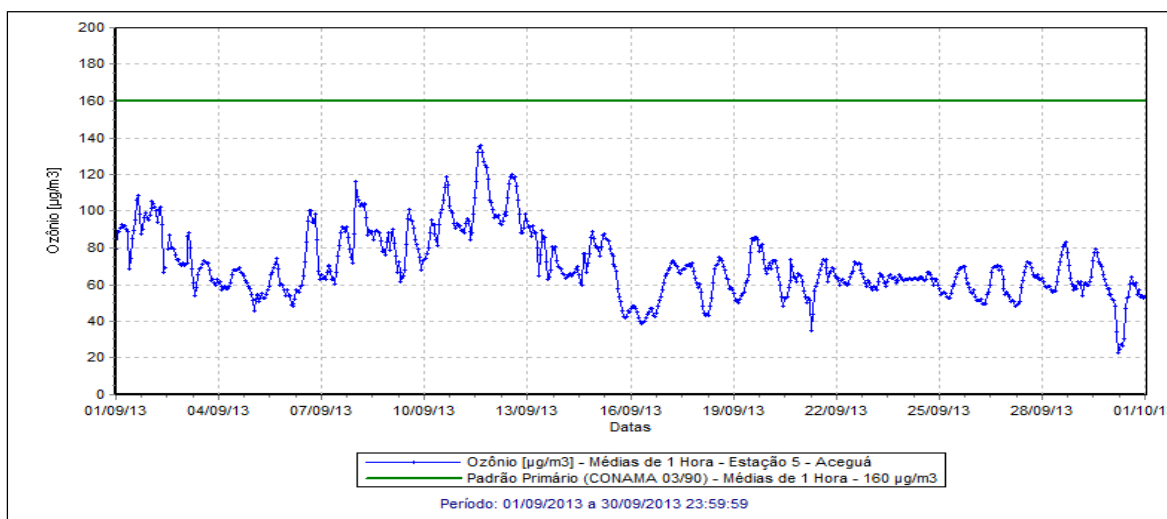
Figura 17 – Evolução das Concentrações de Ozônio – Estação Aceguá.
