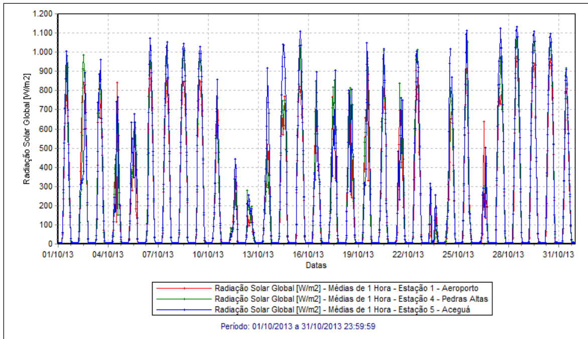
Figura 24 – Evolução das Medições de Radiação Solar.
