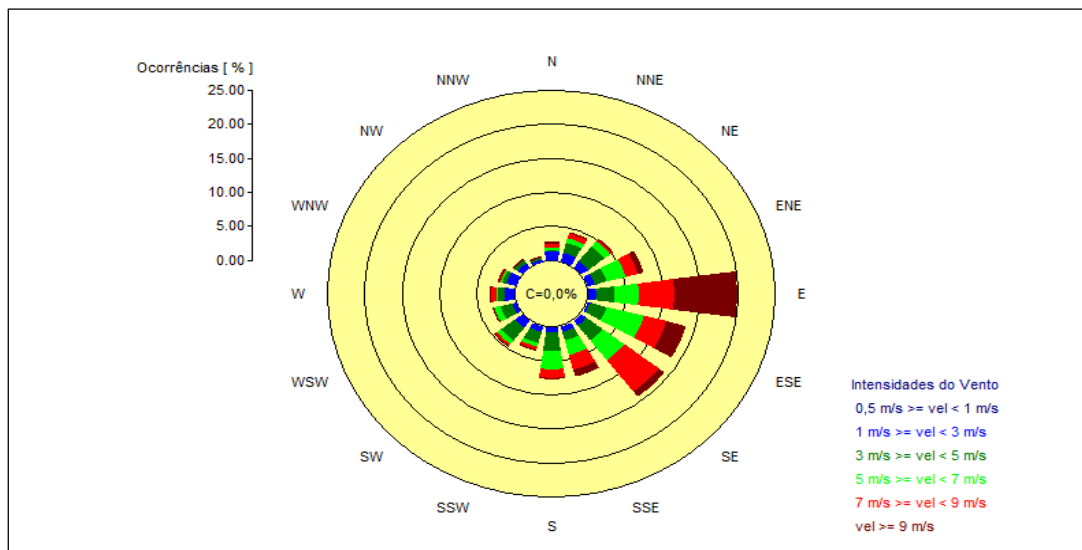
Figura 19 – Rosa dos Ventos – Estação Pedras Altas.
