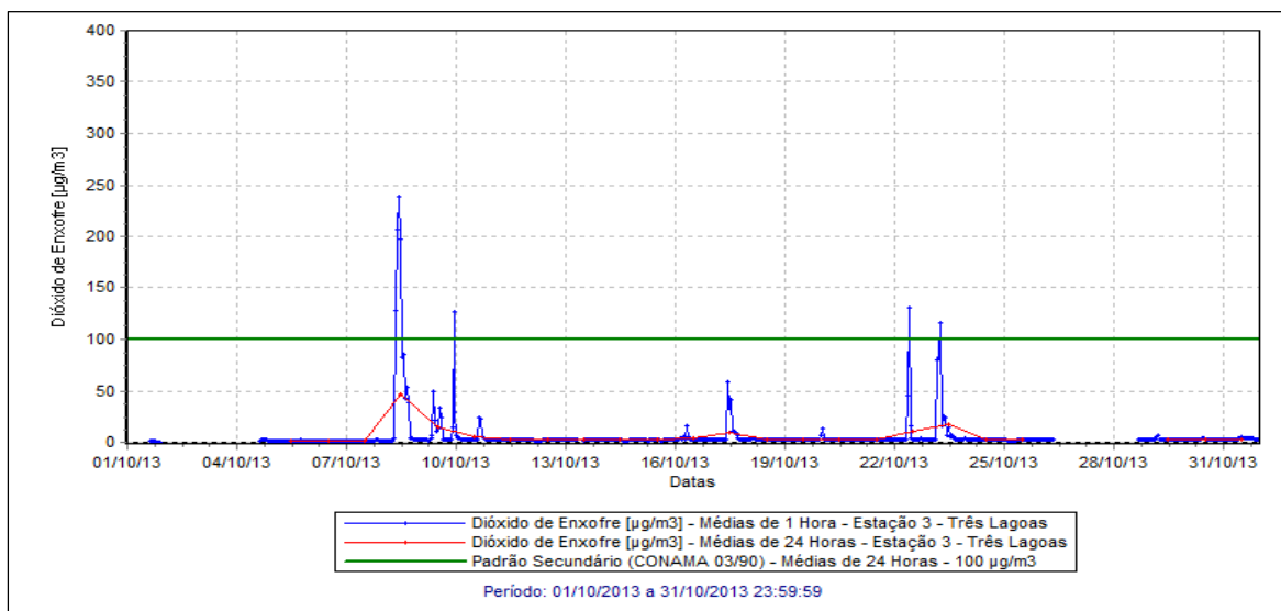
Figura 9 – Evolução das Concentrações de Dióxido de Enxofre – Estação Três Lagoas.
