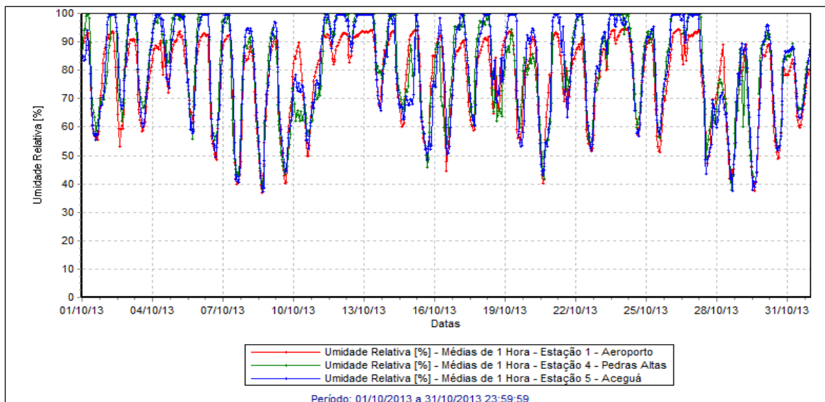
Figura 22 – Evolução das Medições de Umidade Relativa.
