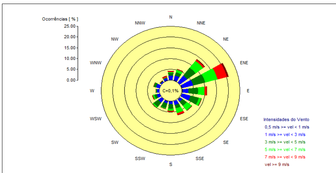
Figura 18 – Rosa dos Ventos – Estação Aeroporto.
