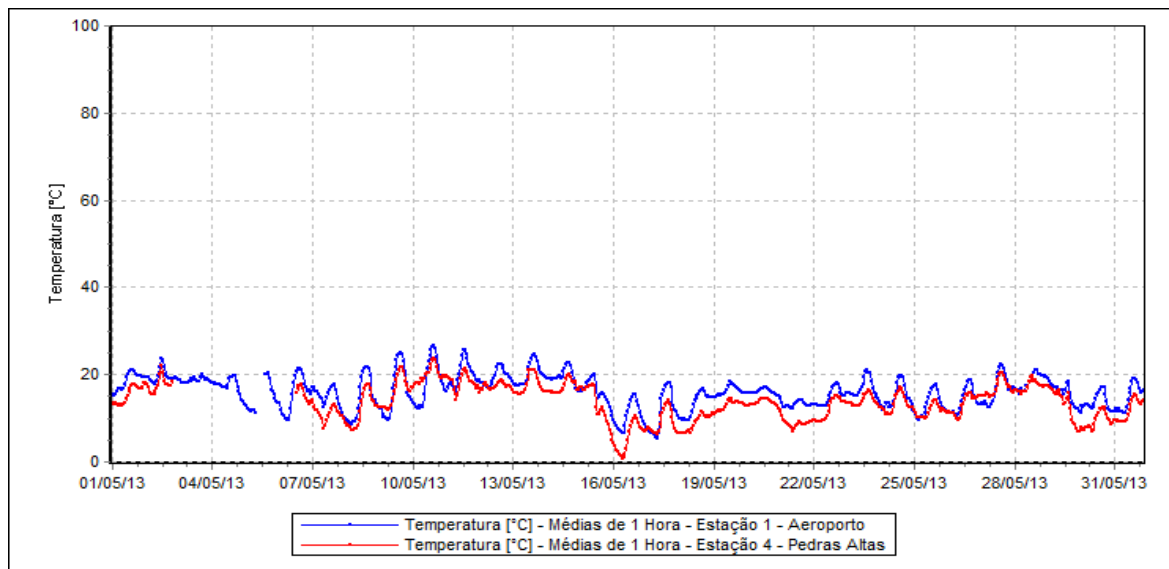
Figura 19 – Evolução das Medições de Temperatura.
