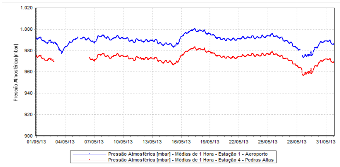
Figura 21 – Evolução das Medições de Pressão Atmosféricas.
