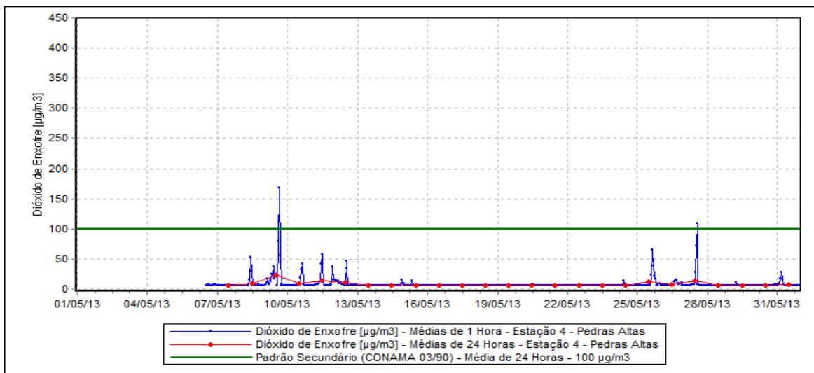
Figura 9 – Evolução das Concentrações de Dióxido de Enxofre – Estação Pedras Altas.
