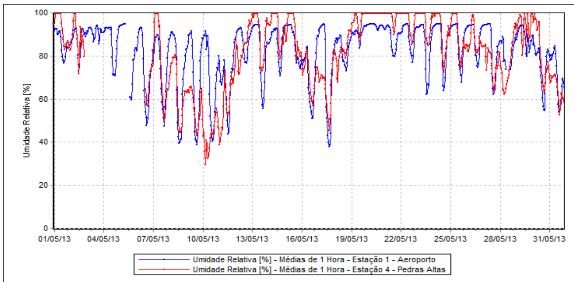
Figura 20 – Evolução das Medições de Umidade Relativa.
