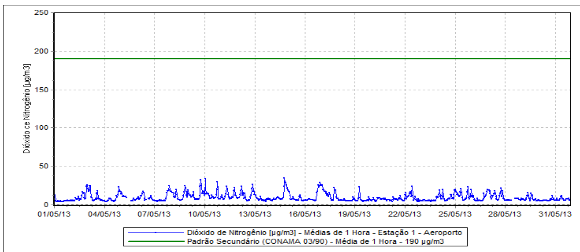
Figura 11 – Evolução das Concentrações de Dióxido de Nitrogênio – Estação Aeroporto.
