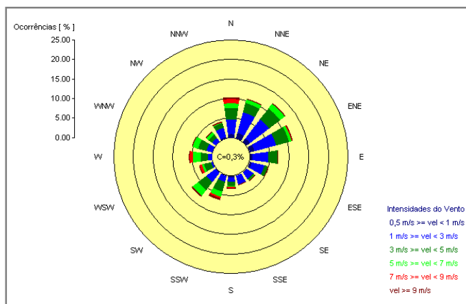
Figura 17 – Rosa dos Ventos – Estação Aeroporto.
