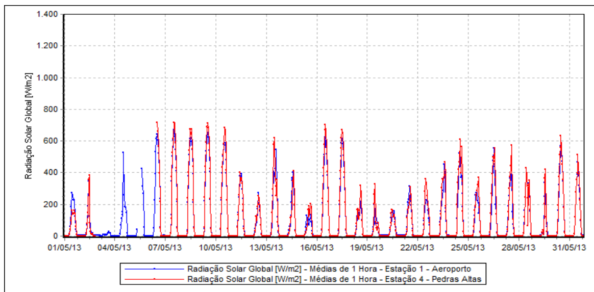
Figura 22 – Evolução das Medições de Radiação Solar.
