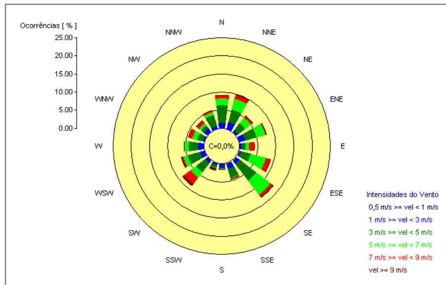
Figura 18 – Rosa dos Ventos – Estação Pedras Altas.
