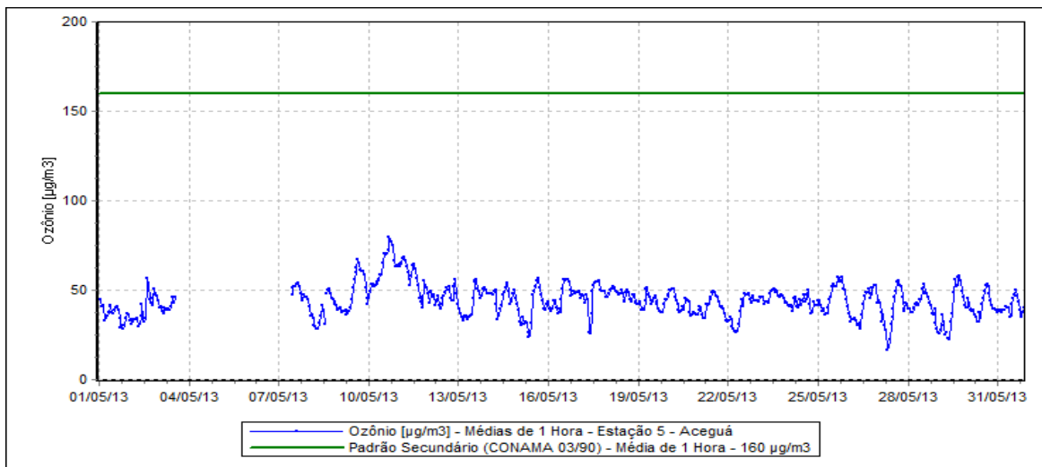
Figura 16 – Evolução das Concentrações de Ozônio – Estação Aceguá.
