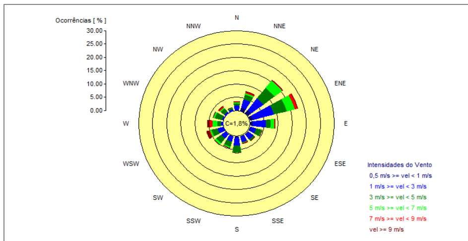
Figura 17 – Rosa dos Ventos – Estação Aeroporto.
