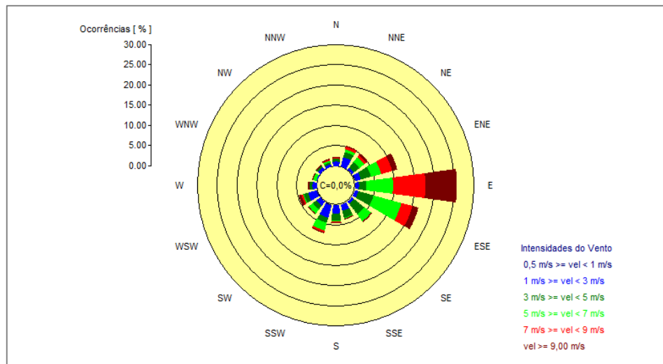
Figura 18 – Rosa dos Ventos – Estação Pedras Altas.
