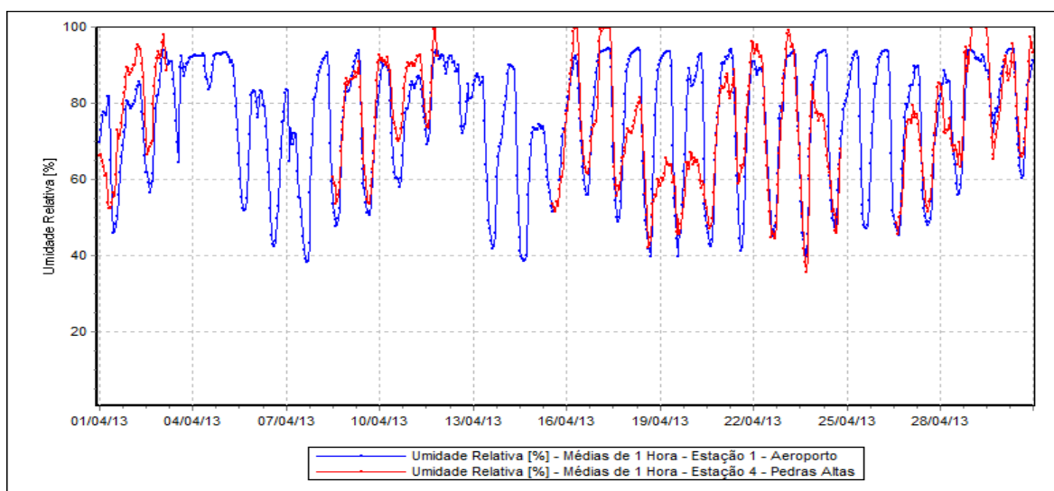
Figura 20 – Evolução das Medições de Umidade Relativa.
