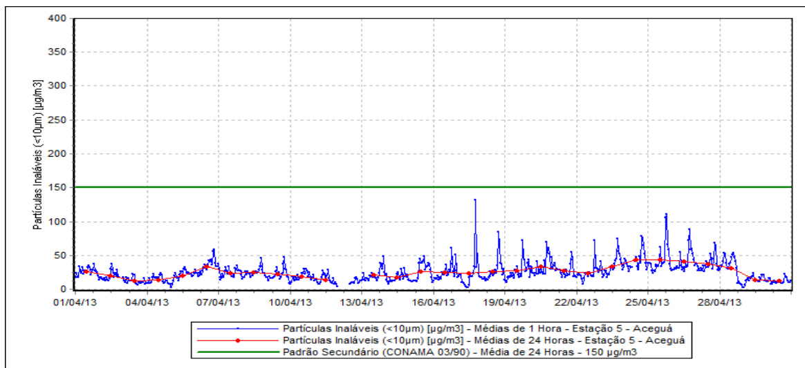
Figura 6 – Evolução das Concentrações de Partículas Inaláveis - Estação Aceguá.
