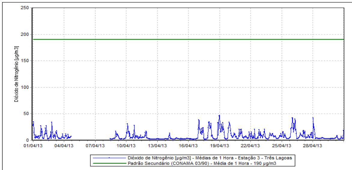
Figura 13 – Evolução das Concentrações de Dióxido de Nitrogênio – Estação Três Lagoas.
