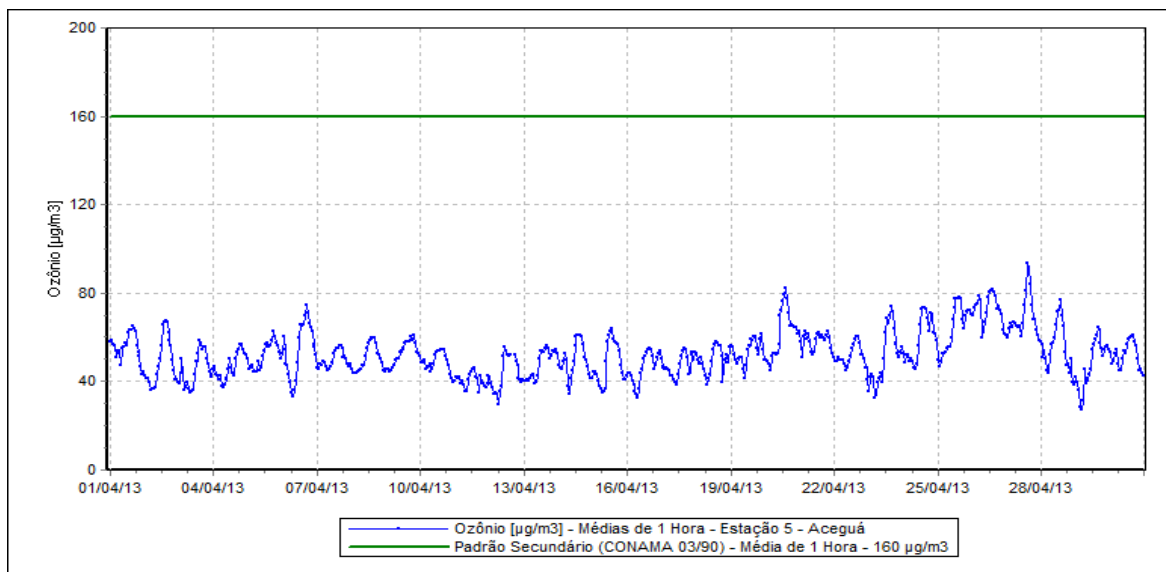
Figura 16 – Evolução das Concentrações de Ozônio – Estação Aceguá.
