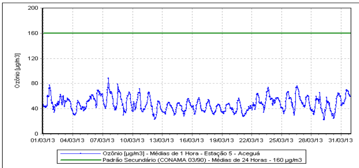
Figura 16 – Evolução das Concentrações de Ozônio – Estação Aceguá.
