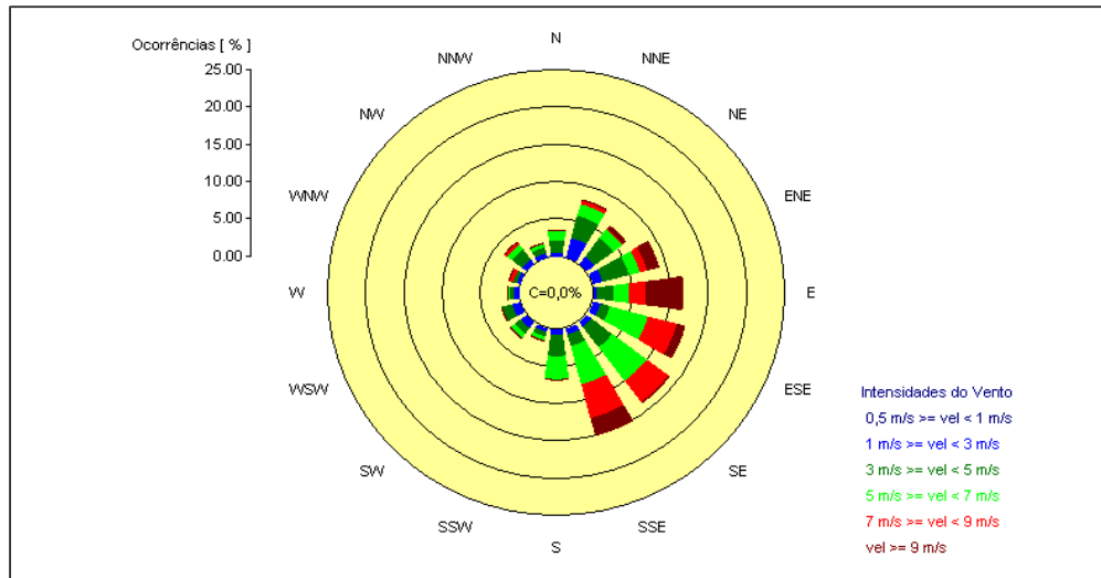
Figura 18 – Rosa dos Ventos – Estação Pedras Altas.
