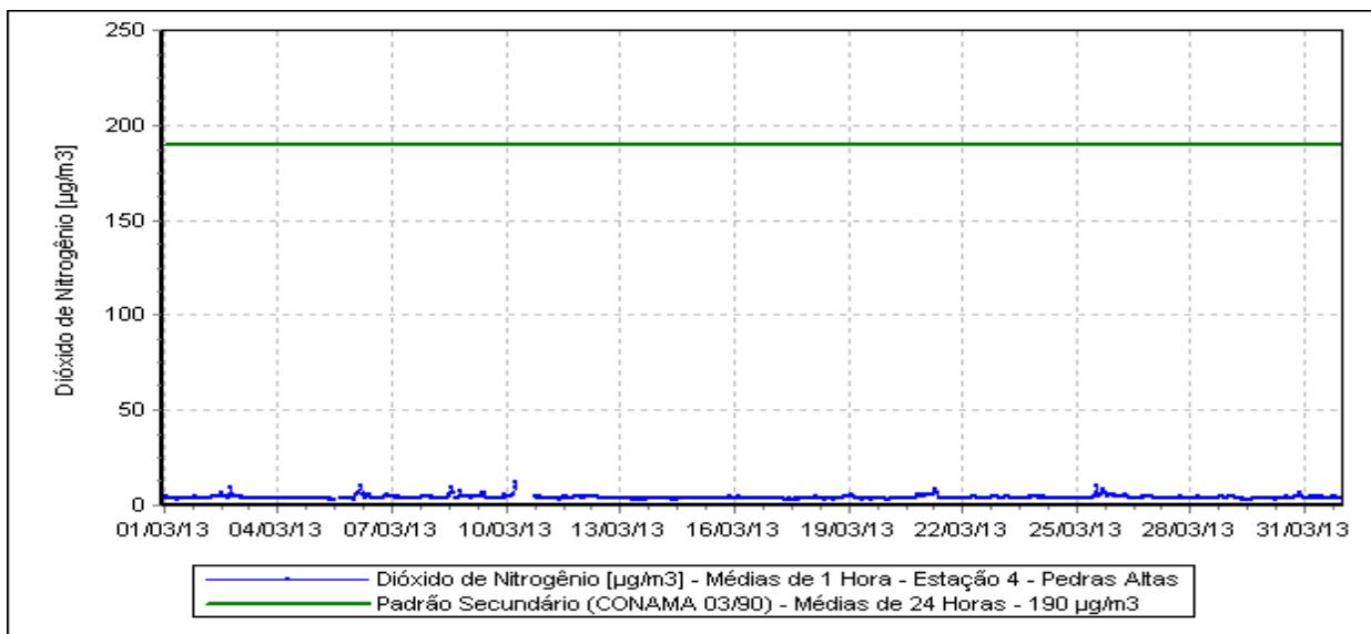
Figura 14 – Evolução das Concentrações de Dióxido de Nitrogênio – Estação Pedras Altas.
