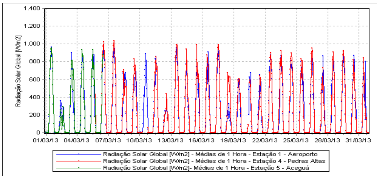
Figura 23 – Evolução das Medições de Radiação Solar.
