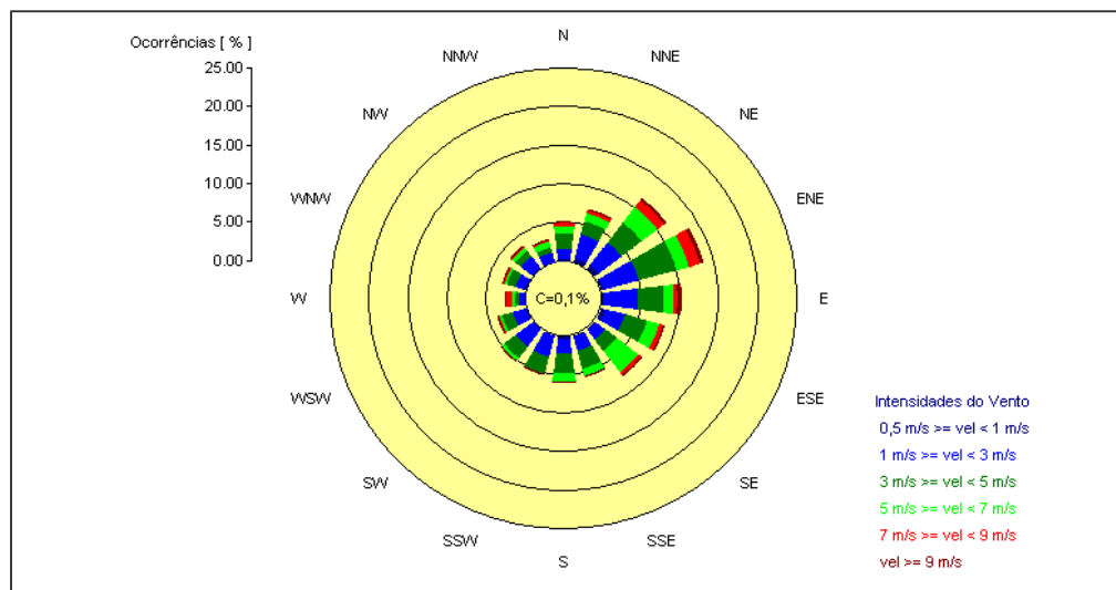
Figura 17 – Rosa dos Ventos – Estação Aeroporto.
