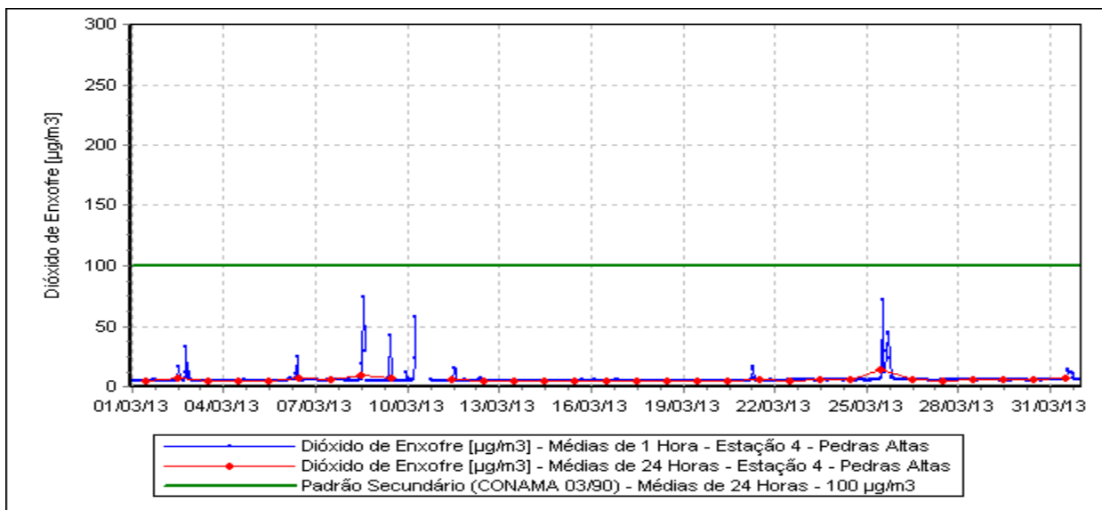
Figura 9 – Evolução das Concentrações de Dióxido de Enxofre – Estação Pedras Altas.
