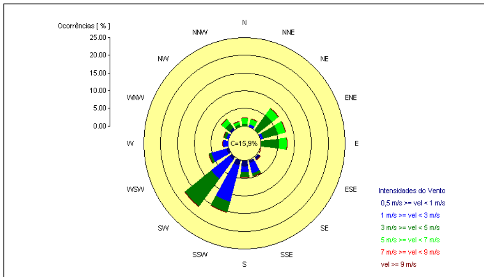
Figura 19 – Rosa dos Ventos – Estação Aceguá.
