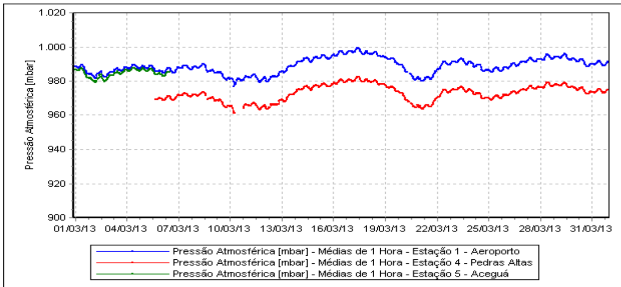
Figura 22 – Evolução das Medições de Pressão Atmosféricas.
