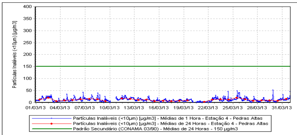
Figura 5 – Evolução das Concentrações de Partículas Inaláveis - Estação Pedras Altas.
