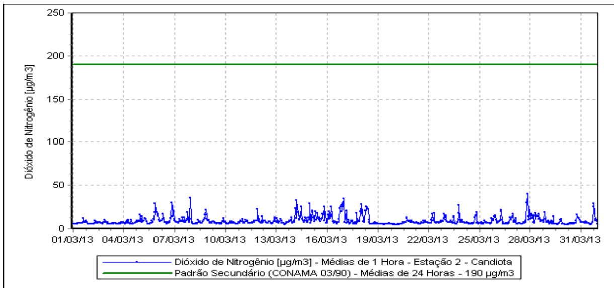
Figura 12 – Evolução das Concentrações de Dióxido de Nitrogênio – Estação Candiota.
