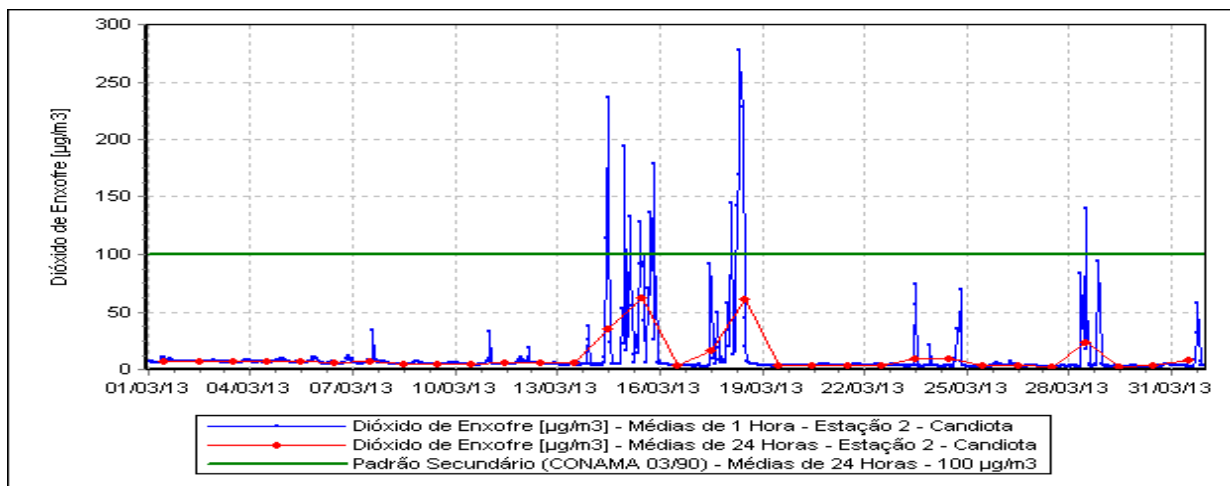
Figura 7 – Evolução das Concentrações de Dióxido de Enxofre – Estação Candiota.
