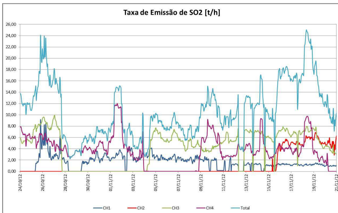
Figura 25 – Evolução das taxas de emissão para o período de testes da Unidade III de Candiota II.
