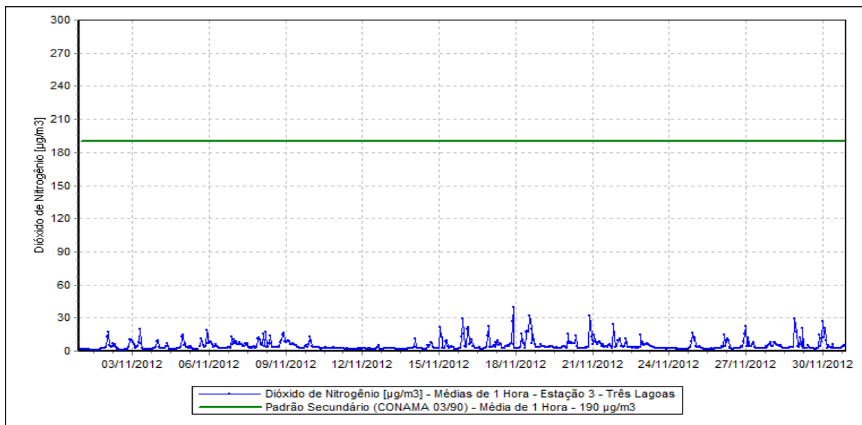
Figura 13 – Evolução das Concentrações de Dióxido de Nitrogênio – Estação Três Lagoas.
