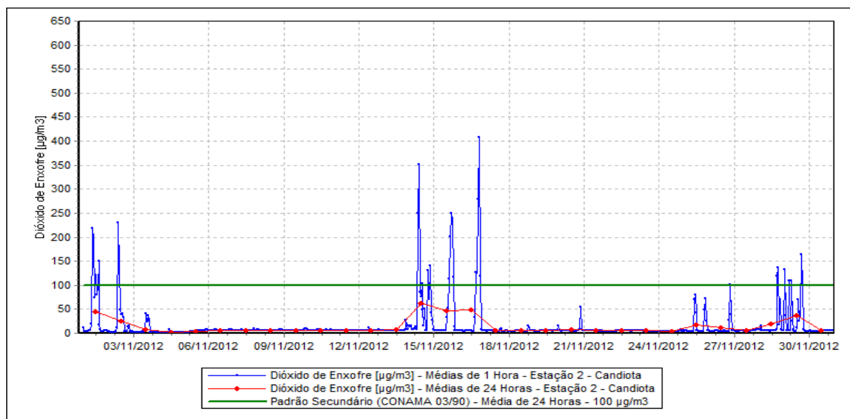
Figura 7 – Evolução das Concentrações de Dióxido de Enxofre – Estação Candiota.
