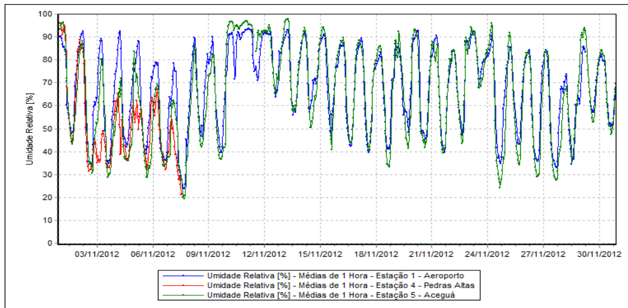
Figura 21 – Evolução das Medições de Umidade Relativa.
