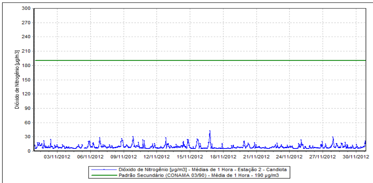
Figura 12 – Evolução das Concentrações de Dióxido de Nitrogênio – Estação Candiota.
