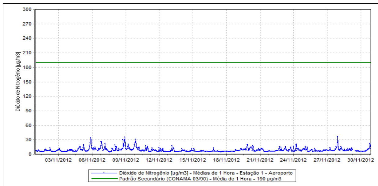
Figura 11 – Evolução das Concentrações de Dióxido de Nitrogênio – Estação Aeroporto.
