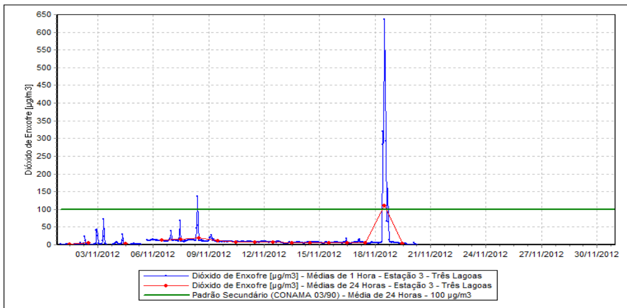
Figura 8 – Evolução das Concentrações de Dióxido de Enxofre – Estação Três Lagoas.
