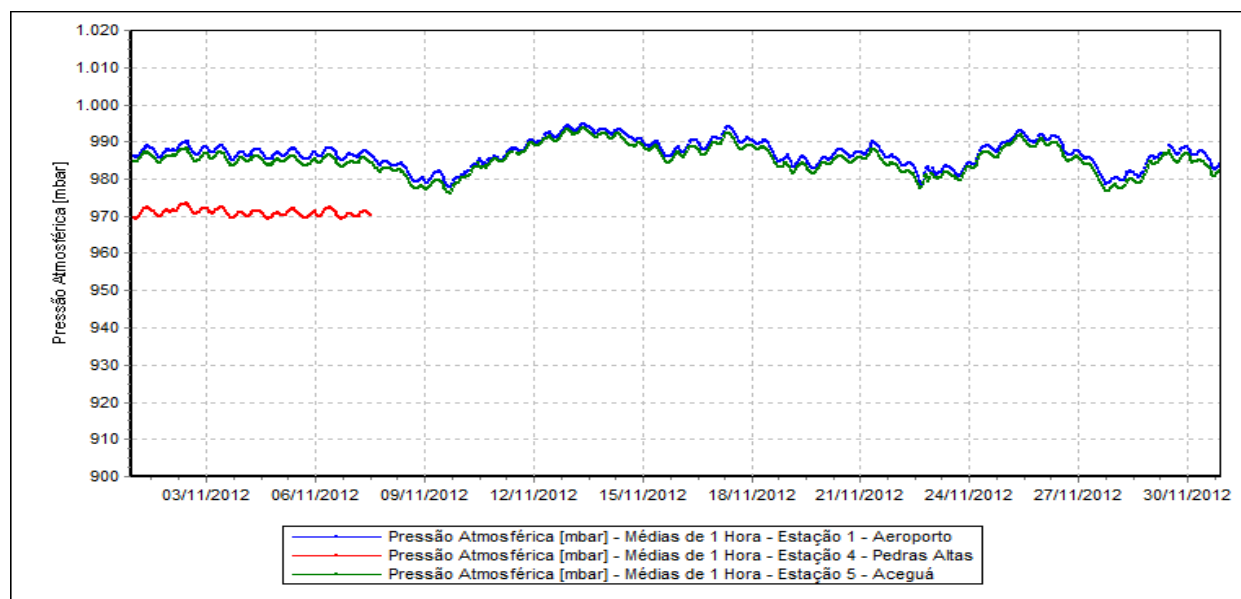
Figura 22 – Evolução das Medições de Pressão Atmosféricas.
