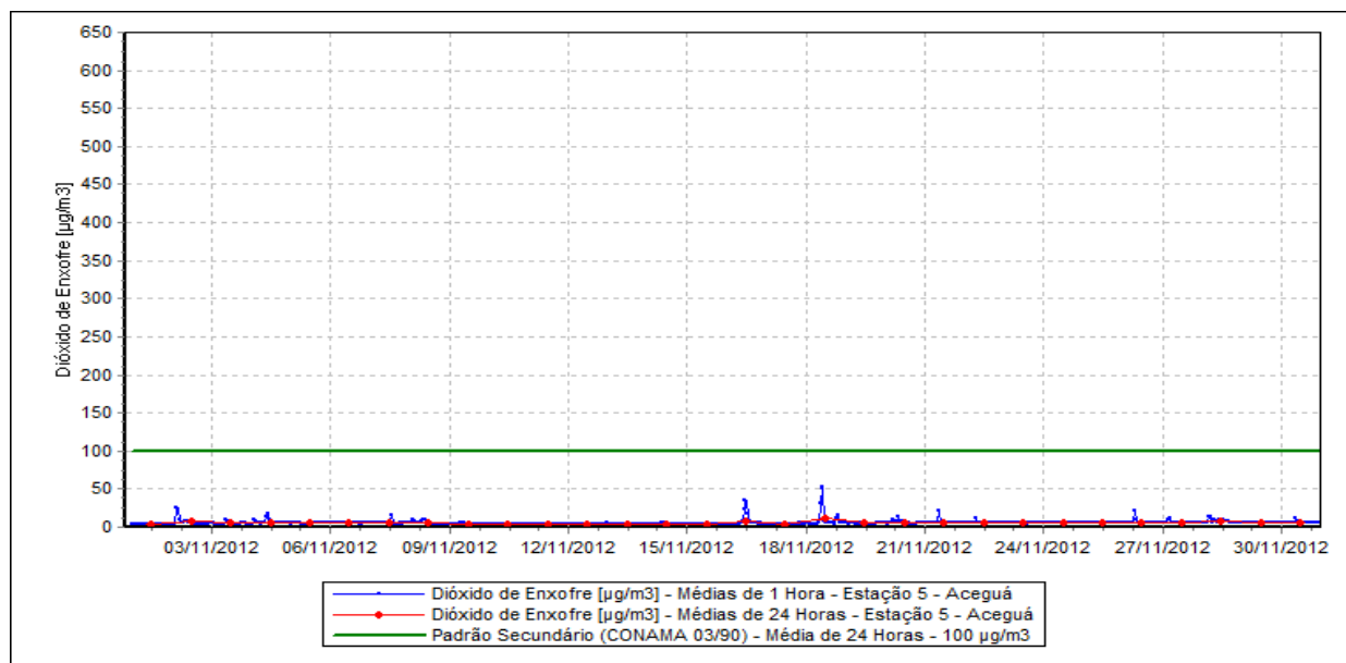
Figura 10 – Evolução das Concentrações de Dióxido de Enxofre – Estação Aceguá.
