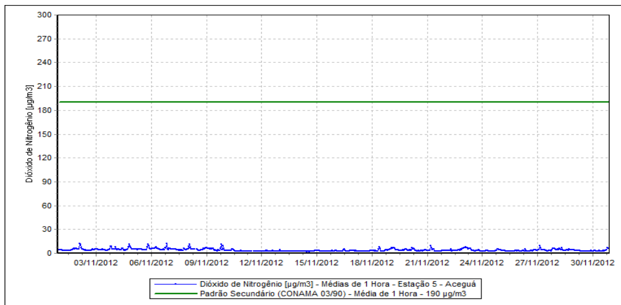
Figura 15 – Evolução das Concentrações de Dióxido de Nitrogênio – Estação Aceguá.
