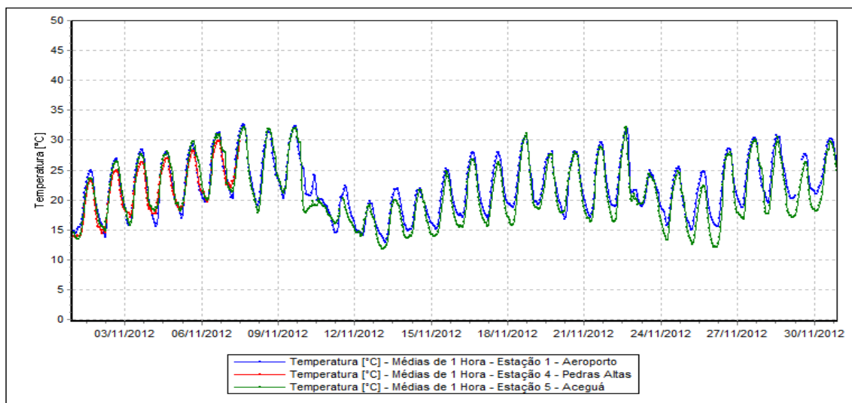
Figura 20 – Evolução das Medições de Temperatura.
