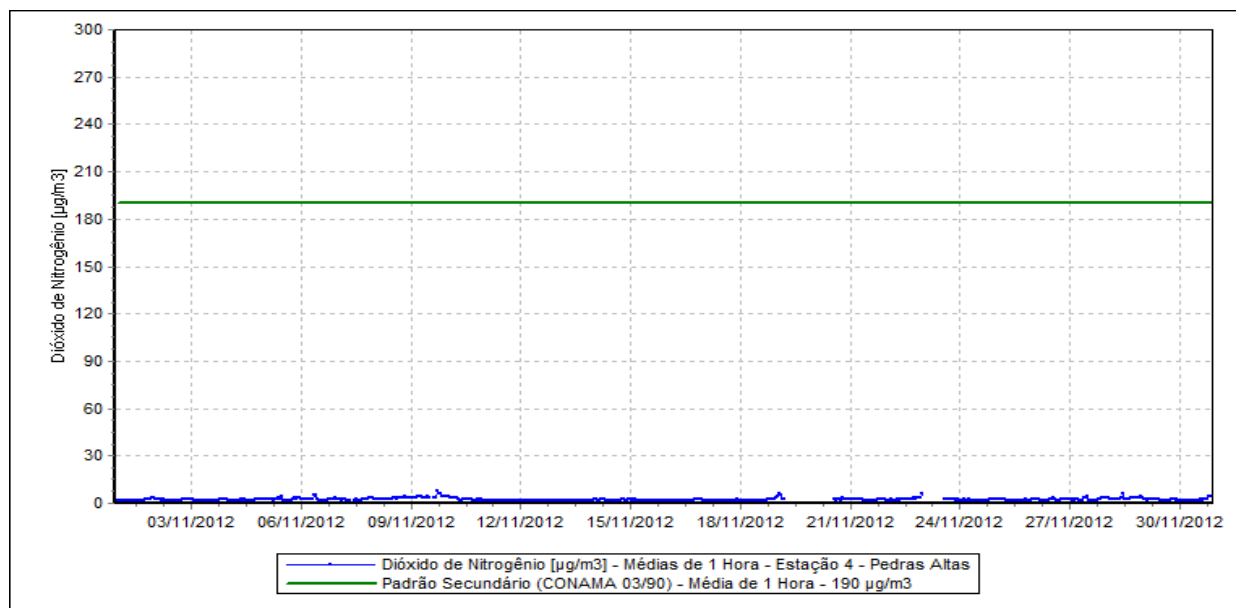
Figura 14 – Evolução das Concentrações de Dióxido de Nitrogênio – Estação Pedras Altas.
