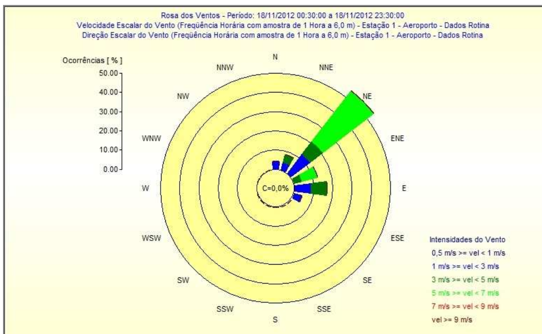
Figura 24 – Rosa dos Ventos – Estação Aeroporto na data de 18/11/2012.
