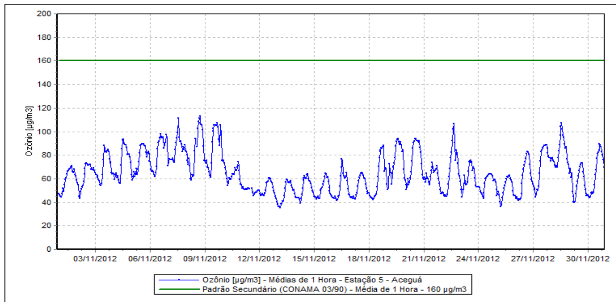
Figura 16 – Evolução das Concentrações de Ozônio – Estação Aceguá.
