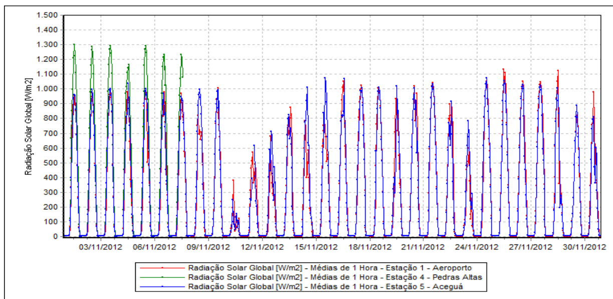
Figura 23 – Evolução das Medições de Radiação Solar.
