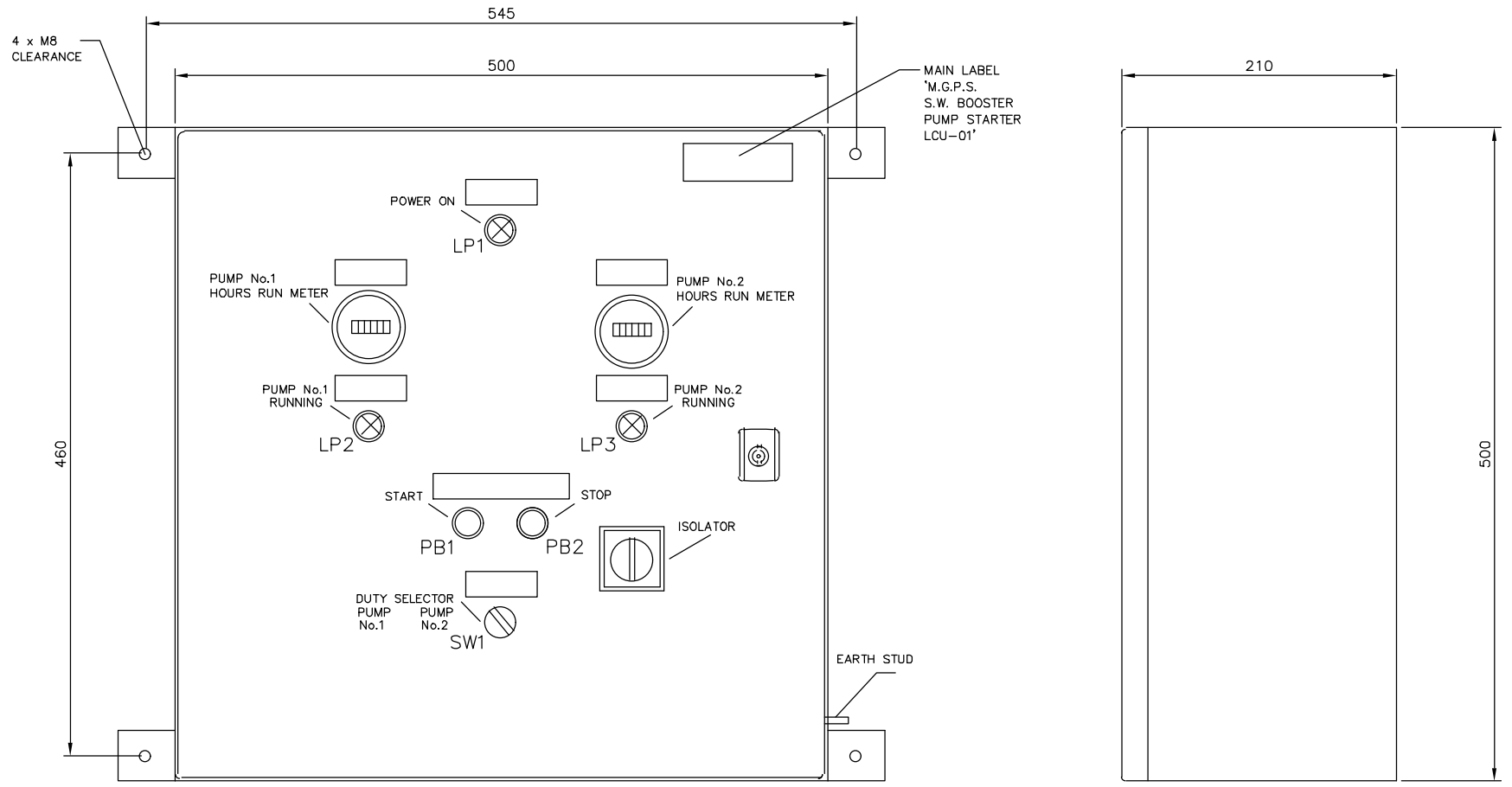
EXTERNAL DOOR LAYOUT
