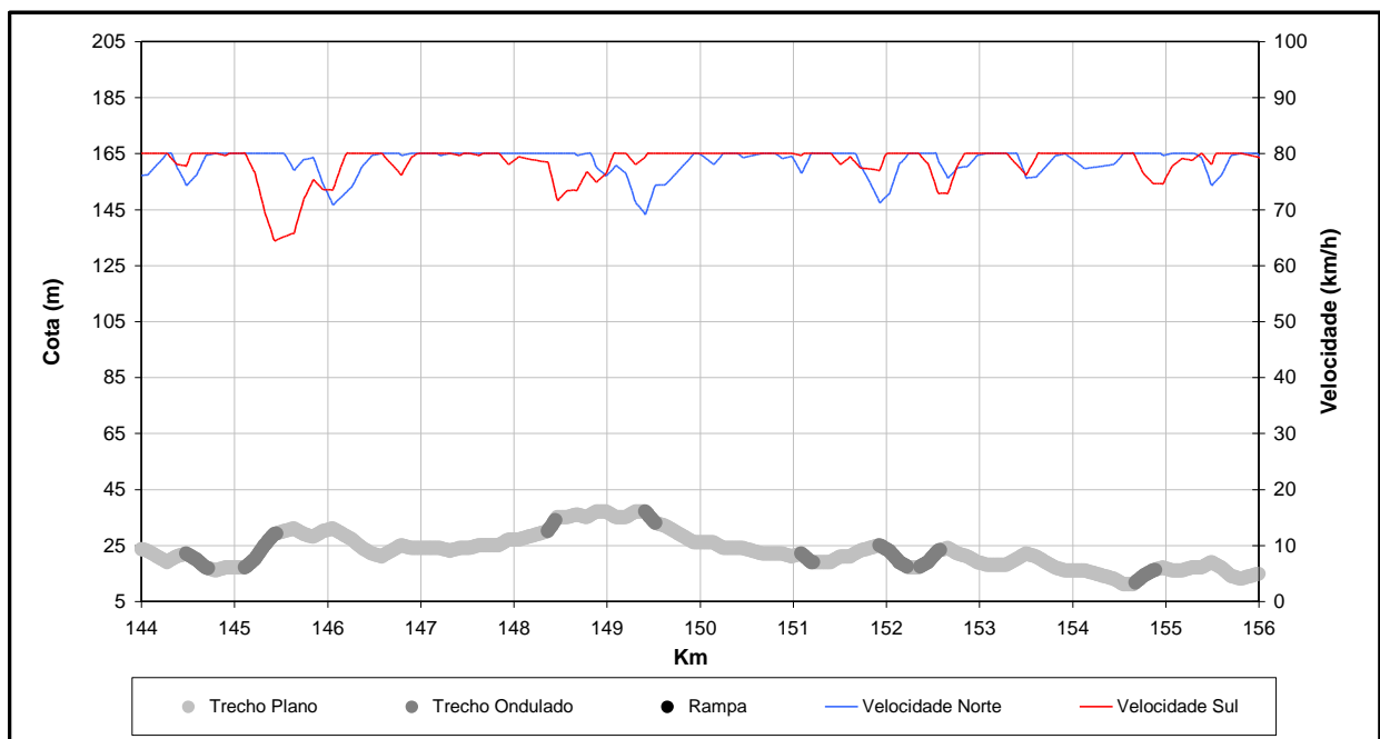
Figura 3.1f: Perfil Vertical da BR 101 RJ – km 144 ao km 156
