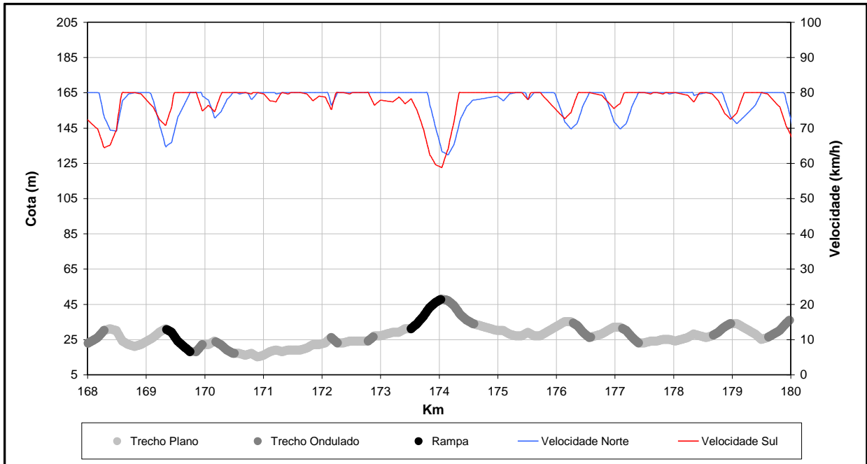
Figura 3.1h: Perfil Vertical da BR 101 RJ – km 168 ao km 180
