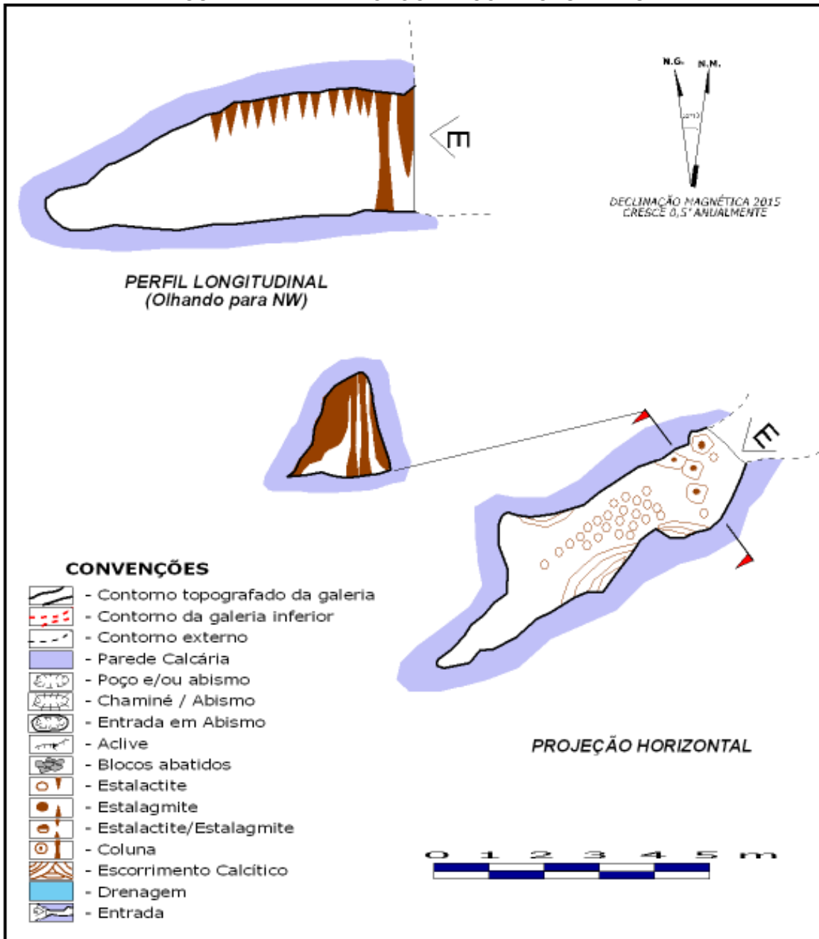
FIGURA 4.47 – MAPA TOPOGRÁFICO DA GRUTA DES II
