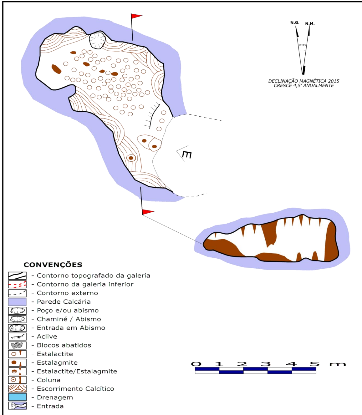
FIGURA 3.23 – MAPA TOPOGRÁFICO DA GRUTA DES IV
