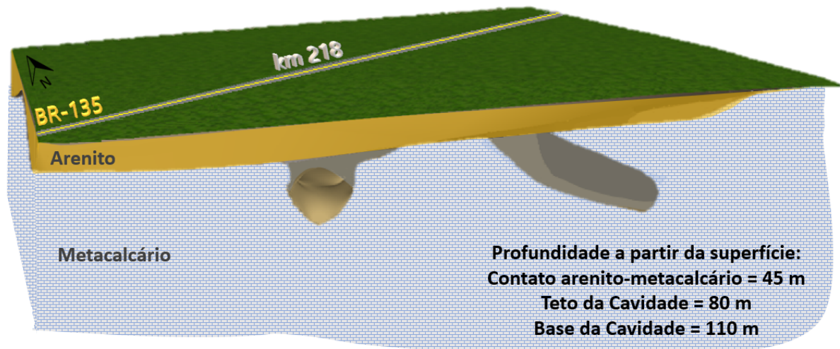
FIGURA 4.69 – REPRESENTAÇÃO TRIDIMENSIONAL DA INTERSEÇÃO ENTRE A BR-135/BA E A CAVERNA BÚRACO DO INFERNO DA LAGOA DO CEMITÉRIO
