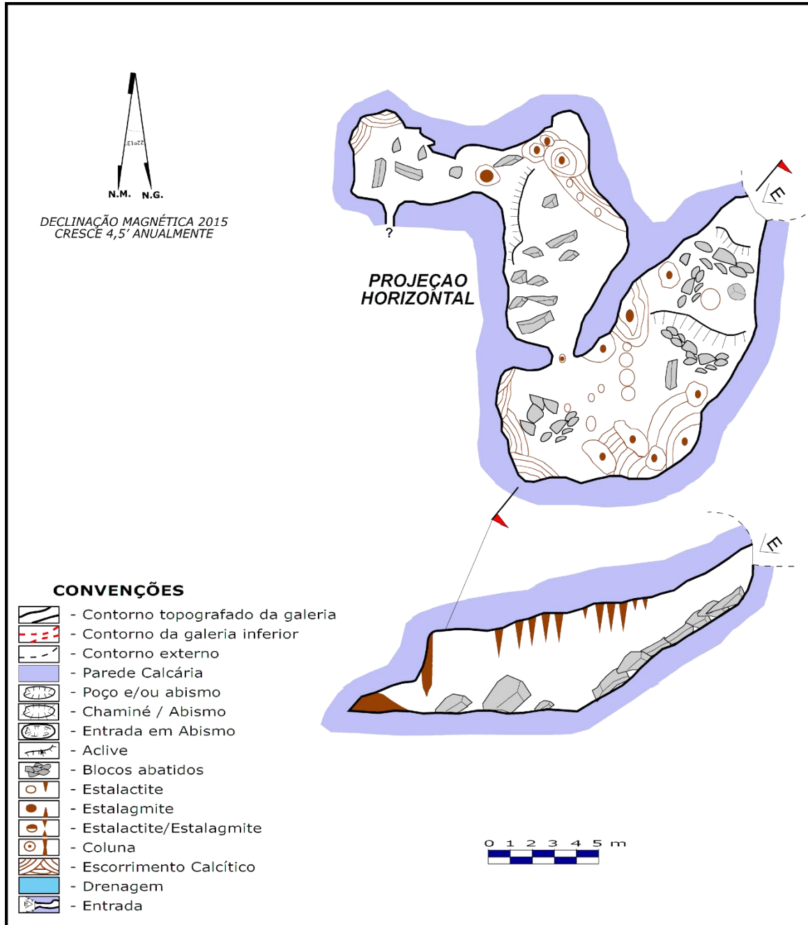
FIGURA 3.34 – MAPA TOPOGRÁFICO DA GRUTA DO JORJÃO
