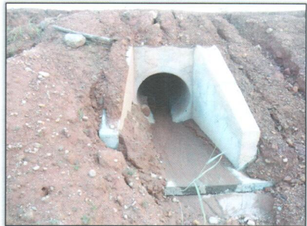
Foto 2 – Desobstrução do bueiro. Estaca: 3056 + 7. S 03.39677° W 052.73244° 13/02/2013
