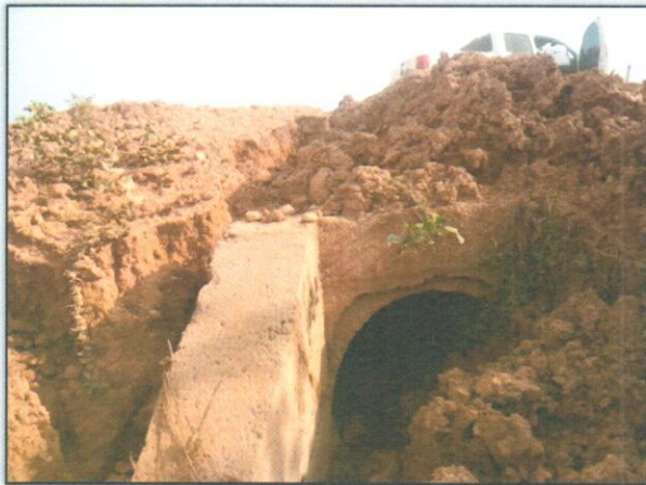
Foto 1 – Obstrução de material excedente na boca do bueiro. Lado: Direito. Estaca: 3048. S 03.39630° W 052.73100° 17/10/2012
