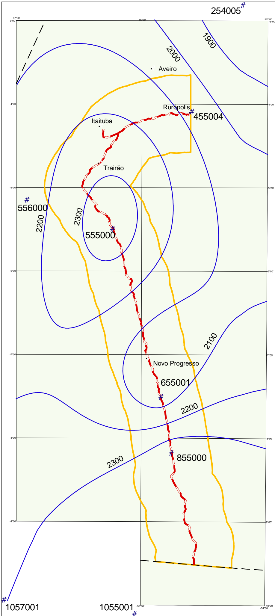
Fig. 2: Isoietas de precipitação média anual
