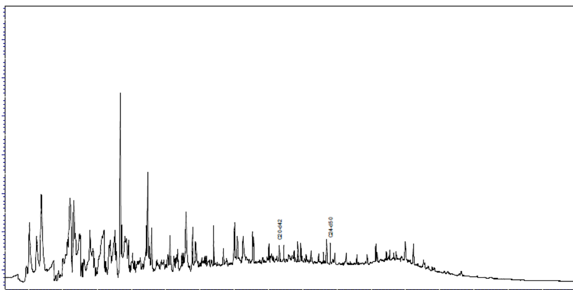
Figura 3.2.2 – Perfil cromatográfico da amostra de água produzida tratada no FPSO Peregrino e coletada em novembro de 2014.
