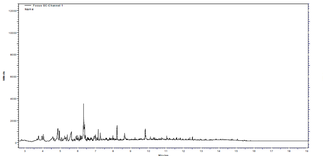
Figura 3.2.1 – Perfil cromatográfico da amostra de água produzida tratada do FPSO Peregrino coletada em maio de 2014.
