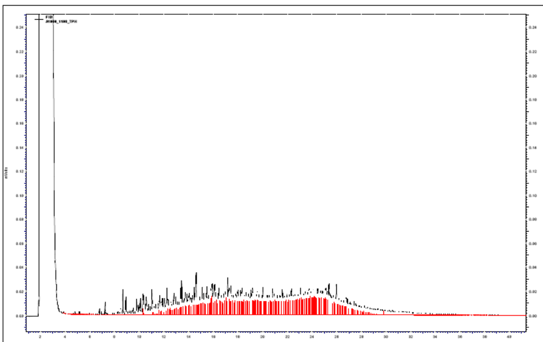
FIGURA 2: Cromatograma da análise de TPH da amostra de água produzida P 50
