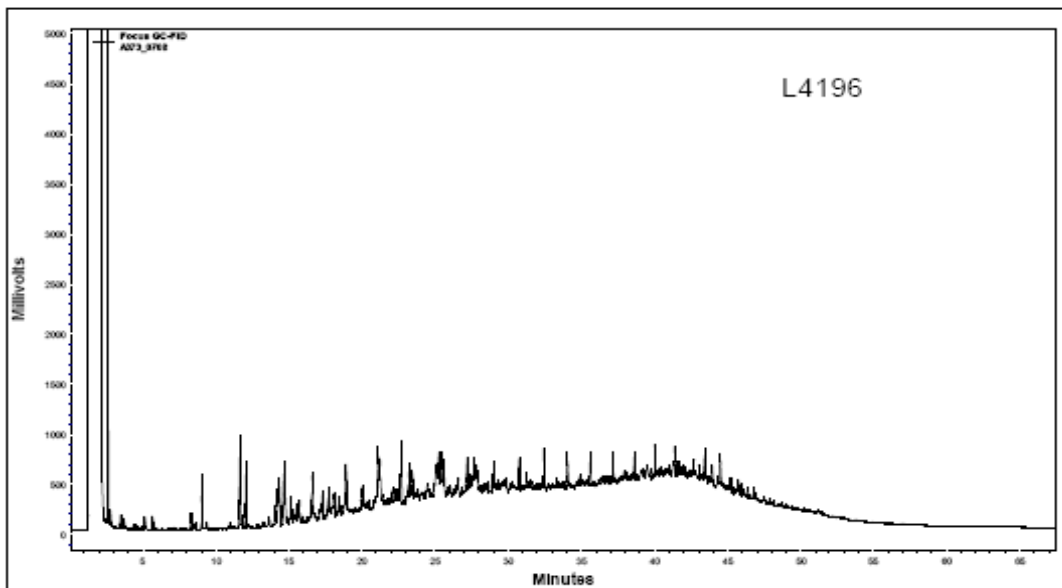
FIGURA 1: Cromatograma da análise de TPH da amostra de água produzida P 50
