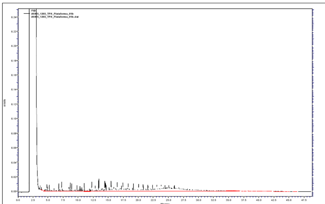
FIGURA 2: Cromatograma da análise de TPH da amostra de água produzida P 48
