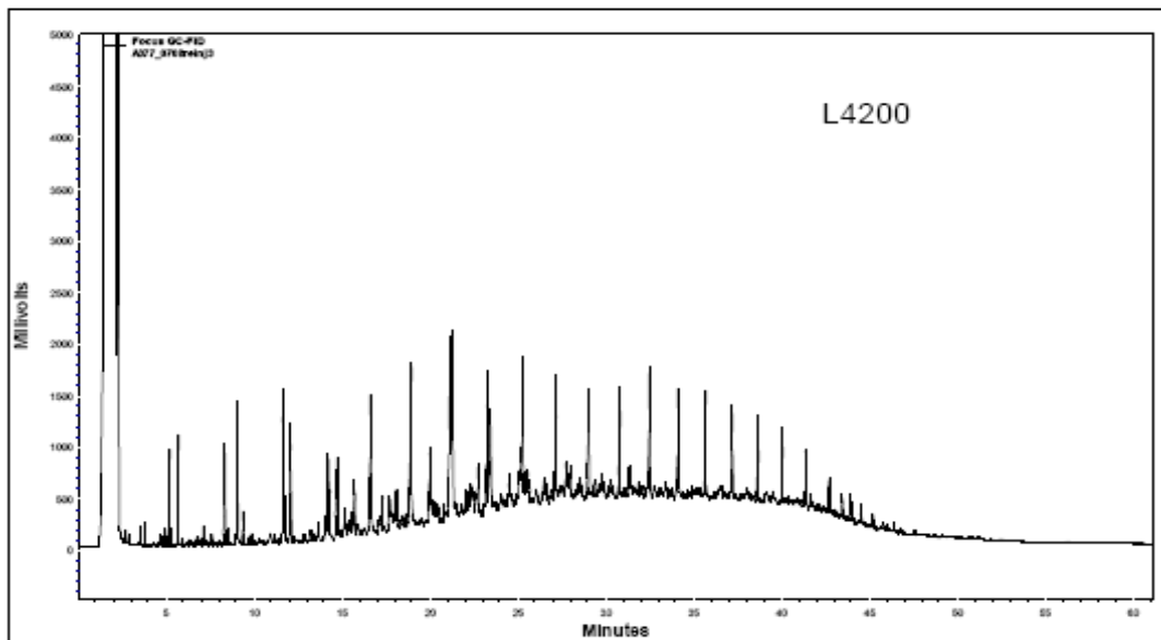
FIGURA 1: Cromatograma da análise de TPH da amostra de água produzida P 48
