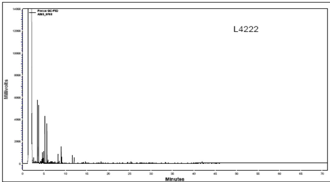
FIGURA 1: Cromatograma da análise de TPH da amostra de água produzida P40
