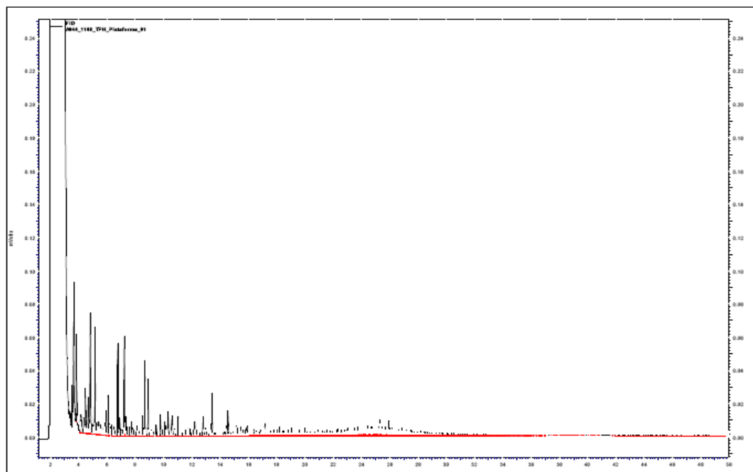
FIGURA 2: Cromatograma da análise de TPH da amostra de água produzida P 40
