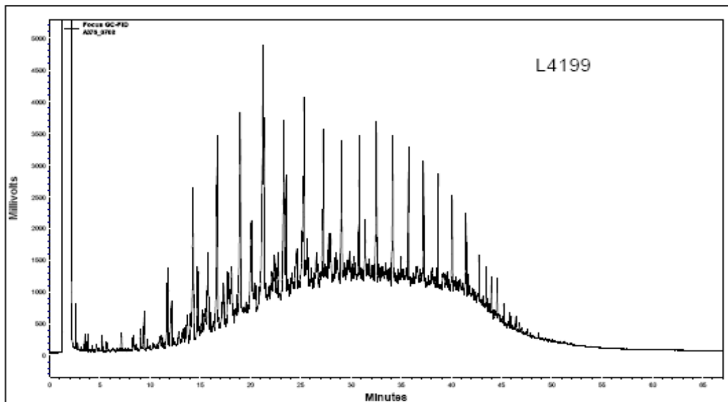
FIGURA 1: Cromatograma da análise de TPH da amostra de água produzida FPBR
