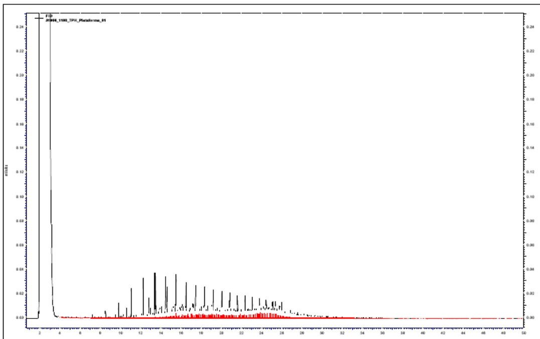
FIGURA 2: Cromatograma da análise de TPH da amostra de água produzida FPBR
