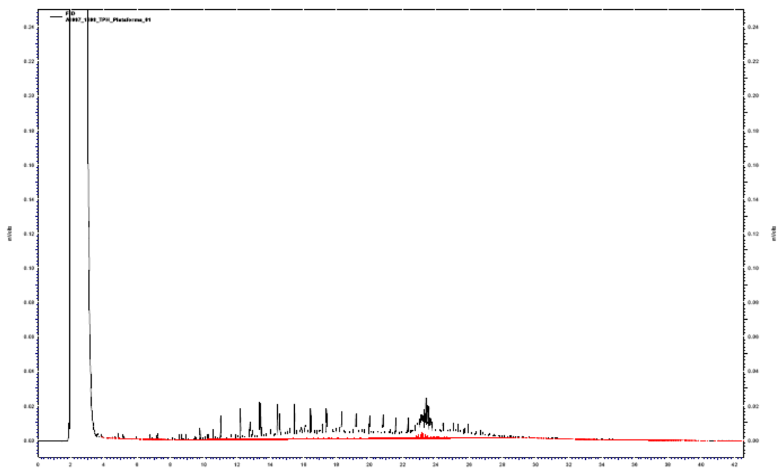
FIGURA 2: Cromatograma da análise de TPH da amostra de água produzida de SS 06
