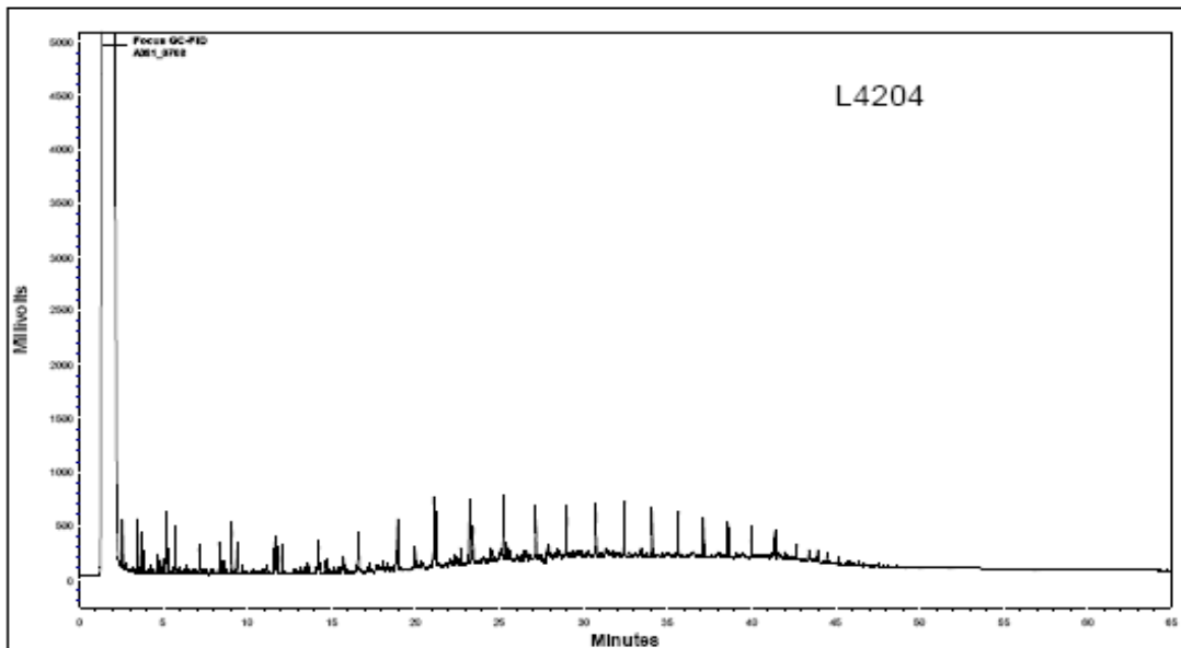
FIGURA 1: Cromatograma da análise de TPH da amostra de água produzida de SS 06
