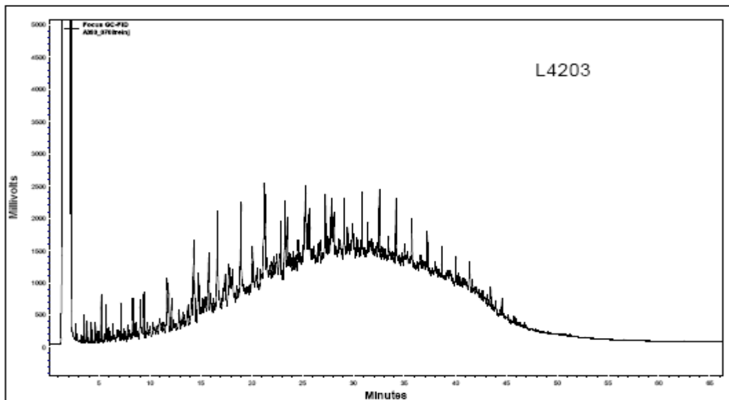
FIGURA 1: Cromatograma da análise de TPH da amostra de água produzida PPM 1 FLOTADOR
