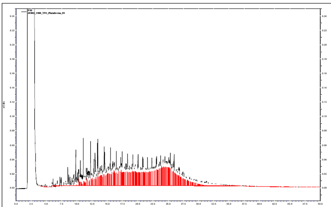
FIGURA 2: Cromatograma da análise de TPH da amostra de água produzida PPM 1 FLOTADOR
