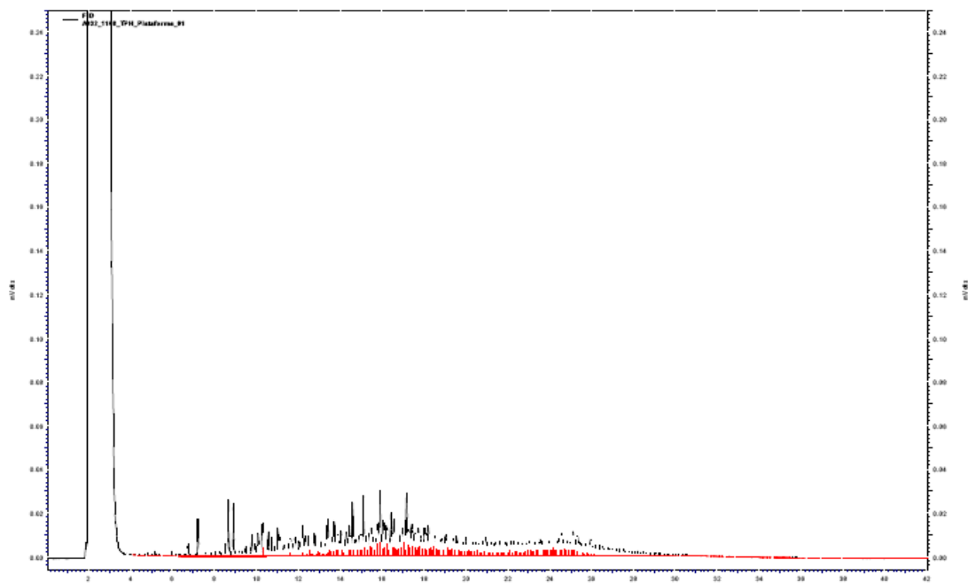
FIGURA 2: Cromatograma da análise de TPH da amostra de água produzida FPRO
