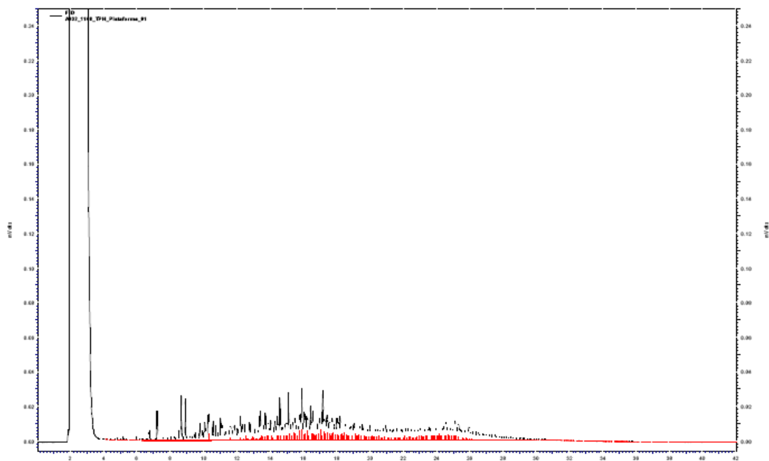
FIGURA 2: Cromatograma da análise de TPH da amostra de água produzida PPG 1
