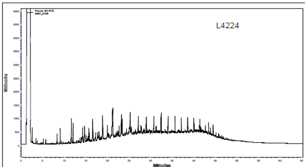
FIGURA 1: Cromatograma da análise de TPH da amostra de água produzida P 27
