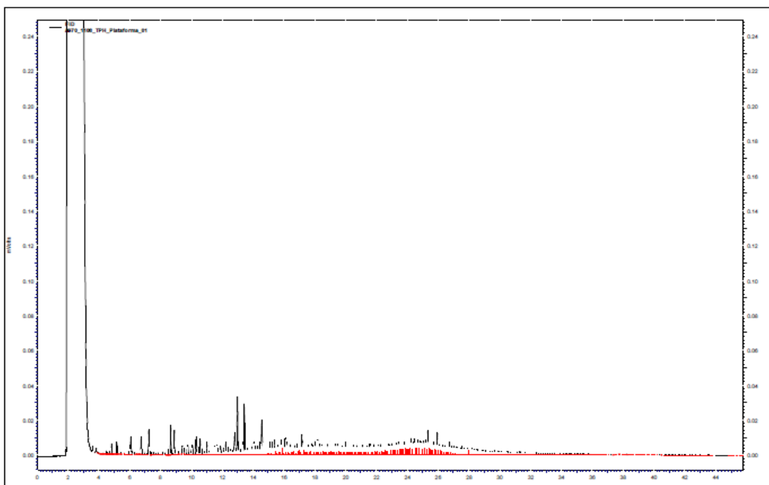
FIGURA 2: Cromatograma da análise de TPH da amostra de água produzida P19
