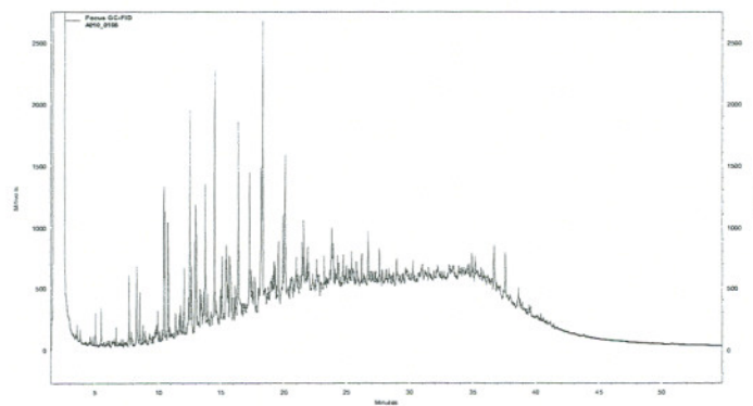
Cromatograma da análise de TPH da amostra de água produzida - Plataforma P-37
