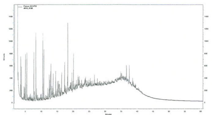
Cromatograma da análise de TPH da amostra de água produzida - Plataforma P-35
