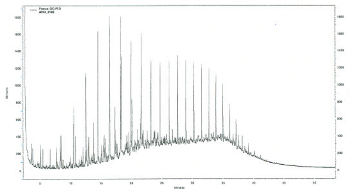
Cromatograma da análise de TPH da amostra de água produzida - Plataforma P-31
