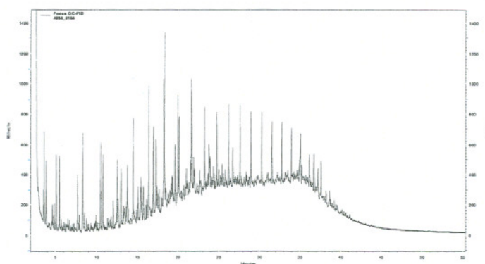
Cromatograma da análise de TPH da amostra de água produzida - Plataforma P-27
