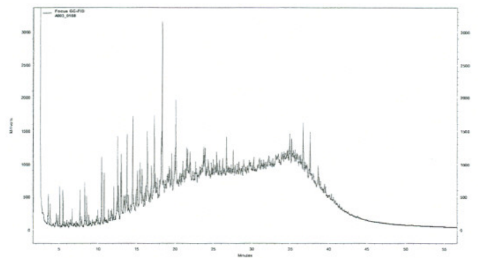
Cromatograma da análise de TPH da amostra de água produzida - Plataforma P-26
