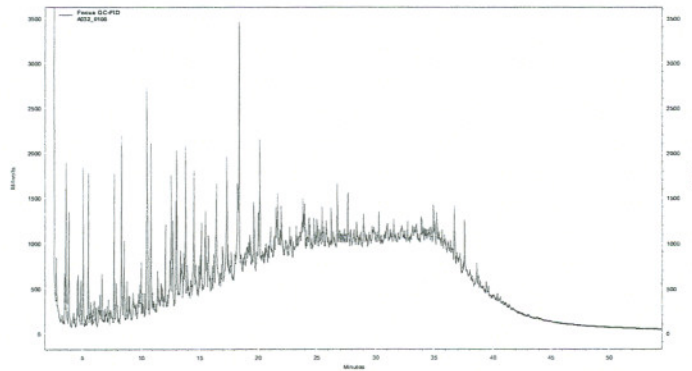
Cromatograma da análise de TPH da amostra de água produzida - Plataforma P18
