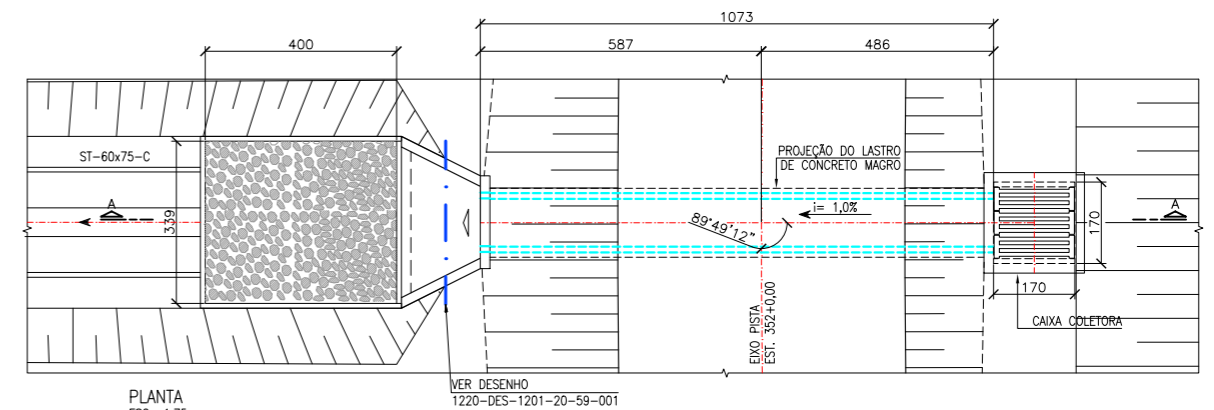
PLANTA ESC.: 1:75
