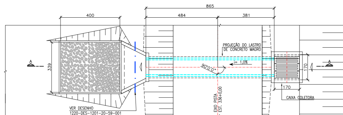
PLANTA ESC.: 1:75
