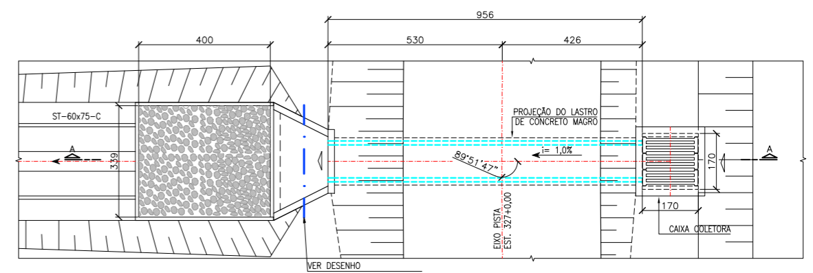
PLANTA ESC.: 1:75
