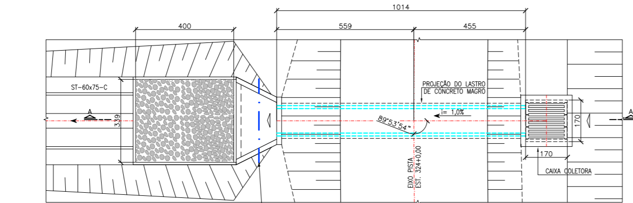
PLANTA ESC.: 1:75
