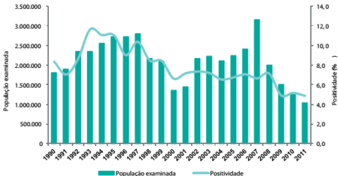
Figura 2.3 – População examinada e percentual de positividade nos inquéritos coproscópicos para esquistossomose - Brasil, de 1990 a 2011.
