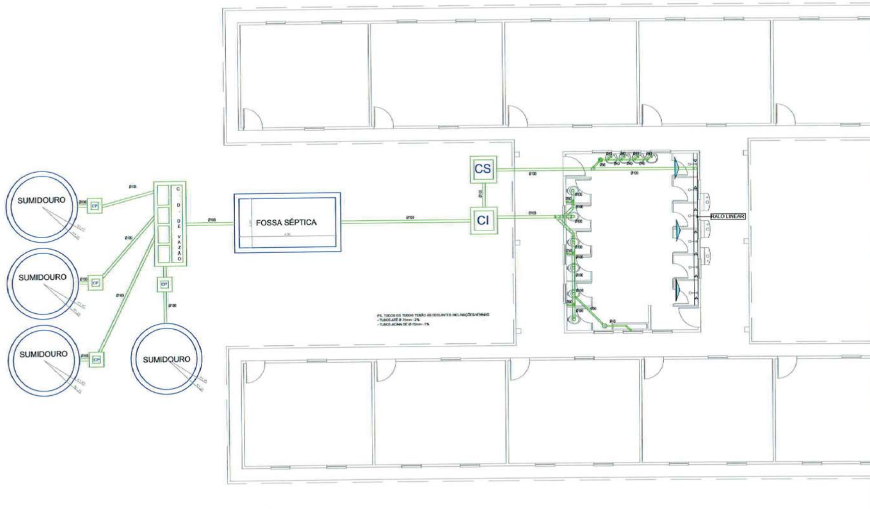
1 PLANTA PAV. TÉRREO ESCALA 1:100
