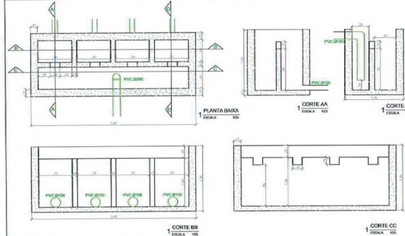
1 CORTE BB ESCALA 1/25
