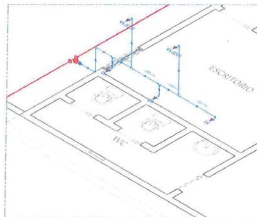
7 ISOMÉTRICO - DETALHE 13 ESCALA 1:25
