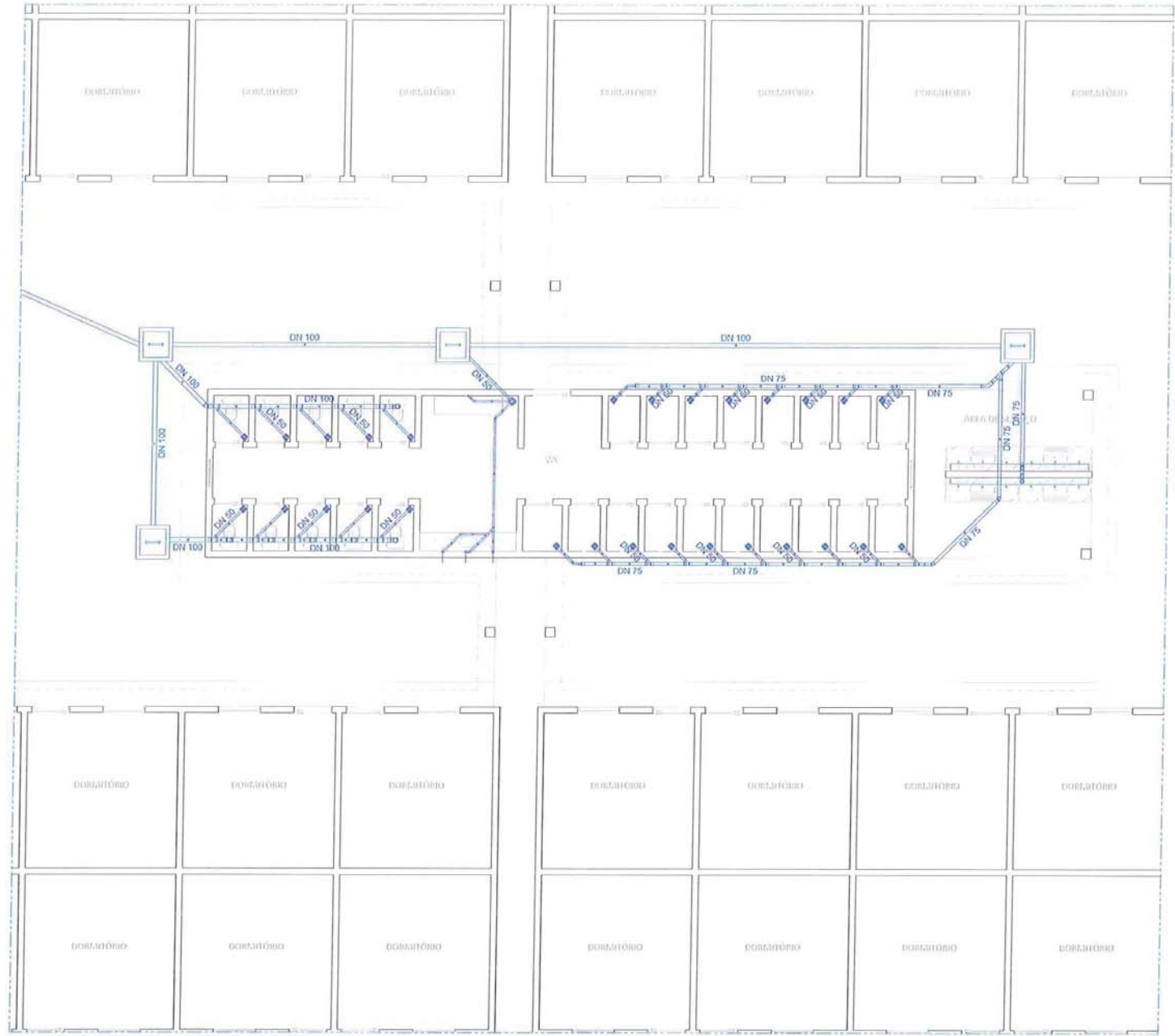
9 PLANTA BAIXA ESGOTO - WC ALOJAMENTO ESCALA 1:50
