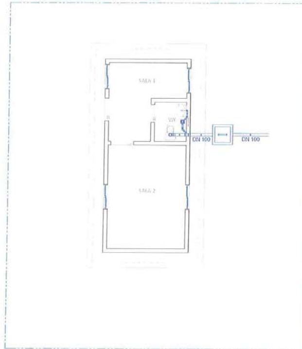
5 PLANTA BAIXA ESGOTO - GUARITA ESCALA 1/50
