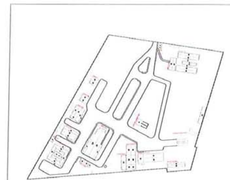
5 PLANTA DE LOCALIZAÇÃO ESCALA 1/200
