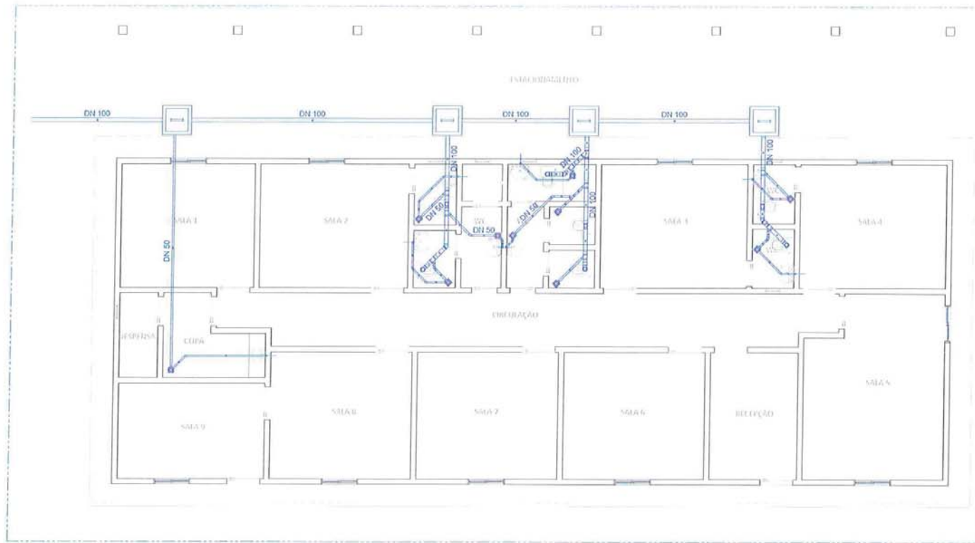
3 PLANTA BAIXA ESGOTO - FISCALIZAÇÃO ESCALA 1/30
