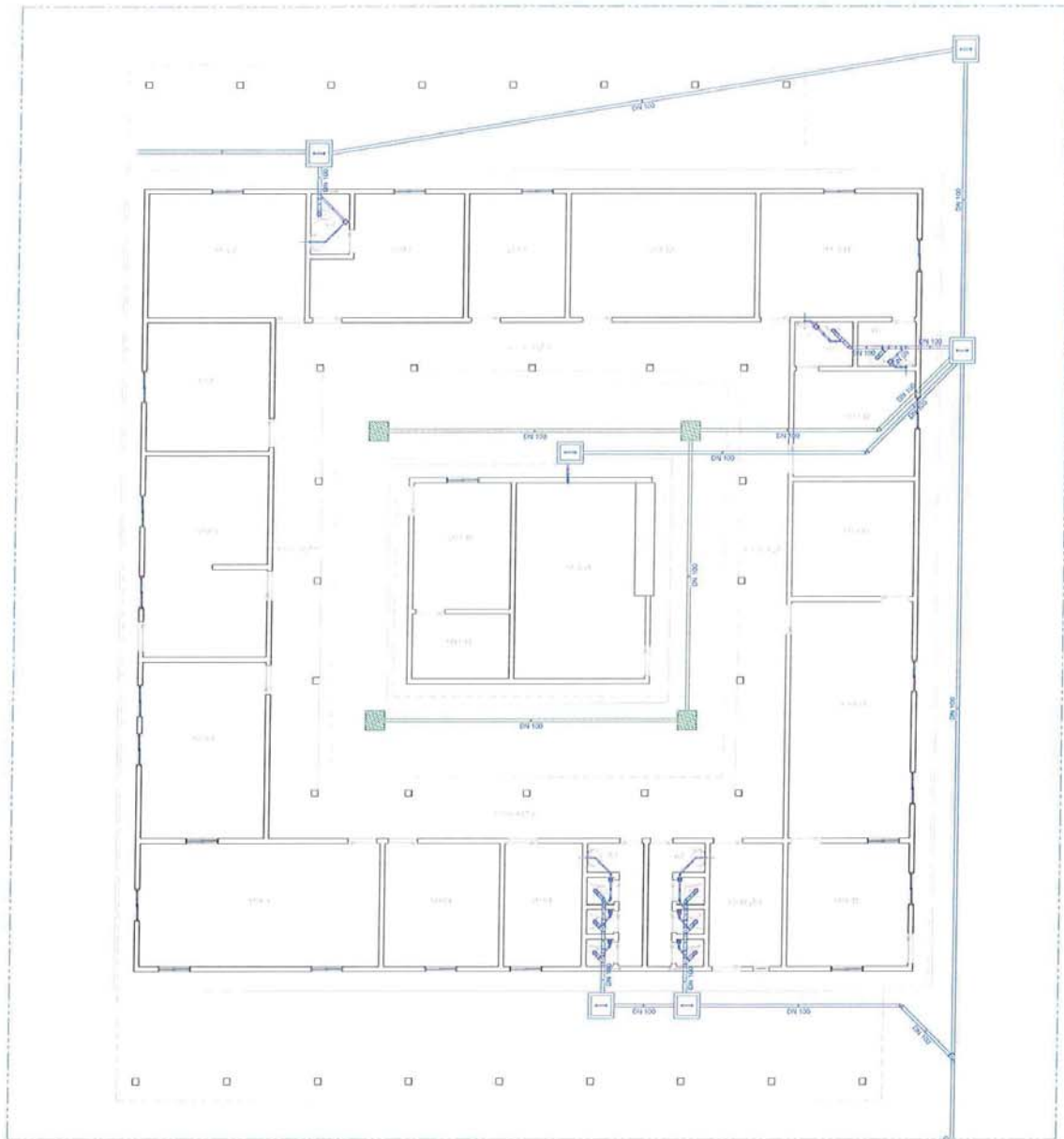
6 PLANTA BAIXA ESGOTO - ADMINISTRAÇÃO ESCALA 1/25
