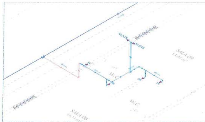
4 ISOMÉTRICO - DETALHE 09 ESCALA 1:25
