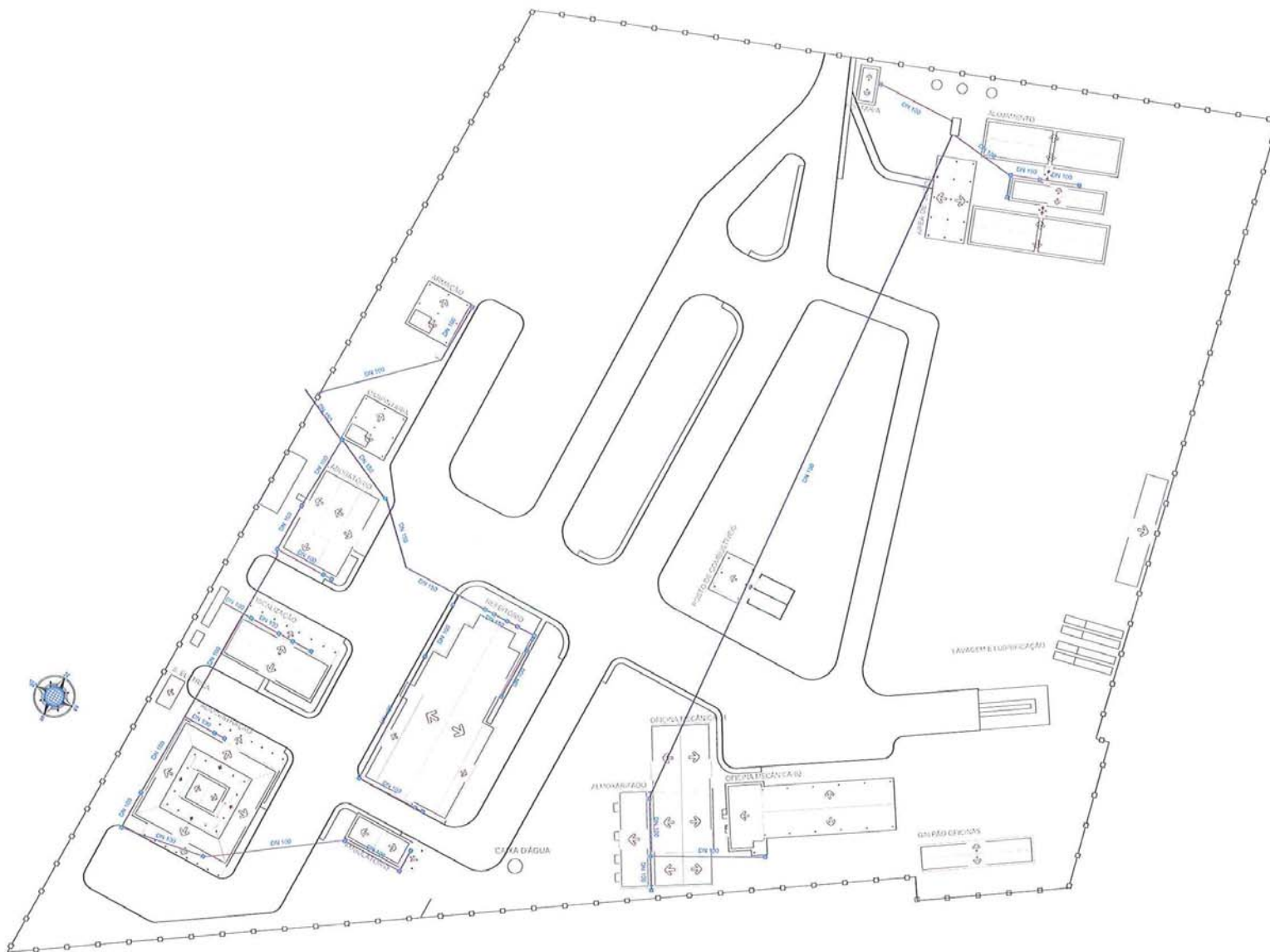
1 PLANTA DE SITUAÇÃO ESGOTO - CANTEIRO LOTE 06 ESCALA 1:500
