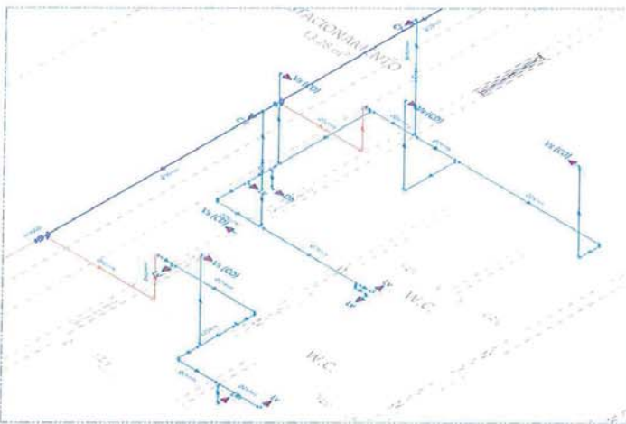
4 ISOMÉTRICO - DETALHE 08 ESCALA 1:25
