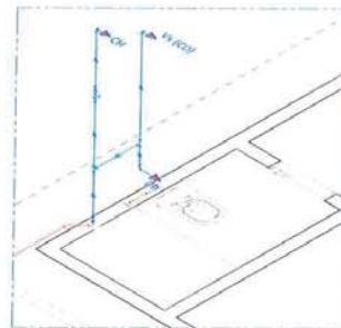
3 ISOMÉTRICO - DETALHE 03 ESCALA 1:10
