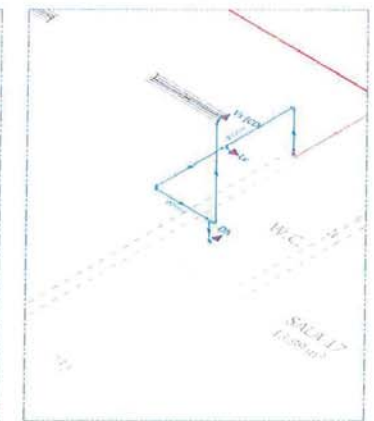
3 ISOMÉTRICO - DETALHE 06 ESCALA 1:25
