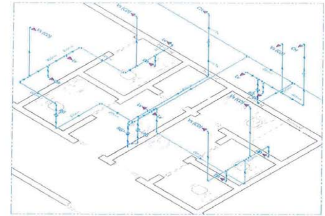
3 ISOMÉTRICO - DETALHE 04 ESCALA 1:10
