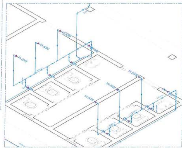
6 ISOMÉTRICO - DETALHE 10 ESCALA 1:20
