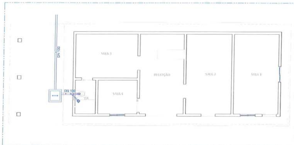
3 PLANTA BAIXA ESGOTO - AMBULATÓRIO ESCALA 1/30
