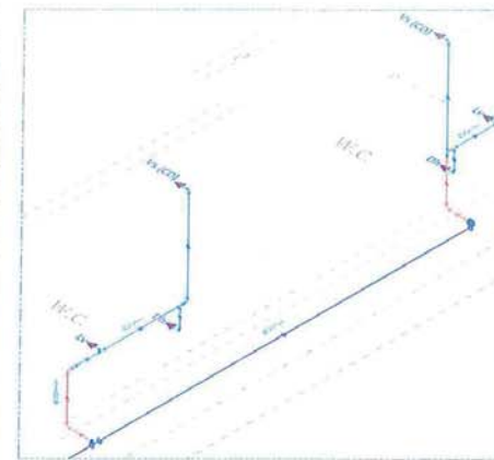
3 ISOMÉTRICO - DETALHE 05 ESCALA 1:25
