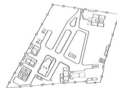
1 PLANTA DE LOCALIZAÇÃO ESCALA 1:2000
