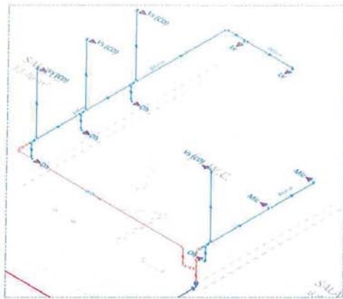
3 ISOMÉTRICO - DETALHE 03 ESCALA 1:25
