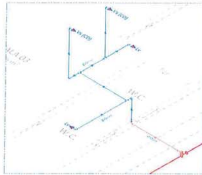
5 ISOMÉTRICO - DETALHE 11 ESCALA 1:25
