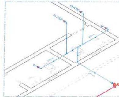
8 ISOMÉTRICO - DETALHE 15 ESCALA 1:25
