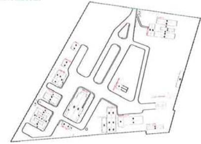
2 PLANTA DE LOCALIZAÇÃO ESCALA 1/200
