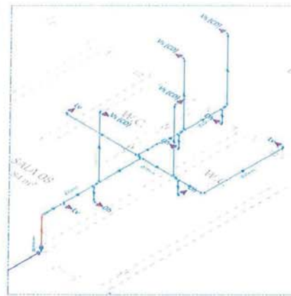
3 ISOMÉTRICO - DETALHE 04 ESCALA 1:25
