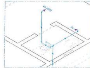
5 ISOMÉTRICO - DETALHE 09 ESCALA 1:25
