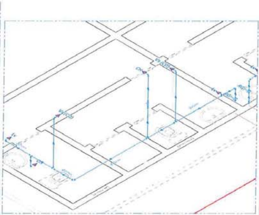
2 ISOMÉTRICO - DETALHE 02 ESCALA 1:25
