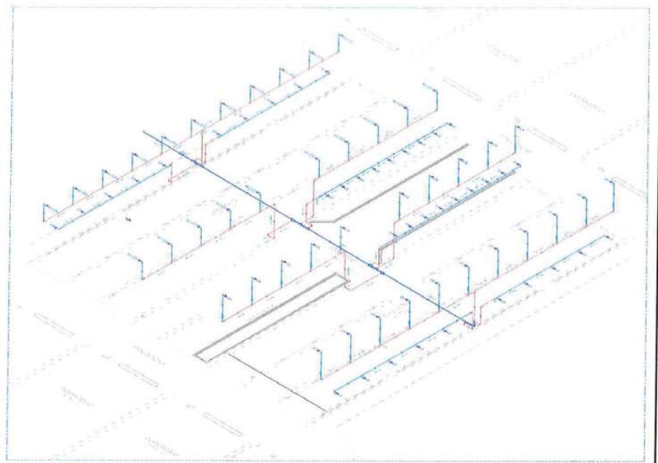
2 ISOMÉTRICO DETALHE 01 - WCS ALOJAMENTO ESCALA 1:50
