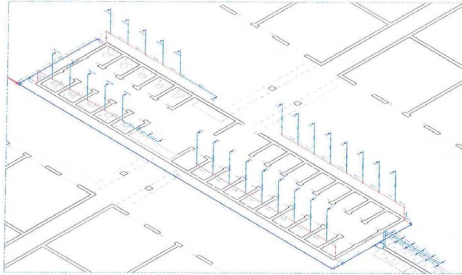
9 ISOMÉTRICO - DETALHE 16 ESCALA 1:25
