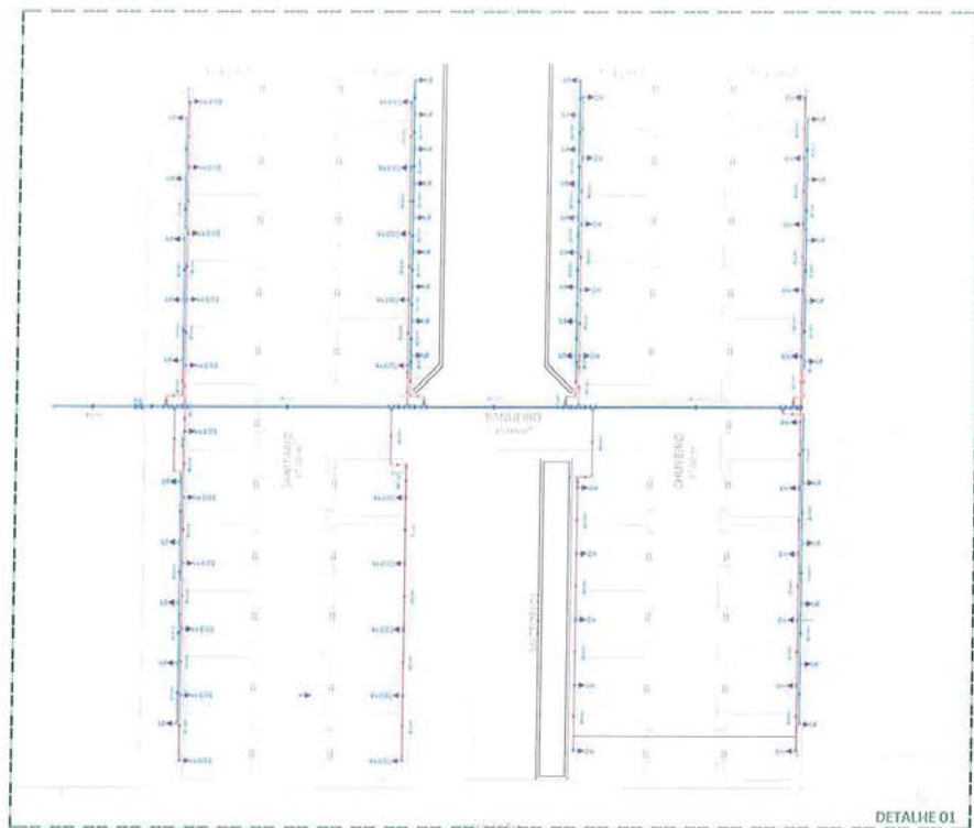
2 PLANTA BAIXA ÁGUA FRIA - WCS ALOJAMENTO ESCALA 1:50
