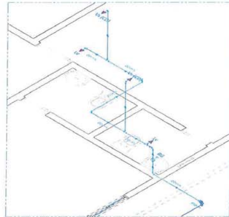
6 ISOMÉTRICO - DETALHE 11 ESCALA 1:20
