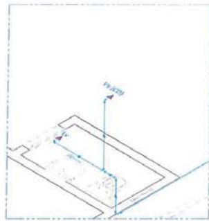
5 ISOMÉTRICO - DETALHE 08 ESCALA 1:25
