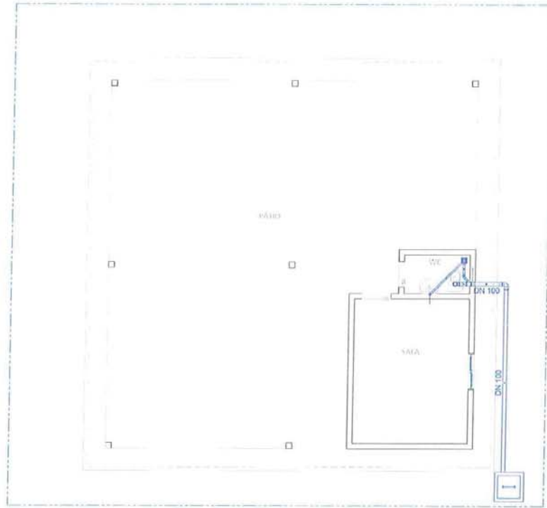
5 PLANTA BAIXA ESGOTO - CARPINTARIA/ARMAÇÃO ESCALA 1/50
