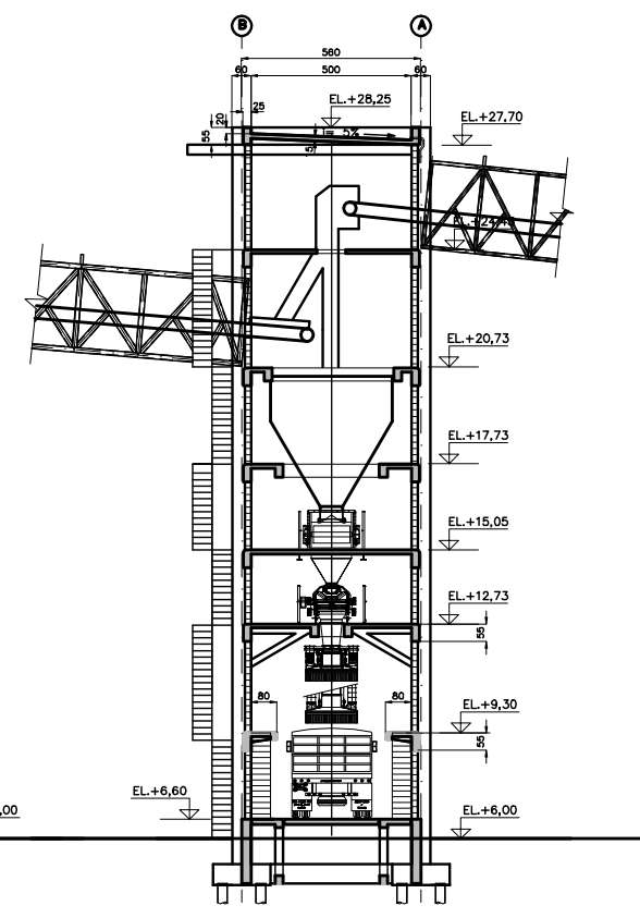
CORTE E-E (TRANSVERSAL - TULHA RODOMÁRIA) ESC. 1:100
