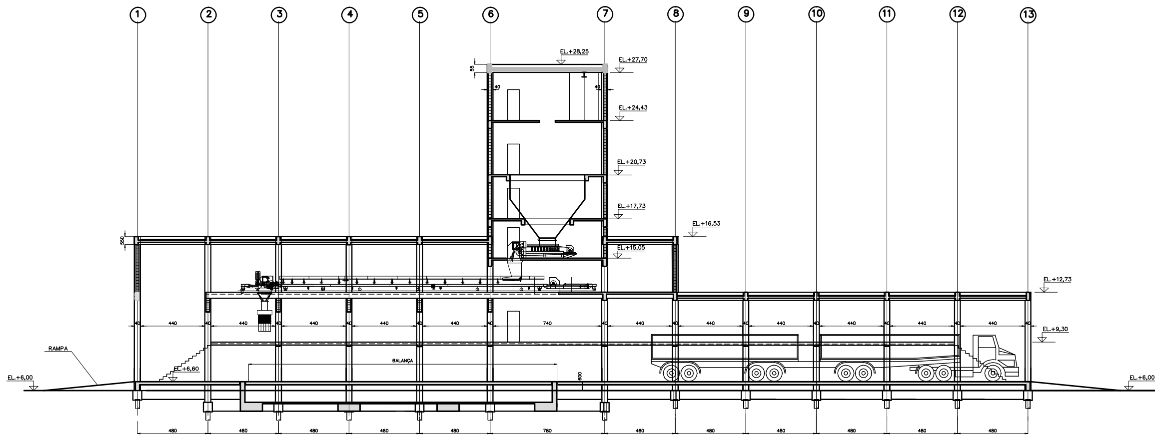
CORTE F-F (LONGITUDINAL - TULHA RODOMÁRIA) ESC. 1:100
